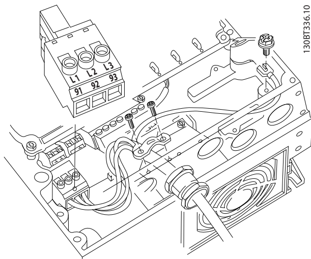
Bild 8.2 Nät och jordning utan fränksiljare
