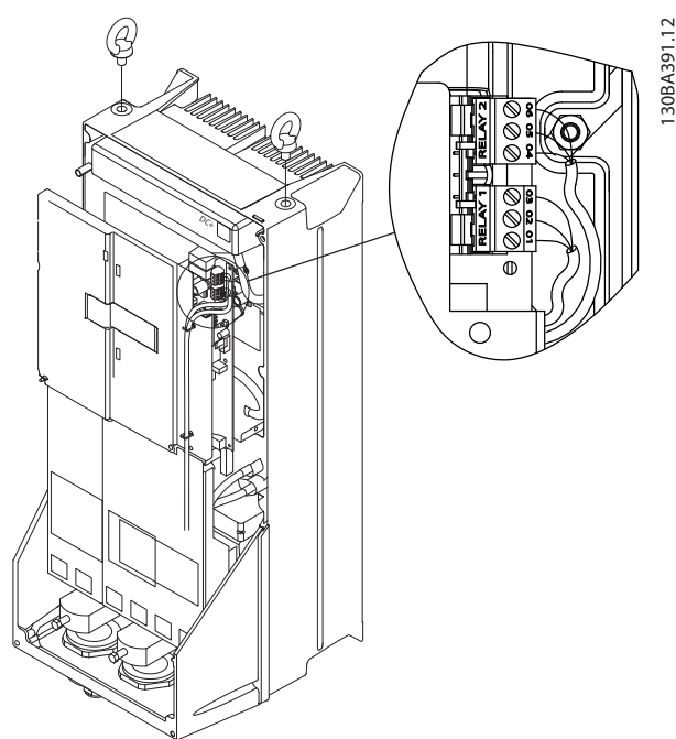
Bild 8.19 Plintar för reläanslutning (kapslingsstorlek C1 och C2).
