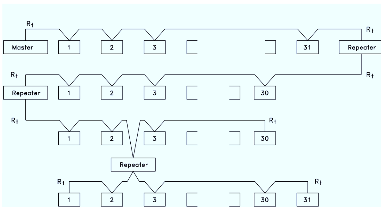
Bild 3.40 RS485-bussgränssnitt
