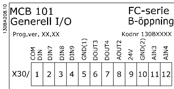
Bild 7.2 Tillvalet MCB 101
