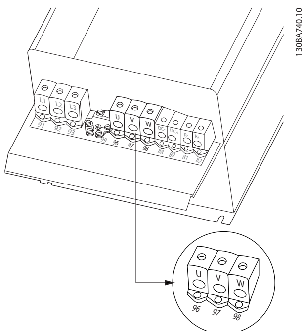
Bild 8.17 Motoranslutning för kapsling C3 och C4
