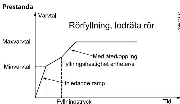
Bild 4.8 Rörfyllningsläge, prestandakurva
