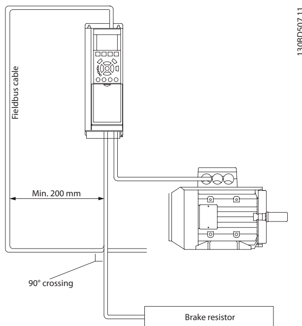
Bild 3.43 Kabeldragning
