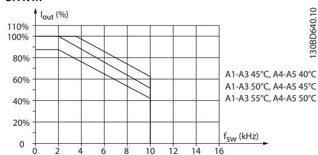
Bild 5.6 Nedstämpling av I_{out} för olika T_{AMB, MAX} för kapslingstyp A, med SFAVM och maximalt 10 m motorkabel
