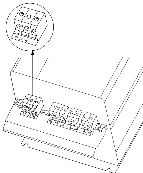
Bild 8.8 Nätanslutning kapsling C3 (IP20).
