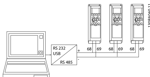
Bild 3.41 Parallellkopplingar
