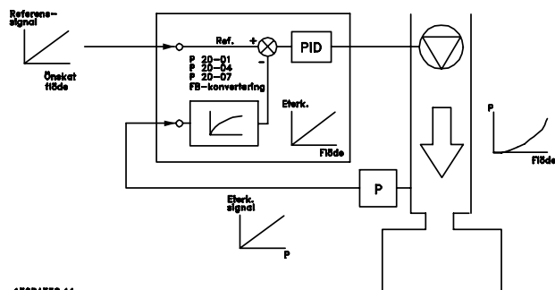
Bild 2.17 Återkopplingskonvertering
