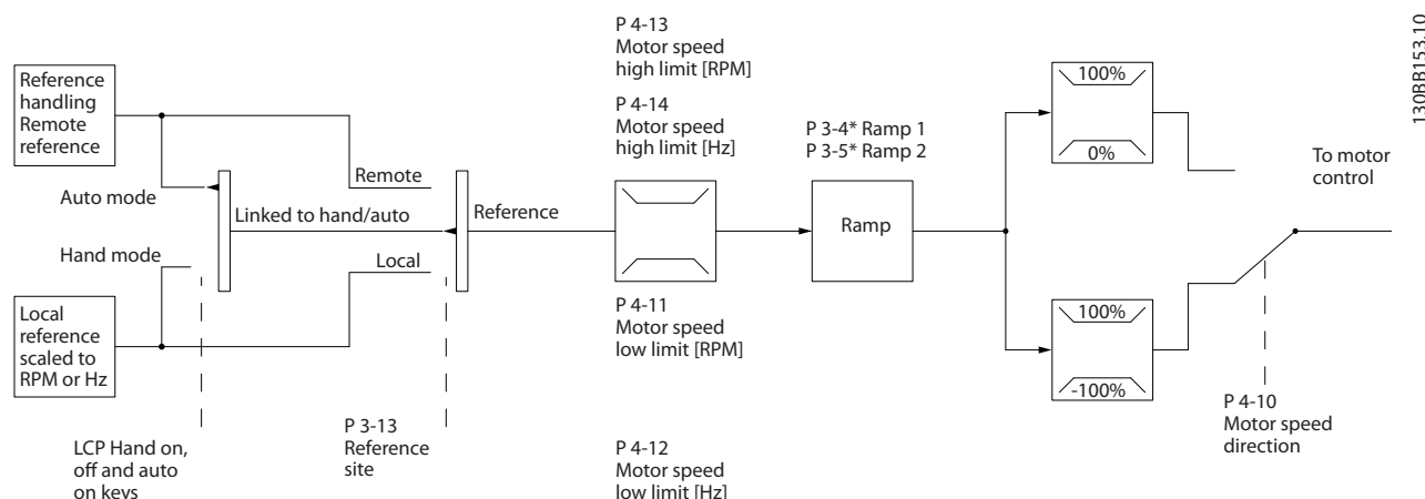
Bild 2.11 Blockdiagram över läge utan återkoppling
