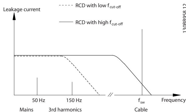
Bild 3.8 Huvudsakliga bidragande faktorer till läckström
