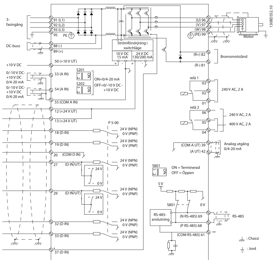
Bild 3.20 Grundläggande kopplingsschema
