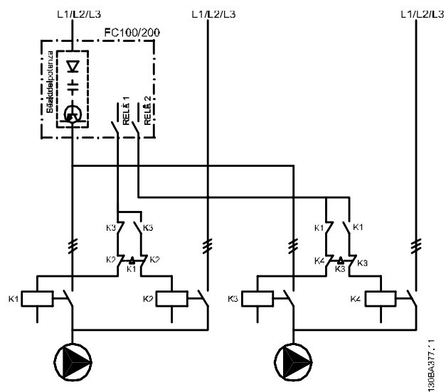
Bild 4.13 Kopplingsschema för huvudpumpsväxling
