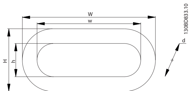
Bild 6.4 HF-CM-kärna
