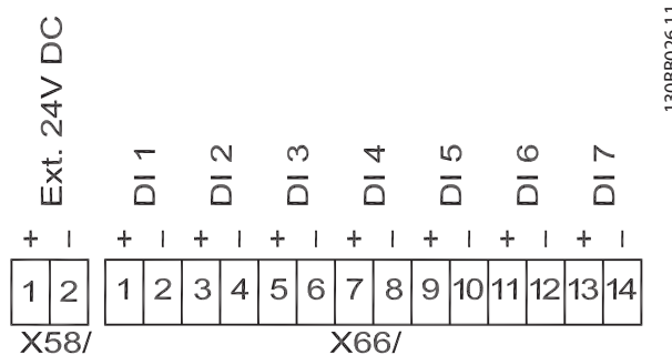
Bild 7.20 Avancerad kaskadregulator MCO 102, plintanslutningar till 7 digitala ingångar och åtkomst till intern 24 V DC
