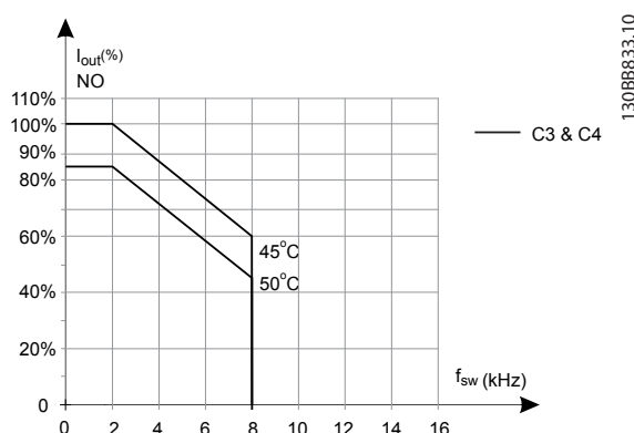
Bild 5.18 Nedstämpling av I_{out} för olika T_{AMB, MAX} för kapslingsstorlek C3 och C4, med SFAVM i läget Normal överbelastning (110 % övermoment)
