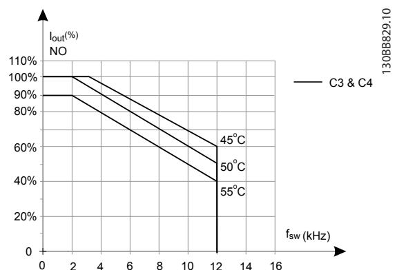
Bild 5.16 Nedstämpling av I_{out} för olika T_{AMB, MAX} för kapslingsstorlek C3 och C4, med 60° AVM i läget Normal överbelastning (110 % övermoment)
