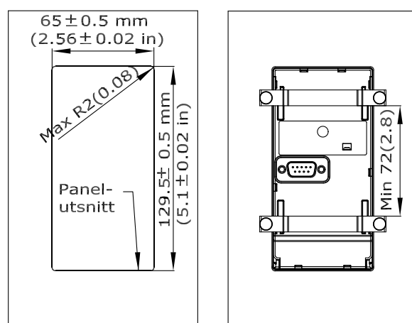
Bild 3.37 LCP-satsens mått
