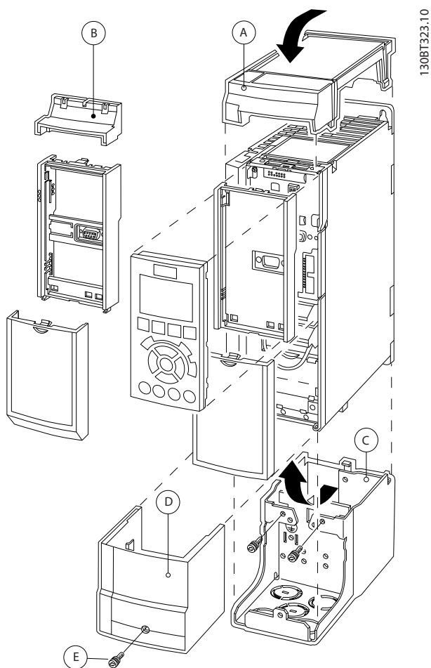
Bild 3.31 Kapslingsstorlek A2
