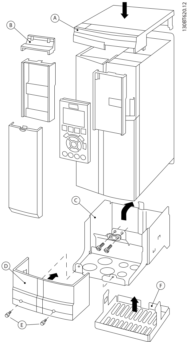
Bild 3.33 Kapslingsstorlek B3
