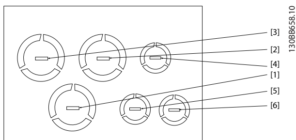
Bild 8.32 Kapslingsstorlek B2, IP55 gängade kabelförskruvningshål
