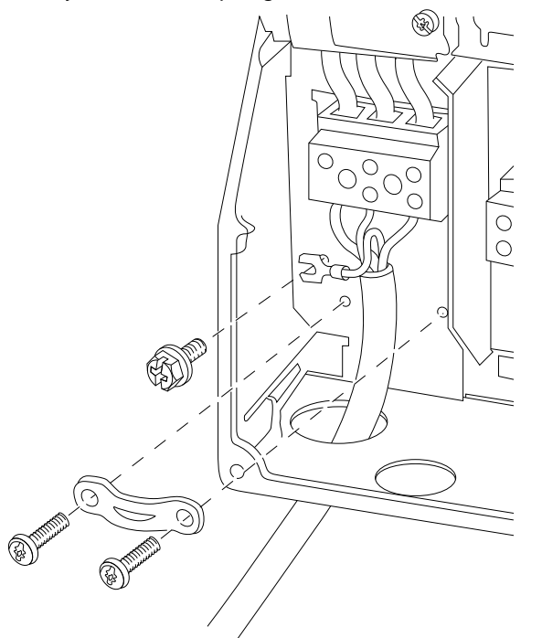
Bild 8.4 Nätanslutning kapsling B1 och B2
