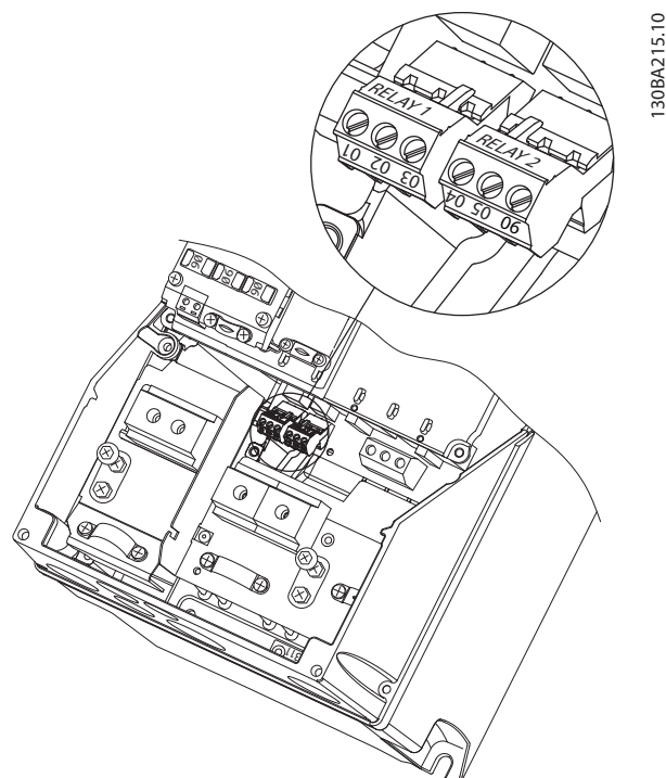
Bild 8.20 Plintar för reläanslutning (kapslingsstorlek A5, B1 och B2).
