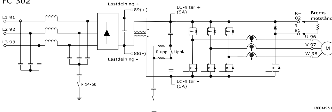
Bild 2.10 Frekvensomformarens struktur
