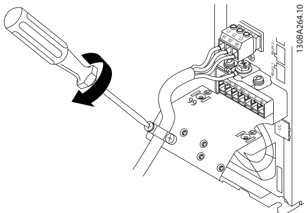
Bild 8.1 Stödfäste
