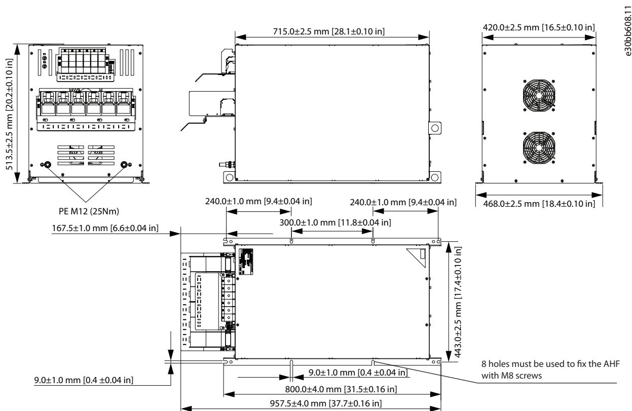
Abbildung 7.30 IP20 X8-V3 Interner Lüfter
