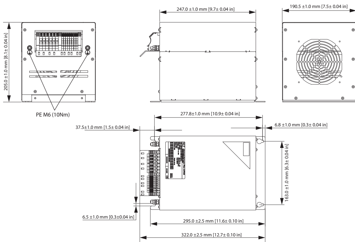
Abbildung 7.2 IP20 X1-V3 Interner Lüfter
