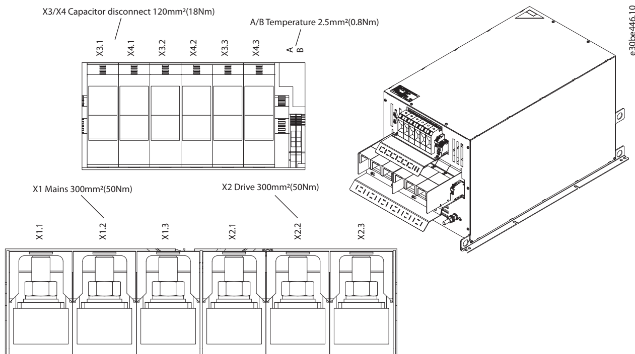
Abbildung 7.29 IP20 X7-V3 Externer Lüfter, Klemmenbezeichnung und 3D-Ansicht
