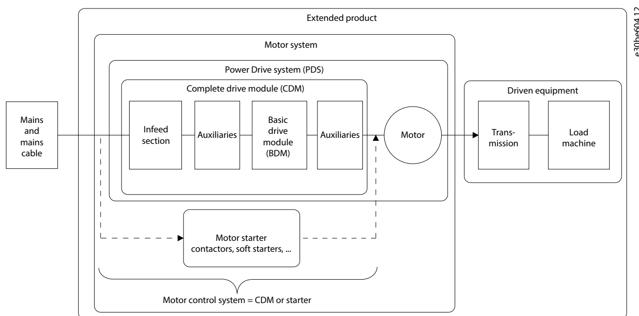
Abbildung 9.1 Antriebssystem und komplettes Antriebsmodul
