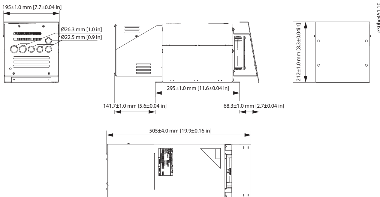
Abbildung 7.34 IP21 X1-V3 interner und externer Lüfter
