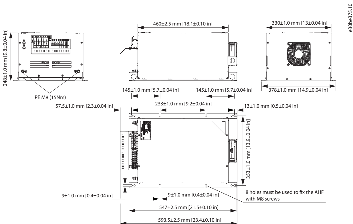
Abbildung 7.12 IP20 X3-V3 Externer Lüfter
