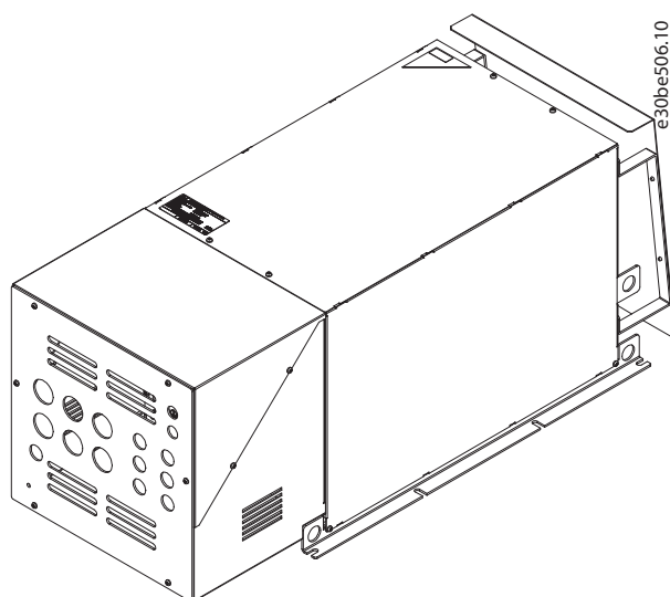
Abbildung 7.45 IP21 X6-V3 interner und externer Lüfter, 3D-Ansicht
