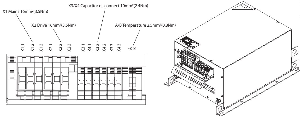
Abbildung 7.11 IP20 X3-V3 Interner Lüfter, Klemmenbezeichnung und 3D-Ansicht
