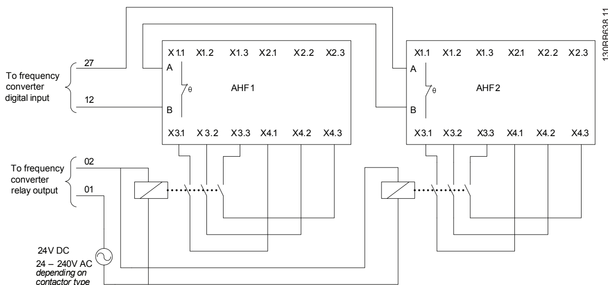
Abbildung 4.9 Parallele Verwendung von AHF mit Kondensatorschalter
