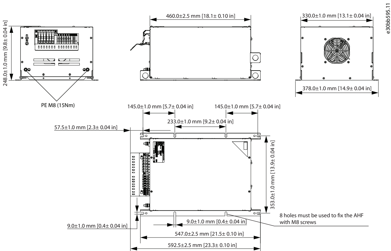
Abbildung 7.10 IP20 X3-V3 Interner Lüfter
