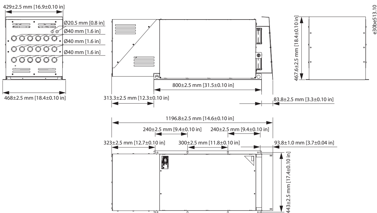
Abbildung 7.46 IP21 X7-V3 interner und externer Lüfter
