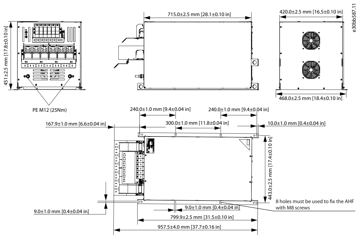
Abbildung 7.26 IP20 X7-V3 Interner Lüfter
