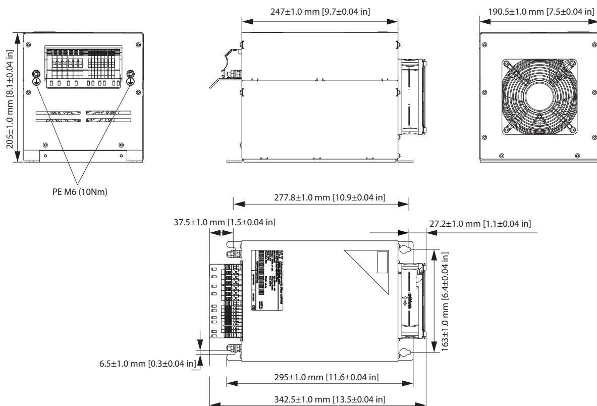
Abbildung 7.4 IP20 X1-V3 Externer Lüfter
