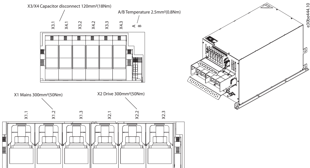
Abbildung 7.27 IP20 X7-V3 Interner Lüfter, Klemmenbezeichnung und 3D-Ansicht
