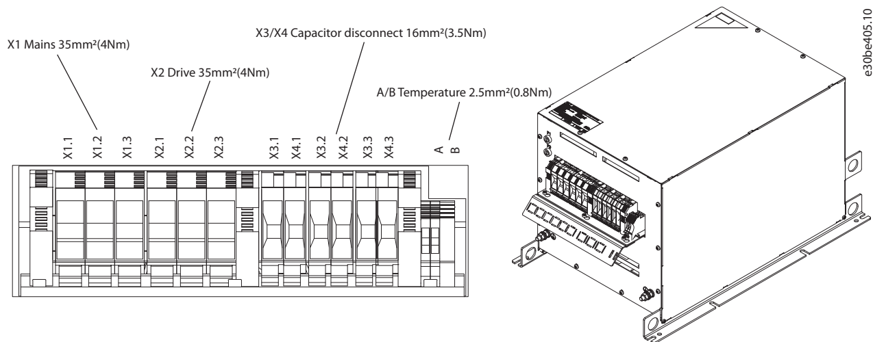
Abbildung 7.17 IP20 X4-V3 Externer Lüfter, Klemmenbezeichnung und 3D-Ansicht
