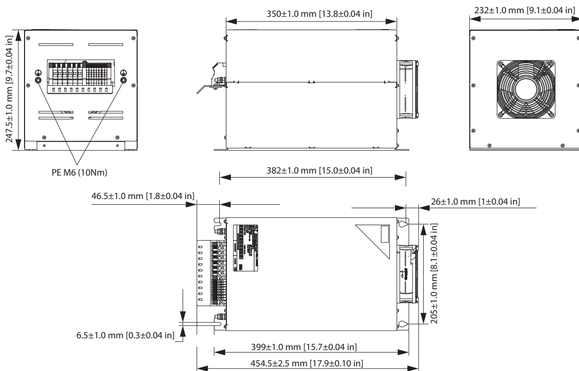
Abbildung 7.8 IP20 X2-V3 Externer Lüfter
