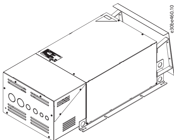
Abbildung 7.39 IP21 X3-V3 interner und externer Lüfter, 3D-Ansicht
