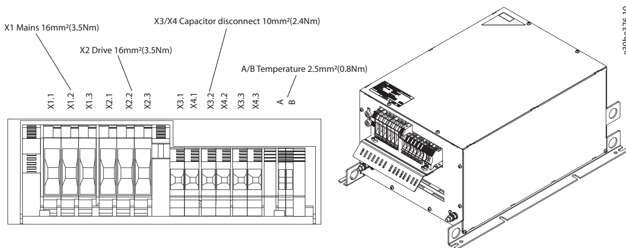
Abbildung 7.13 IP20 X3-V3 Externer Lüfter, Klemmenbezeichnung und 3D-Ansicht
