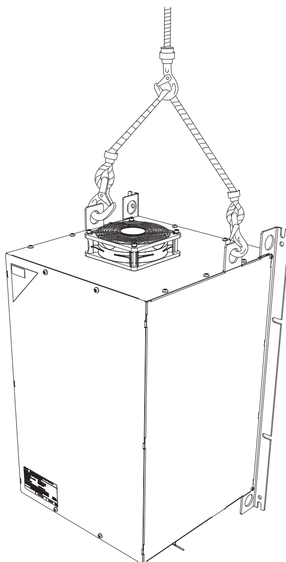
Abbildung 4.2 Empfohlenes Hebeverfahren, Externe Lüfterfilter
