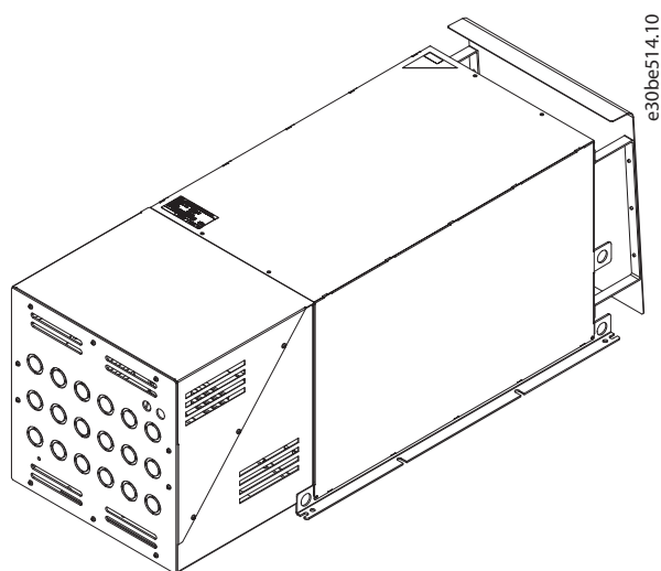
Abbildung 7.47 IP21 X7-V3 interner und externer Lüfter, 3D-Ansicht
