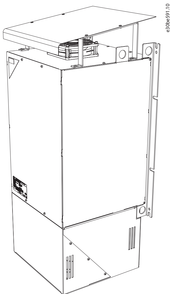
Abbildung 5.1 IP21/NEMA 1-Satz, interner Lüfter und externer Lüfter
