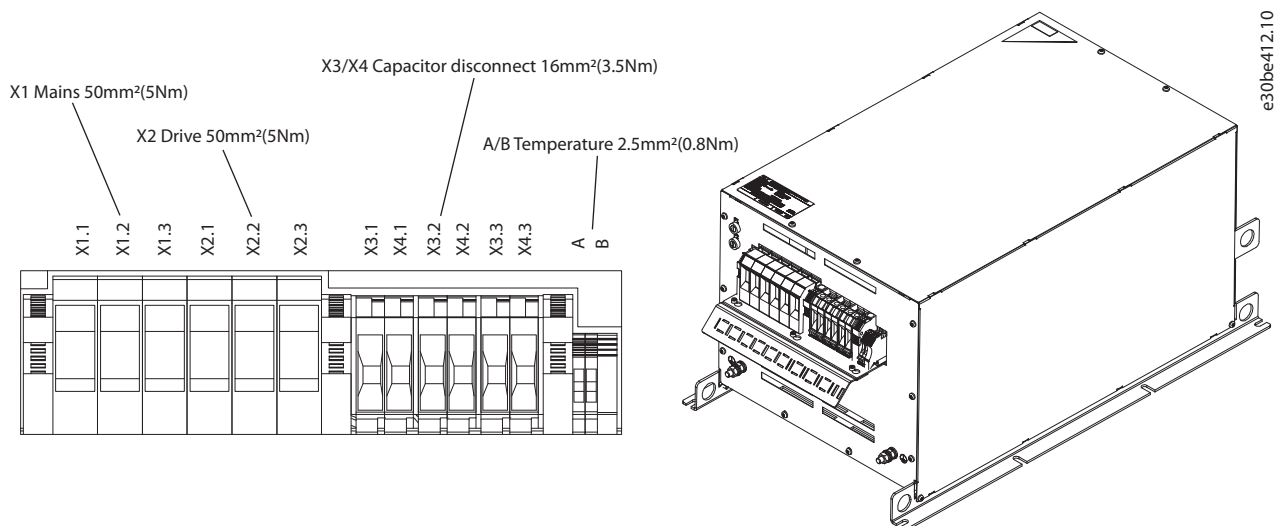
Abbildung 7.21 IP20 X5-V3 Externer Lüfter, Klemmenbezeichnung und 3D-Ansicht
