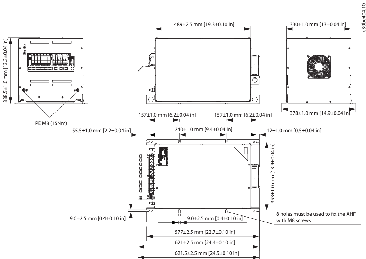
Abbildung 7.16 IP20 X4-V3 Externer Lüfter
