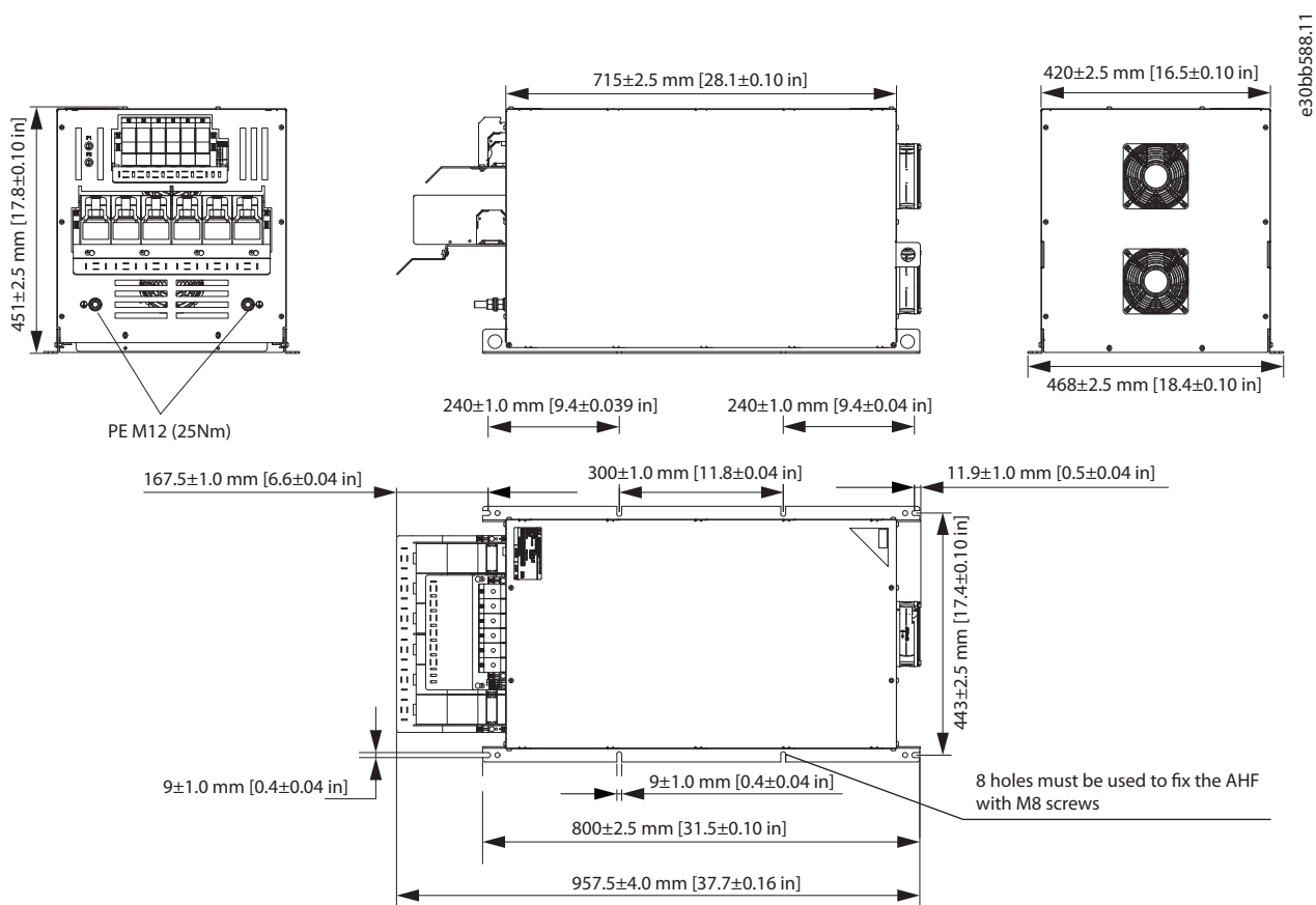
Abbildung 7.28 IP20 X7-V3 Externer Lüfter
