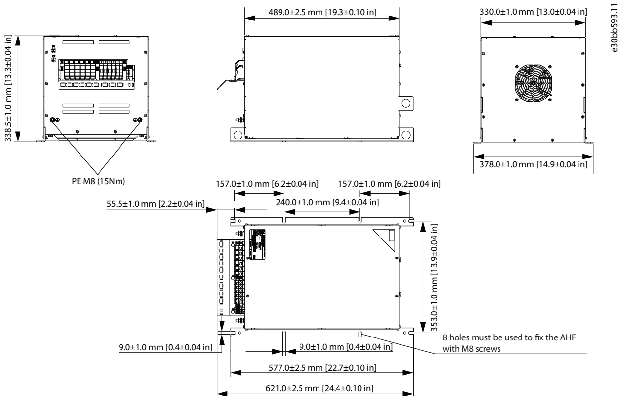
Abbildung 7.14 IP20 X4-V3 Interner Lüfter
