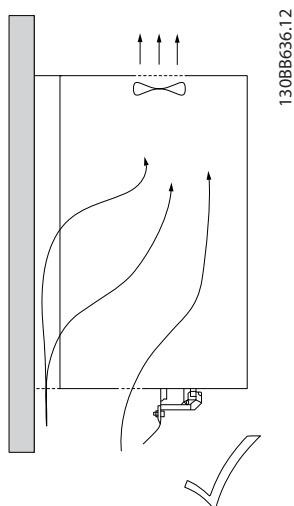
Abbildung 4.3 Einwandfreie Luftzirkulation ohne Rückwand
