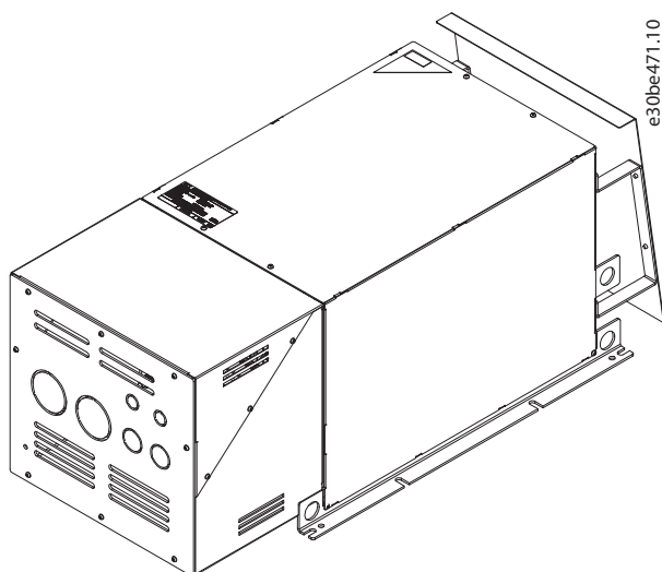
Abbildung 7.41 IP21 X4-V3 interner und externer Lüfter, 3D-Ansicht
