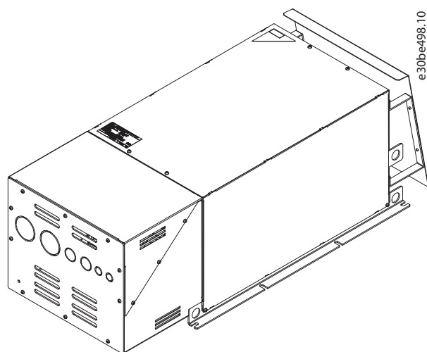
Abbildung 7.43 IP21 X5-V3 interner und externer Lüfter, 3D-Ansicht
