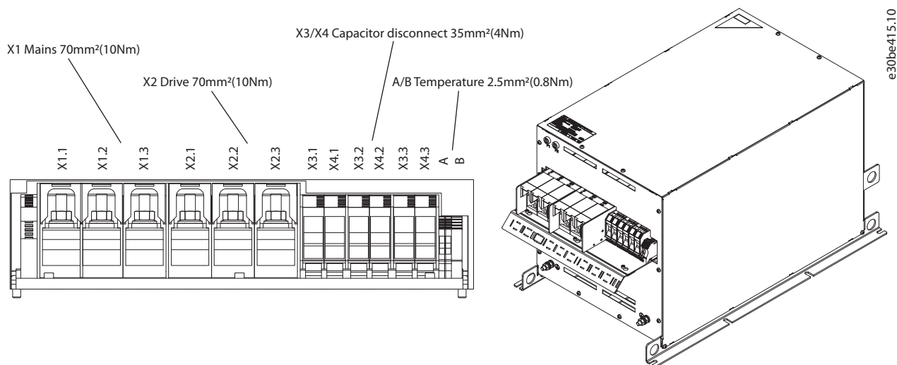
Abbildung 7.23 IP20 X6-V3 Interner Lüfter, Klemmenbezeichnung und 3D-Ansicht
