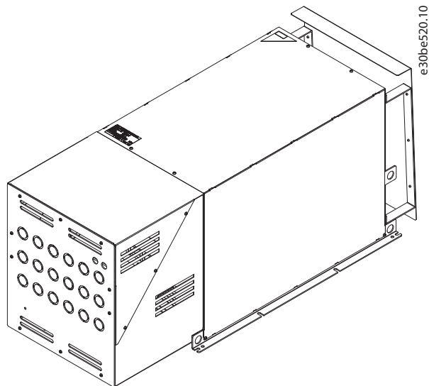
Abbildung 7.49 IP21 X8-V3 interner und externer Lüfter, 3D-Ansicht
