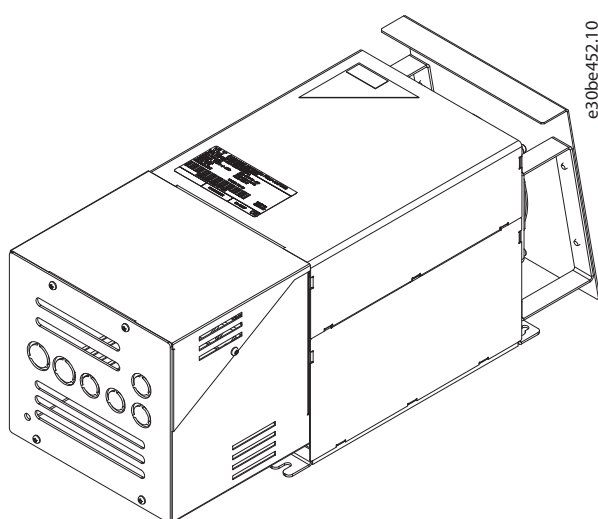
Abbildung 7.35 IP21 X1-V3 interner und externer Lüfter, 3D-Ansicht
