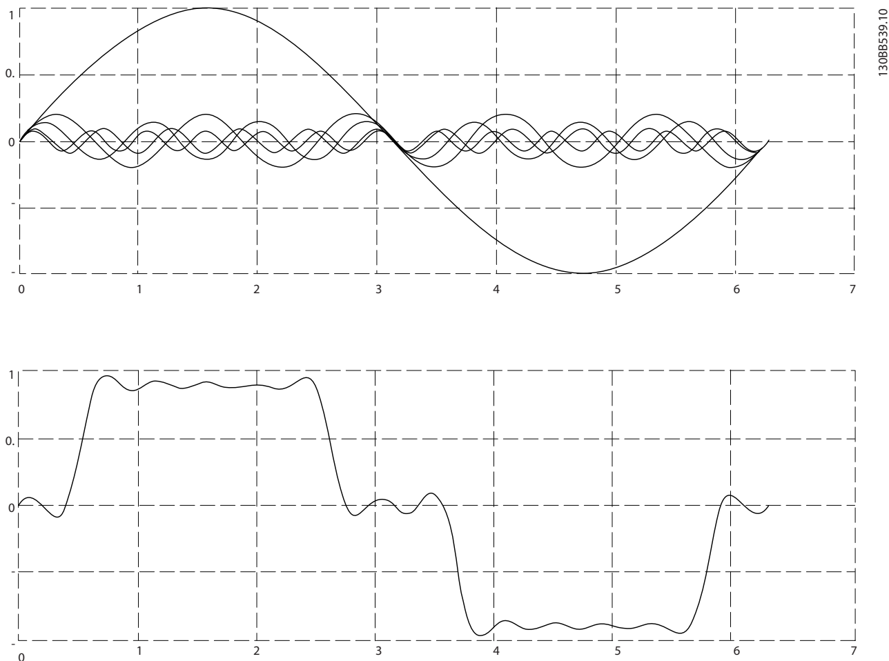
Abbildung 2.3 Sinusförmige Signalkurven
