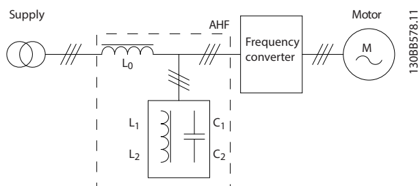
Abbildung 3.1 Funktionsprinzip
