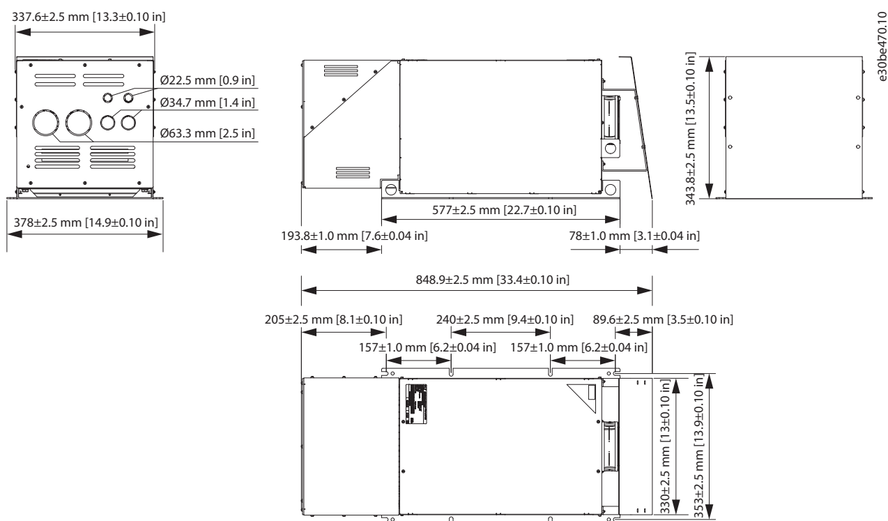
Abbildung 7.40 IP21 X4-V3 interner und externer Lüfter
