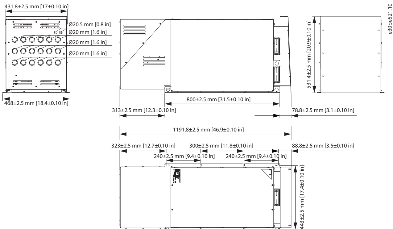
Abbildung 7.48 IP21 X8-V3 interner und externer Lüfter
