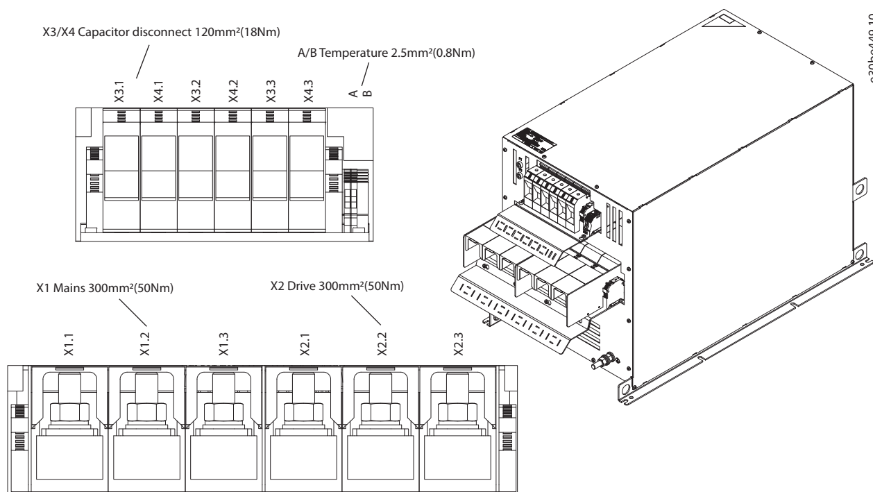
Abbildung 7.33 IP20 X8-V3 Externer Lüfter, Klemmenbezeichnung und 3D-Ansicht
