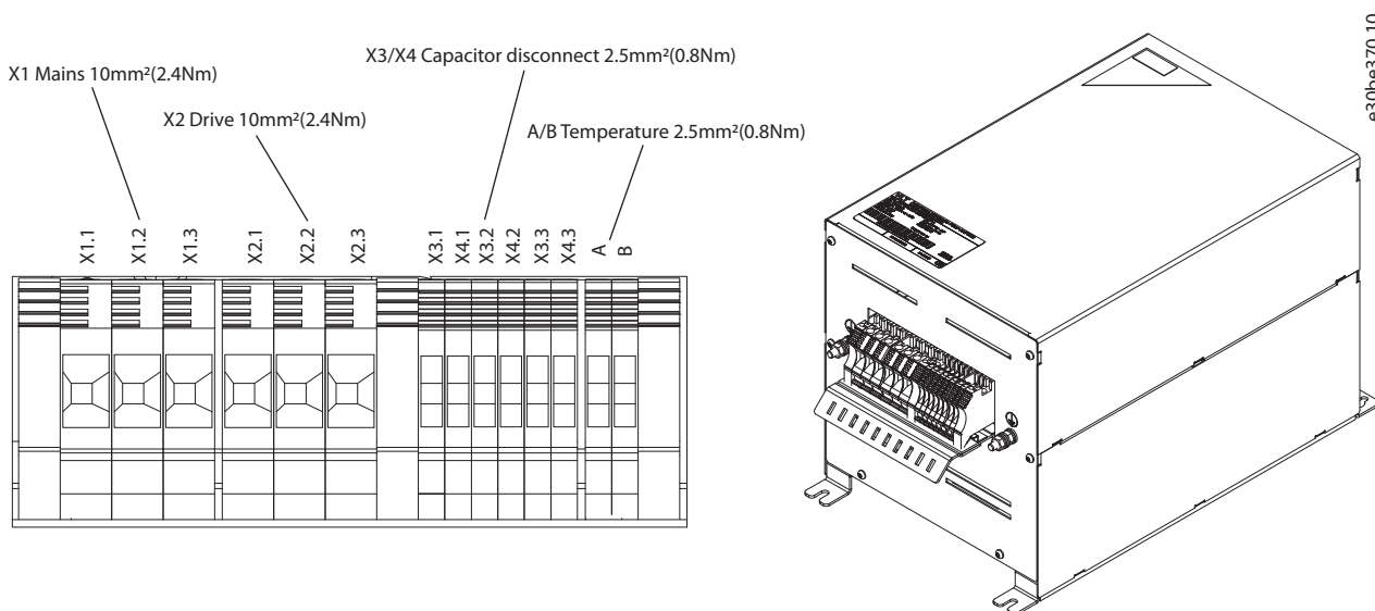
Abbildung 7.7 IP20 X2-V3 Interner Lüfter, Klemmenbezeichnung und 3D-Ansicht
