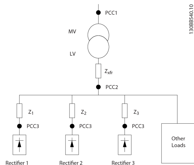
Abbildung 2.4 Kleine Verteilungsanlage
