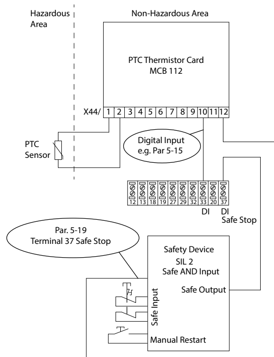
Abbildung 3.3 Kombination einer STO-Anwendung und einer MCB 112-Anwendung
