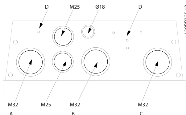
Illustration 5.9 Orifices d'entrée de câble pour protection B1. L'utilisation proposée des orifices n'est qu'une suggestion et d'autres solutions sont possibles.
