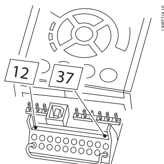
Illustration 2.2 Ponter le cavalier entre la borne 37 et les 24 V CC.
