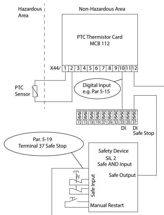
Ilustracja 3.3 Połączenie aplikacji bezpiecznego wyłączenia momentu (STO) z aplikacją MCB 112
