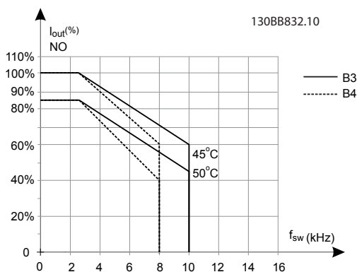
Рисунок 9.11 Снижение номинального тока I_{\text{вых}} при различных значениях T_{\text{окр. ср., макс.}} для корпусов типа В3 и В4 для модели коммутации SFAVM в режиме нормальной перегрузки (перегрузка по крутящему моменту 110 %).
