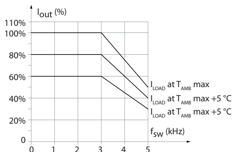
Рисунок 9.7 Снижение номинального тока I_{\text{вых}} при различных значениях T_{\text{окр. ср., макс.}} для корпуса типа АЗ
