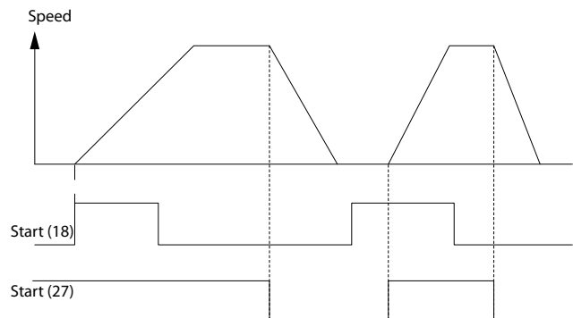
Рисунок 7.2 Клемма 37: Предусматривается только с функцией безопасного отключения крутящего момента.
