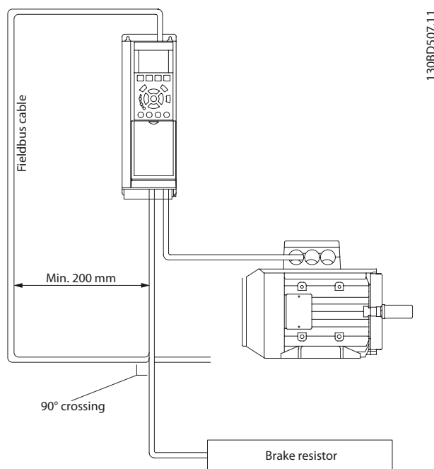
Bild 8.4 Kabeldragning
