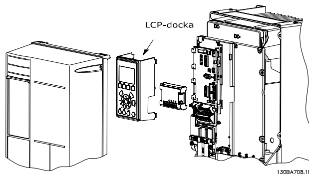
Bild 3.2 Kapslingstyp A5, B1, B2, B4, C1, C2, C3 och C4
