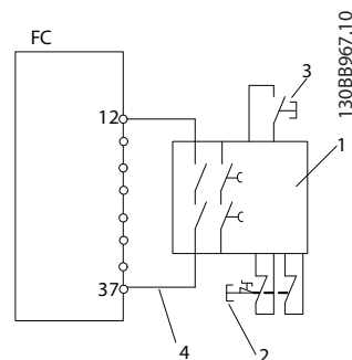
Bild 2.2 Installation för att uppfylla en stoppkategori 0 (SS-EN 60204-1) med säkerhetskat. 3/PL "d" (ISO 13849-1) eller SIL 2 (SS-EN 62061).
