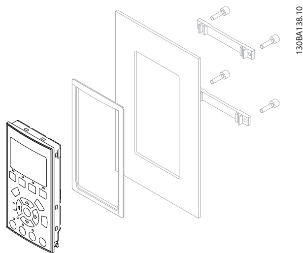
Bild 3.16 LCP-sats med grafisk LCP, fästdon, 3 m kabel och packning Beställningsnr 130B1113
