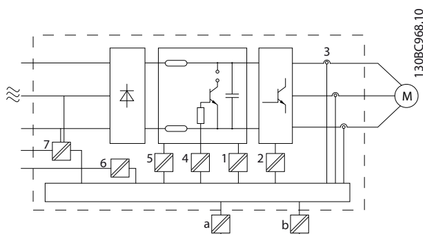
Bild 2.34 Galvanisk isolering
