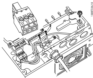
Bild 6.6 Anslutning till nät och jordning utan fränksiljare
