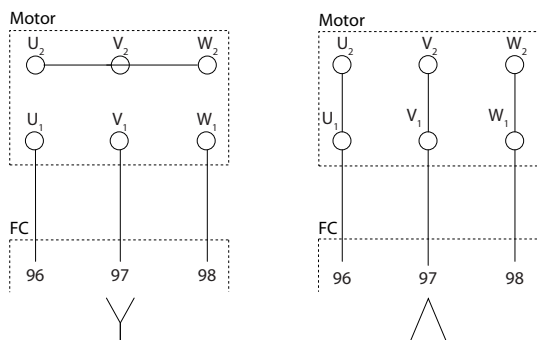
Bild 6.20 Y/D-anlutningar
