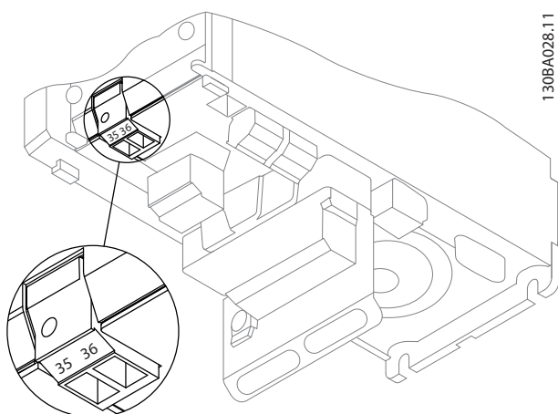
Bild 3.10 Anslutning till 24 V-reservförsörjning (A2-A3).
