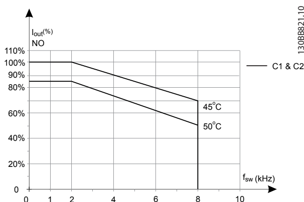
Bild 9.20 Nedstämpling för utström med switchfrekvens och omgivande temperatur för 600 V-frekvensomformare, kapslingstyp C, 60° AVM, NÖ
