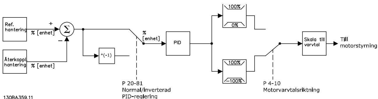
Bild 2.26 Blockdiagram över regulator med återkoppling
