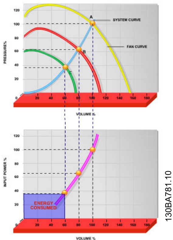
Bild 2.9 När en frekvensomformare används för att minska fläktkapaciteten till 60 % kan energibesparingar på mer än 50 % uppnås i vanliga tillämpningar
