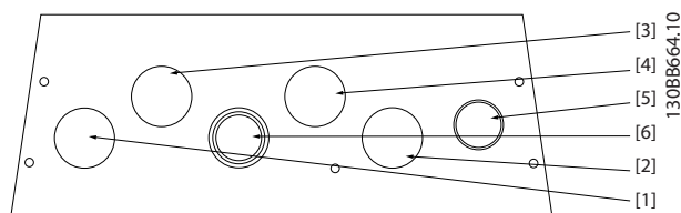
Bild 6.25 A5 - IP55
