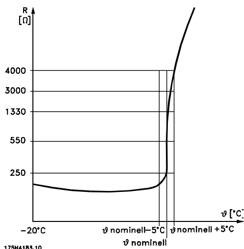
Bild 2.41 Termistorurkoppling
