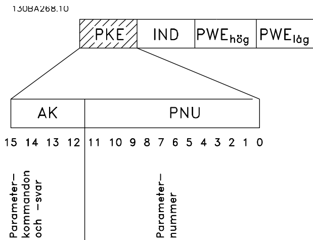
Bild 8.10 PKE-fält
