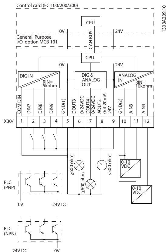
Bild 3.4 Kopplingsschema
