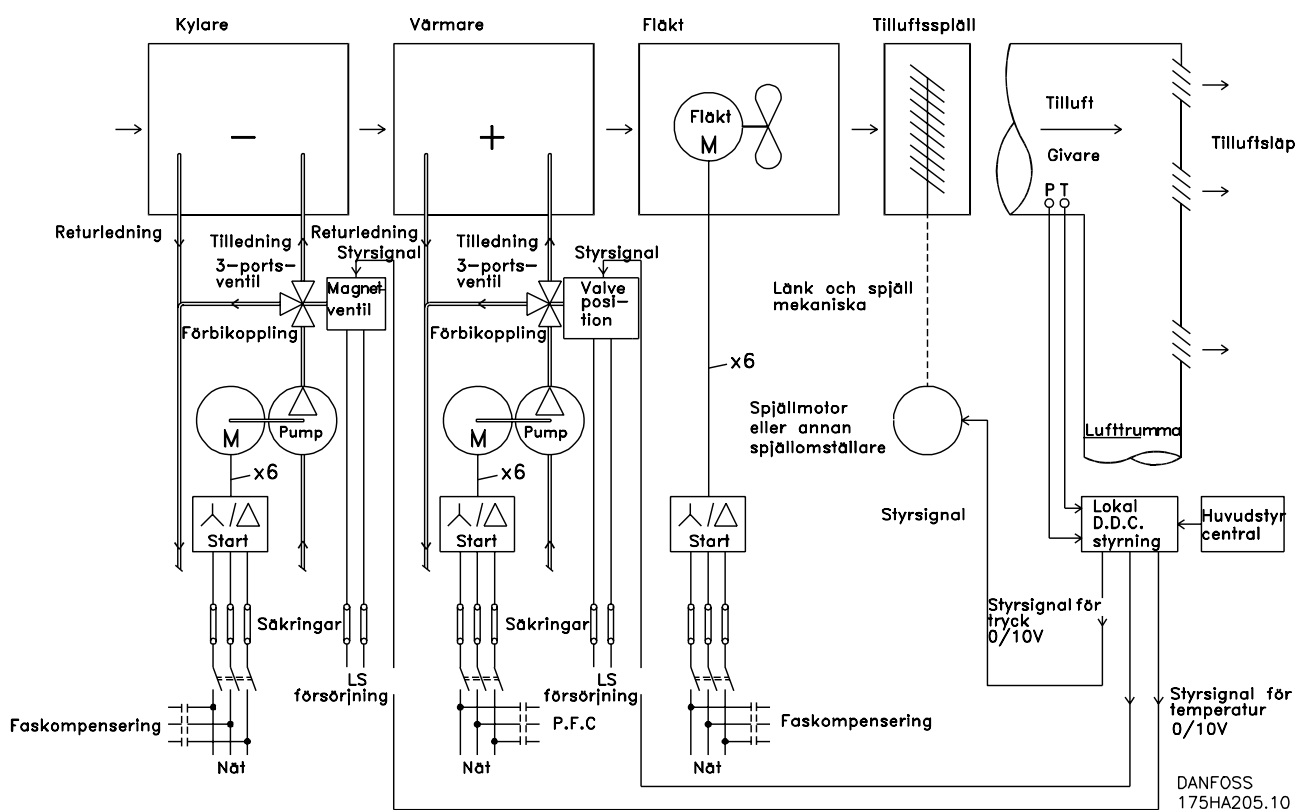
Bild 2.15 Traditionellt fläktsystem
