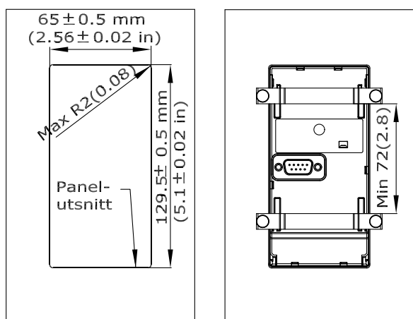
Bild 3.18 Dimensioner
