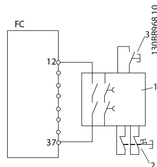
Bild 2.3 STO, exempel
