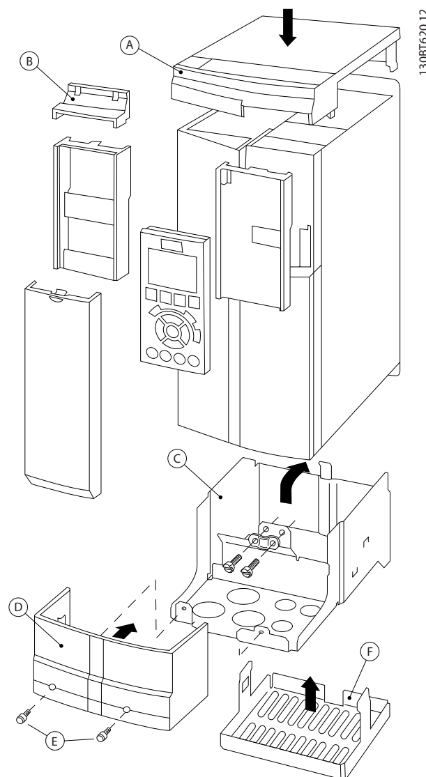
Bild 3.21 Kapslingstyp B3
