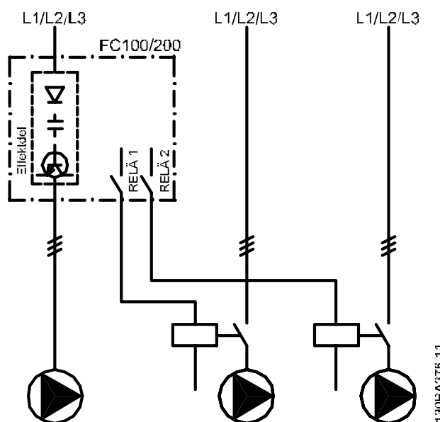
Bild 7.9 Elschema för pump med variabelt varvtal
