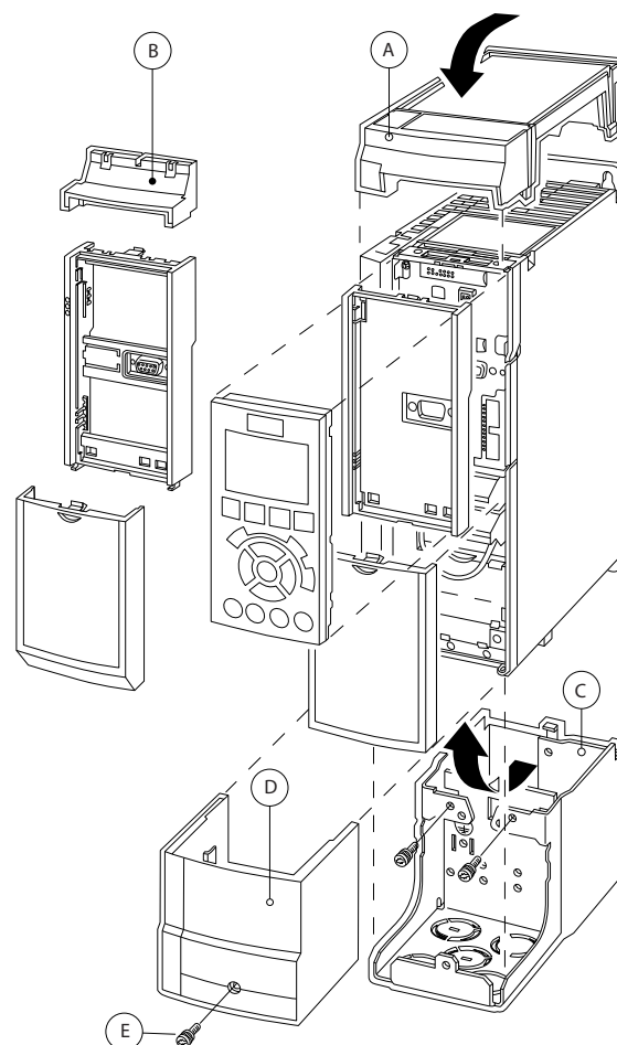
Bild 3.19 Kapslingstyp A2
