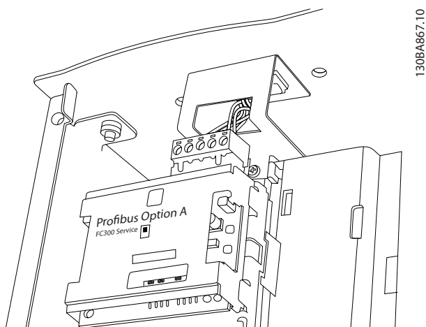
Bild 6.45 Inre placering av fältbuss
