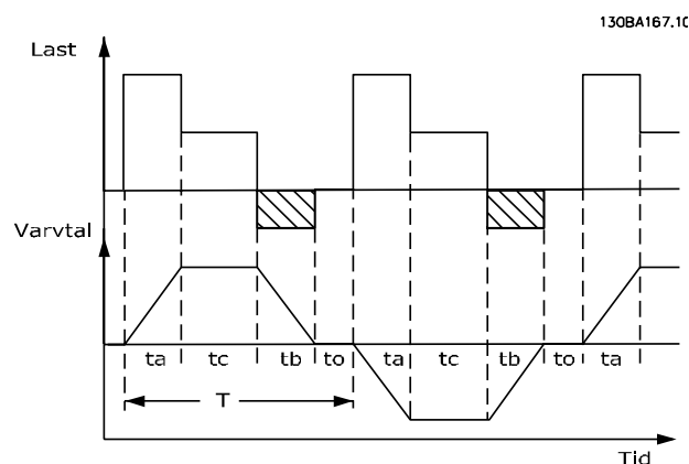
Bild 2.39 Intermittent driftcykel för motståndet
