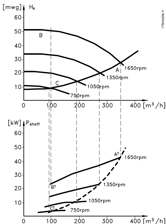
Bild 2.13 Exempel med varierande flöde
