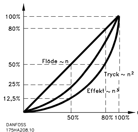
Bild 2.10 Varvtalets påverkan på flöde, tryck och effektförbrukning
