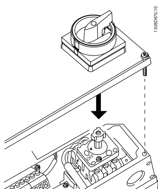
Bild 6.39 Placering av strömbrytaren
