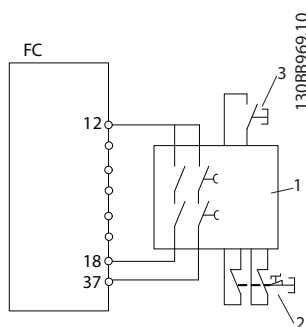
Bild 2.4 SS1, exempel
