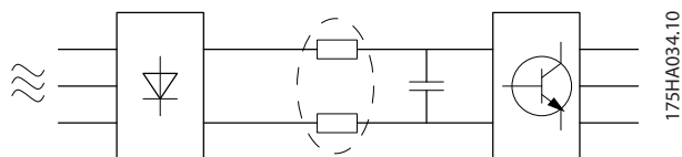
Bild 2.33 Övertensströmmar
