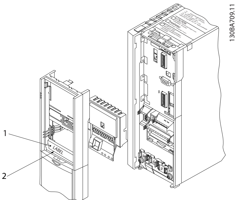
Bild 3.5 Relätillval MCB 105
