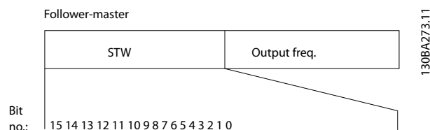
Bild 8.17 Statusord
