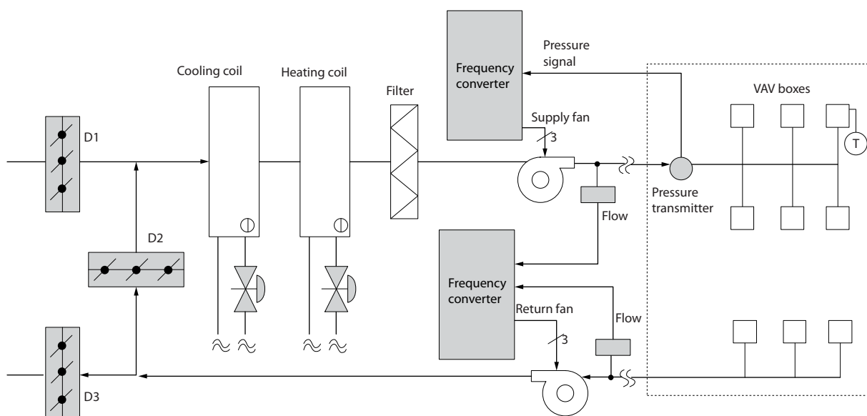
Bild 2.17 Lösning med VLT
