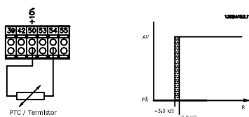
Bild 2.44 Med en analog ingång och 10 V som strömförsörjning
