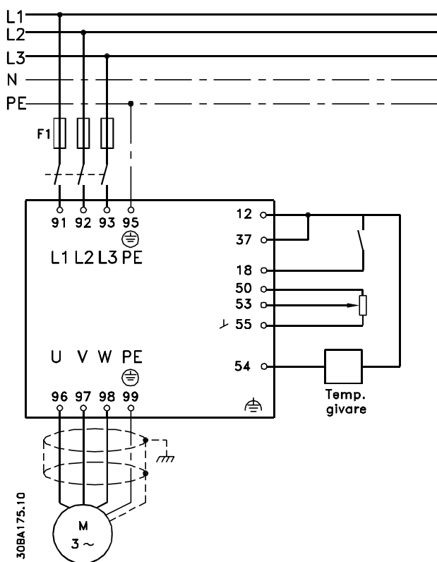
Bild 6.63 Elektriskt anslutningsschema
