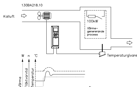
Bild 2.30 Styrning med återkoppling för ett ventilationssystem
