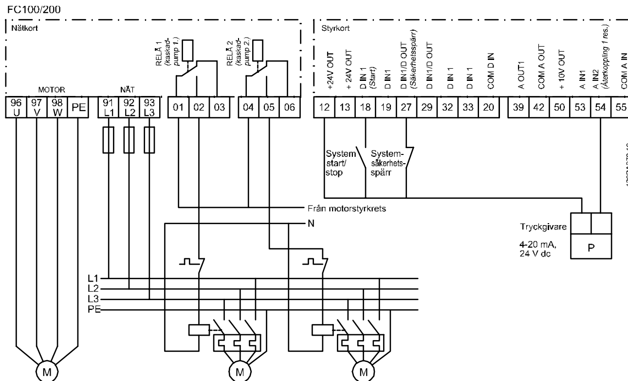
Bild 7.11 Elschema för kaskadregulator
