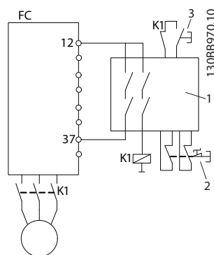
Bild 2.5 STO kategori 4, exempel
