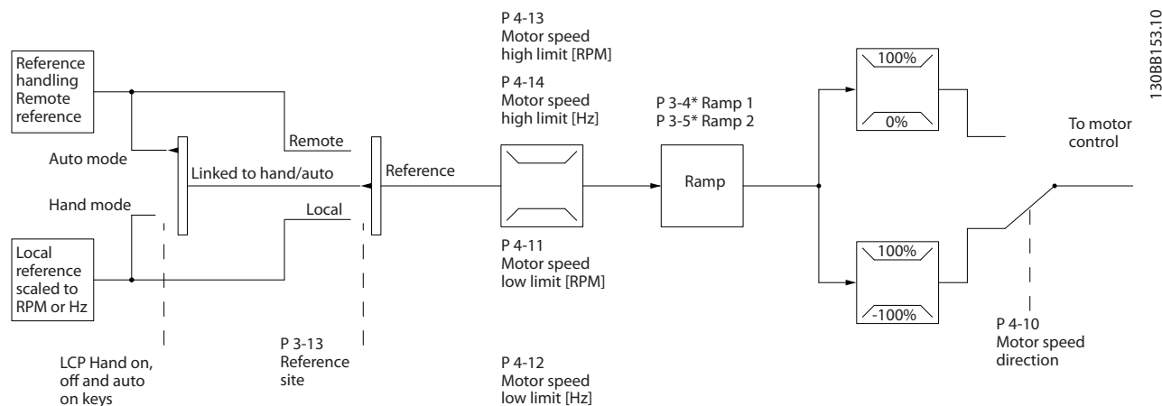
Bild 2.24 Struktur utan återkoppling
