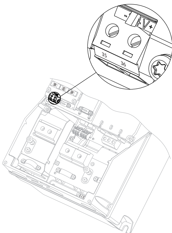
Bild 3.11 Anslutning till 24 V-reservförsörjning (A5-C2).
