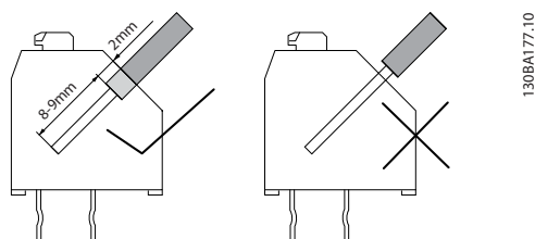
Bild 3.8 Montering
