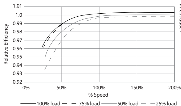
Bild 9.2 Typiska verkningsgradskurvor
