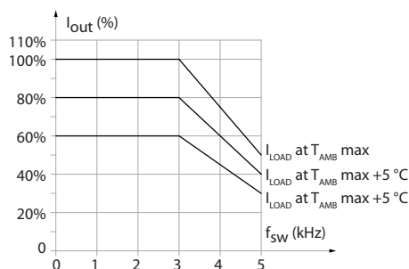
Bild 9.7 Nedstämpling av I_{out} för olika T_{AMB, MAX} för kapslingstyp A3
