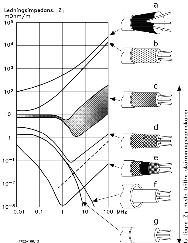
Bild 6.64 Överföringsimpedans
