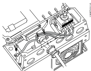
Bild 6.7 Anslutning till nät och jordning med fränksiljare
