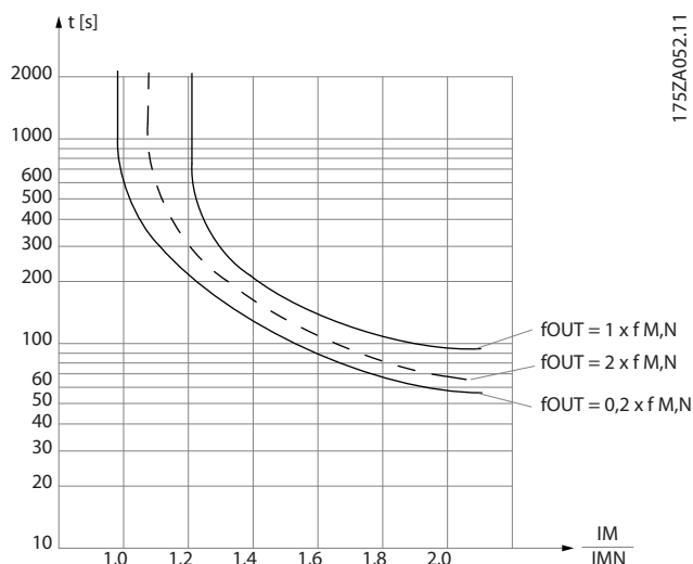
Bild 2.40 X-axeln visar förhållandet mellan I_{\text{motor}} och I_{\text{motor}} nominellt. Y-axeln visar tiden i sekunder innan ETR stänger av och trippar frekvensomformaren. Kurvorna visar det karaktäristiska nominella varvtalet vid dubbla det nominella varvtalet och vid 0,2 x det nominella motorvarvtalet.
