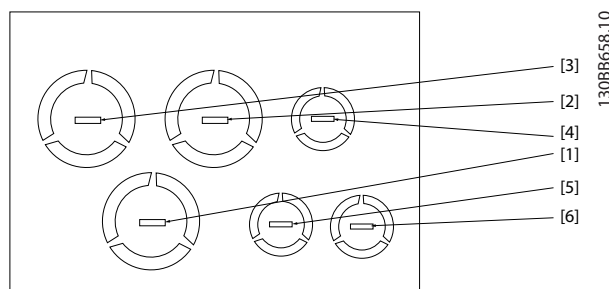
Bild 6.33 B3 - IP21
