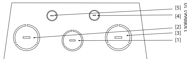
Bild 6.34 C1 - IP21
