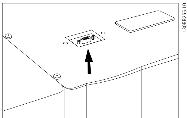
Bild 6.46 Toppanslutning för fältbuss på IP00
