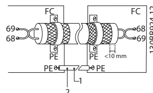
Bild 6.68 Plint 61 ej ansluten
