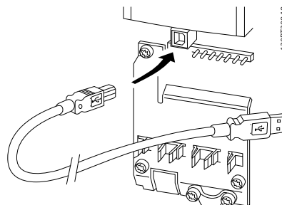
Bild 6.60 USB-anslutning
