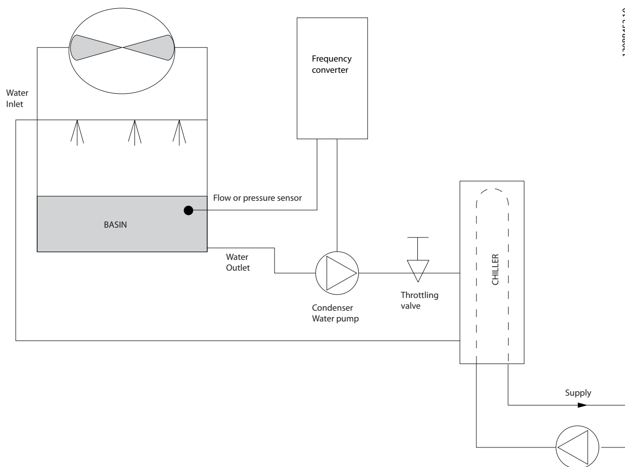
Bild 2.20 Lösning med VLT
