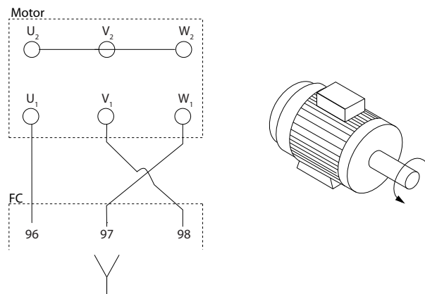
Bild 6.42 Steg för kontroll av motorers rotation
