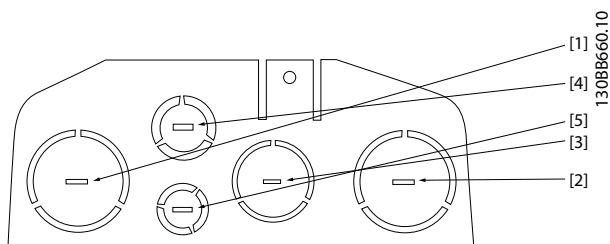
Bild 6.30 B2 - IP21
