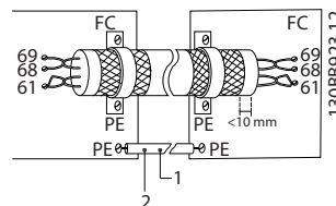
Bild 6.67 Tvinnade parkablar
