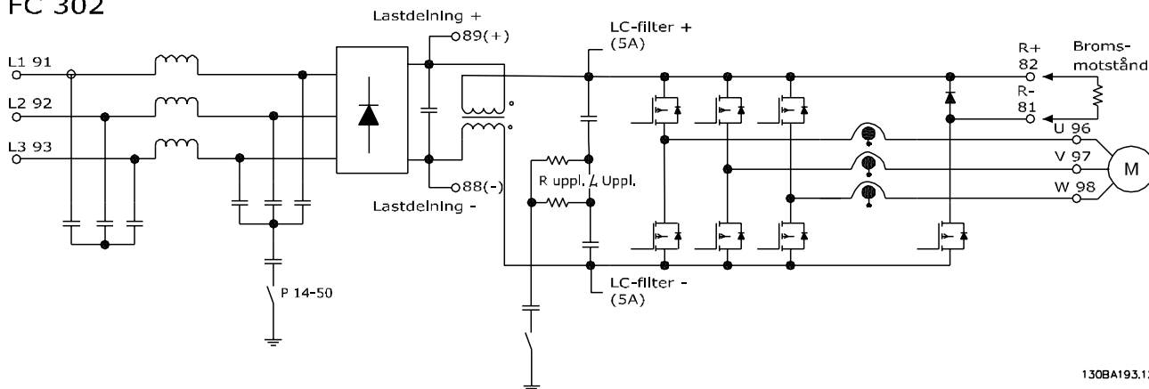
Bild 2.23 Styrstrukturer
