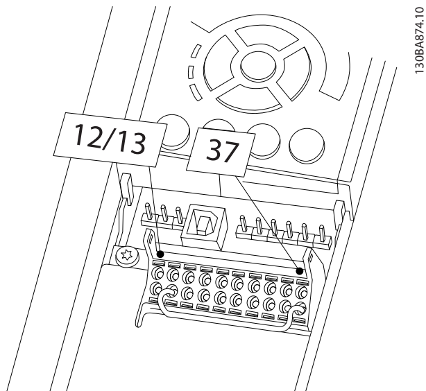
图 3.1 端子 12/13 (24 V) 与 37 (FCD 302 以外的所有变频器) 之间的跳线
