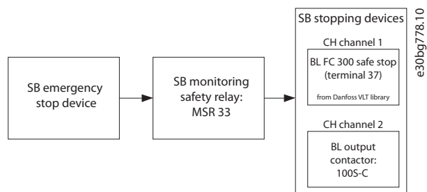
图 5.6 与安全相关的框图
