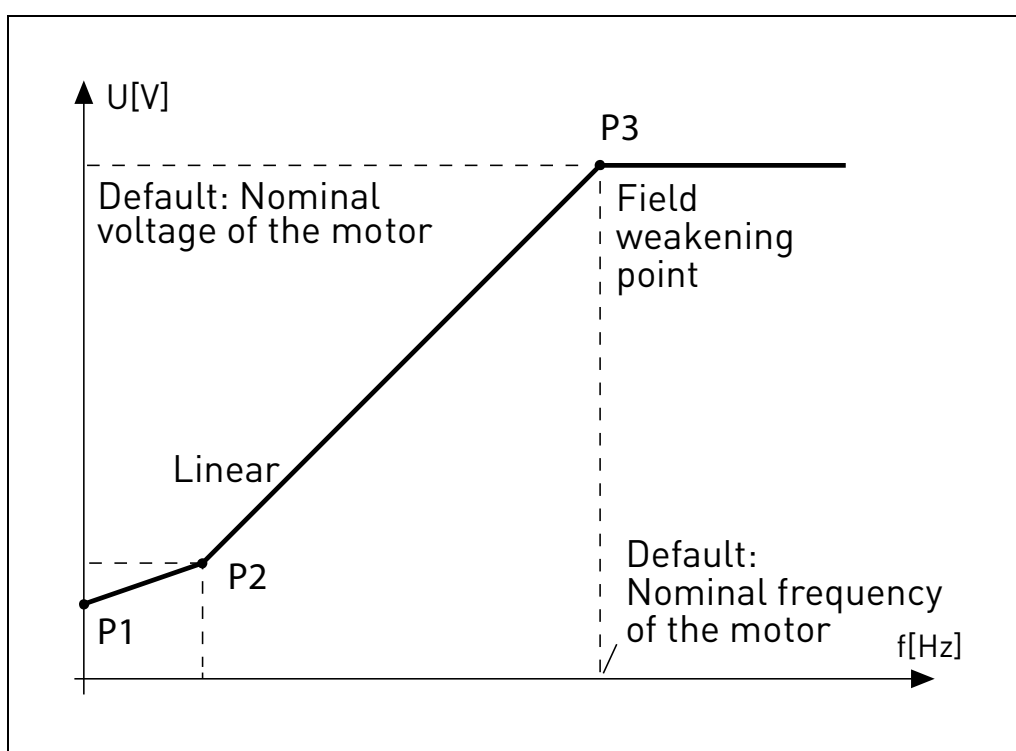
Figura 15. Curva programable.
