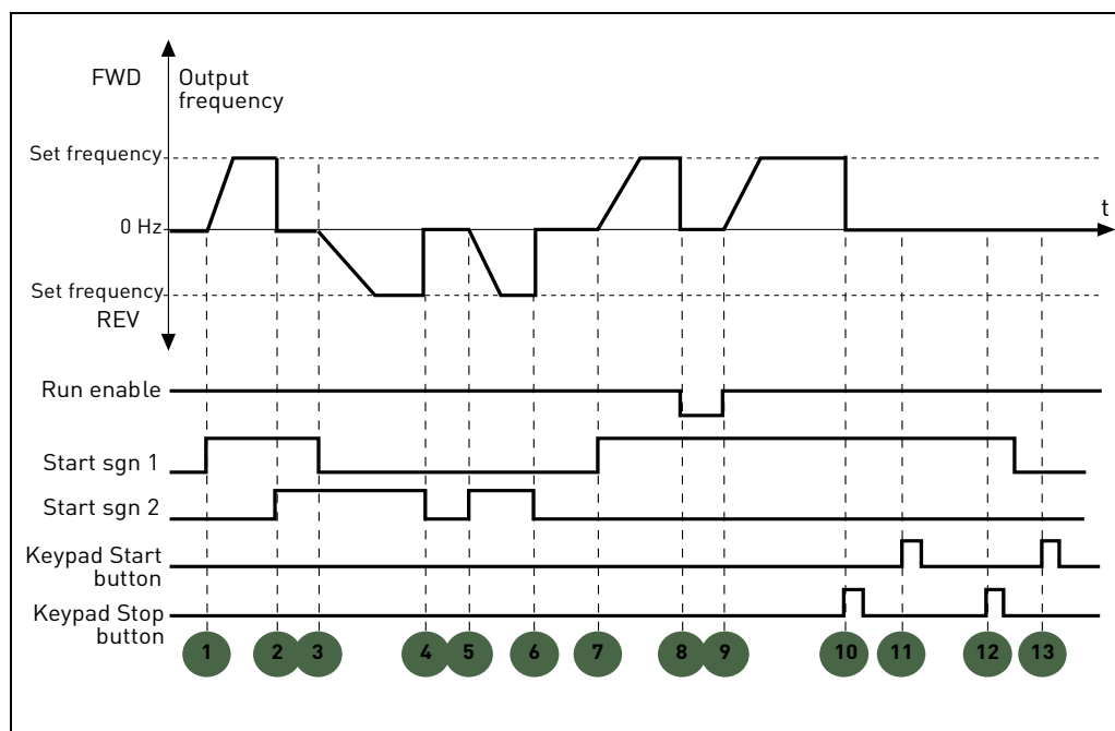
Figura 5. Lógica arranque/parada = 0.
