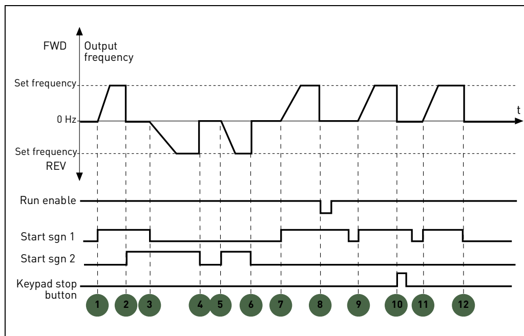
Figura 8. Lógica arranque/parada = 3.
