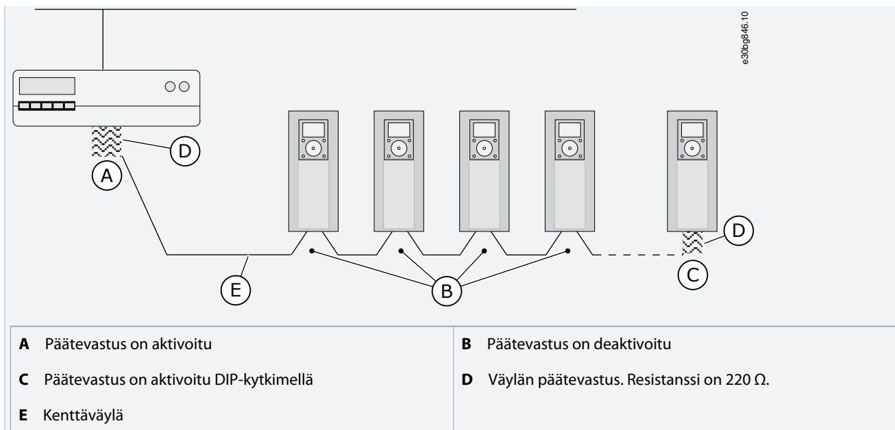
Kuva 40: Kenttäväylälinjan väylän päätevastuksen määrittäminen
