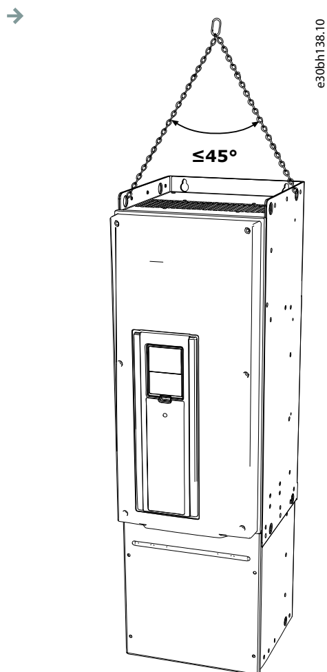
Kuva 2: Suurin sallittu nostokulma
