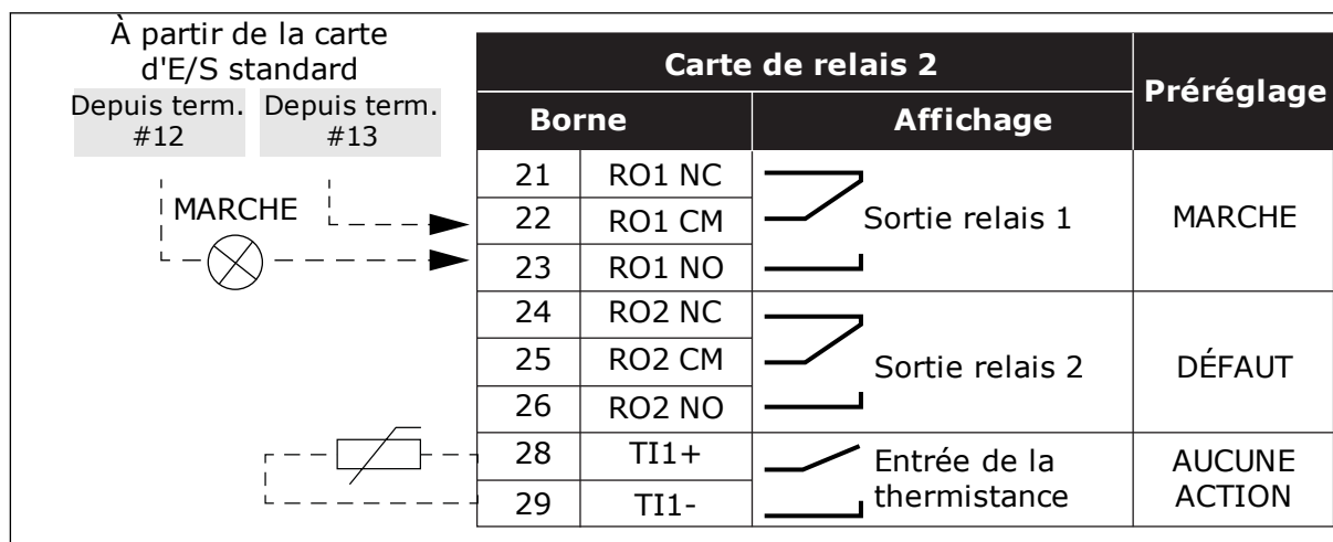
Fig. 41: La carte de relais optionnelle (+SBF4)
