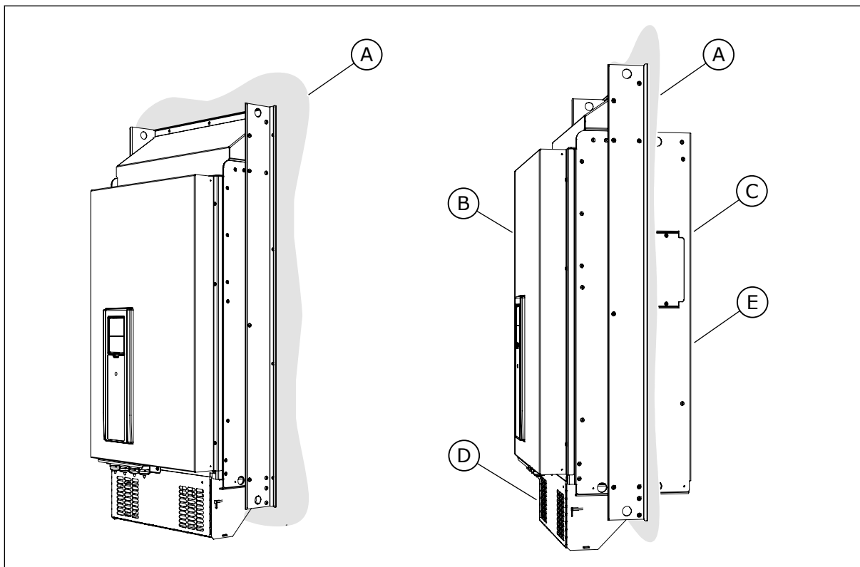
Fig. 18: Exemple de montage traversant (taille MR9)
