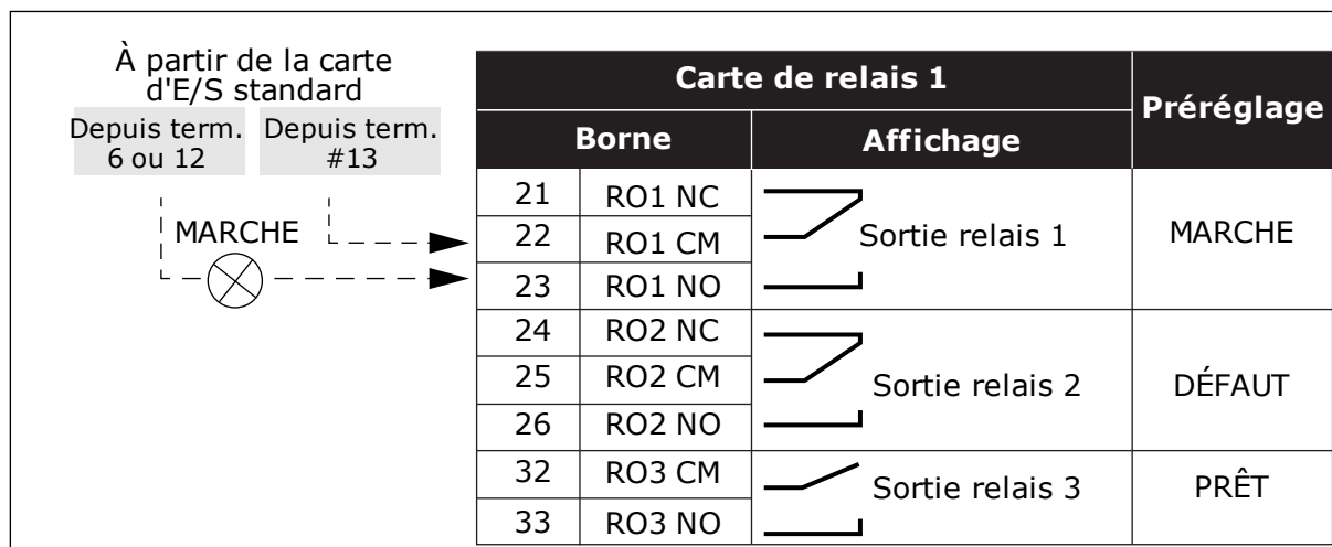
Fig. 40: La carte de relais standard (+SBF3)
