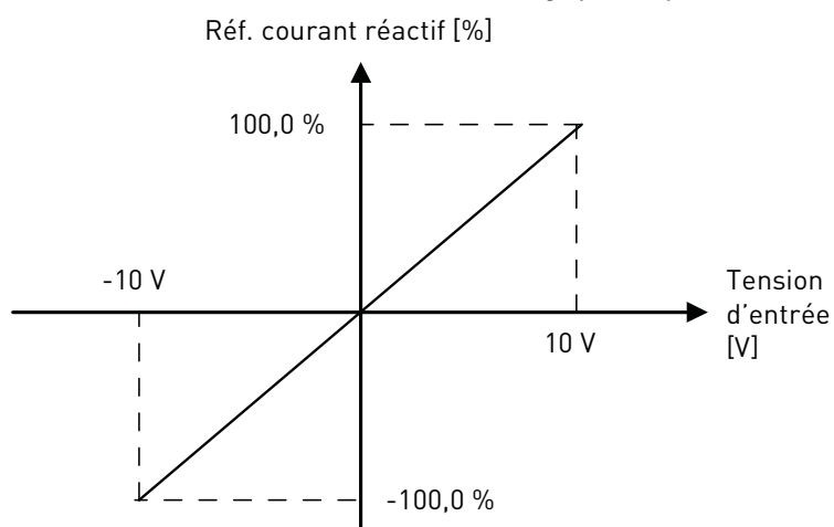
Figure 7. Mise à l'échelle de l'entrée analogique (bipolaire)
