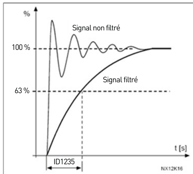
Figure 9. Filtrage de la sortie analogique
