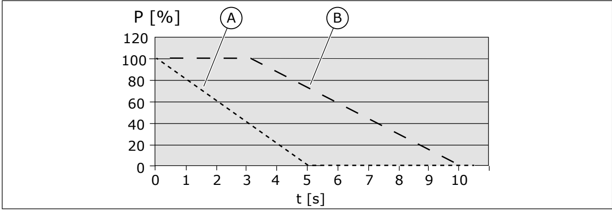
Şekil 48: LD ve HD pulsleri, P = fren gücü
