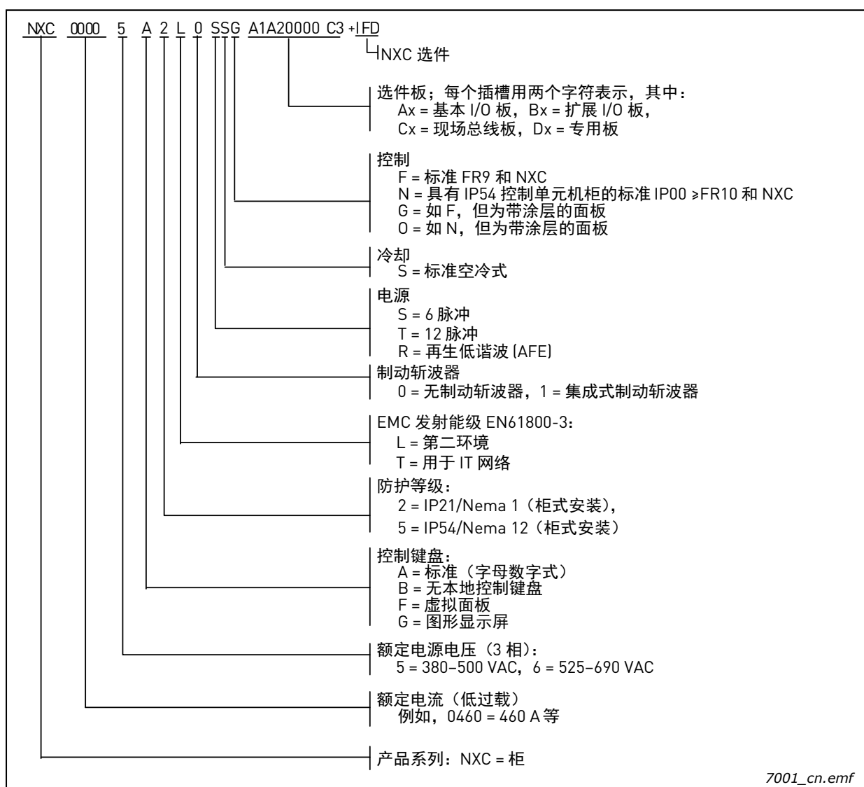
图 1. Vacon NXC 型号代码
