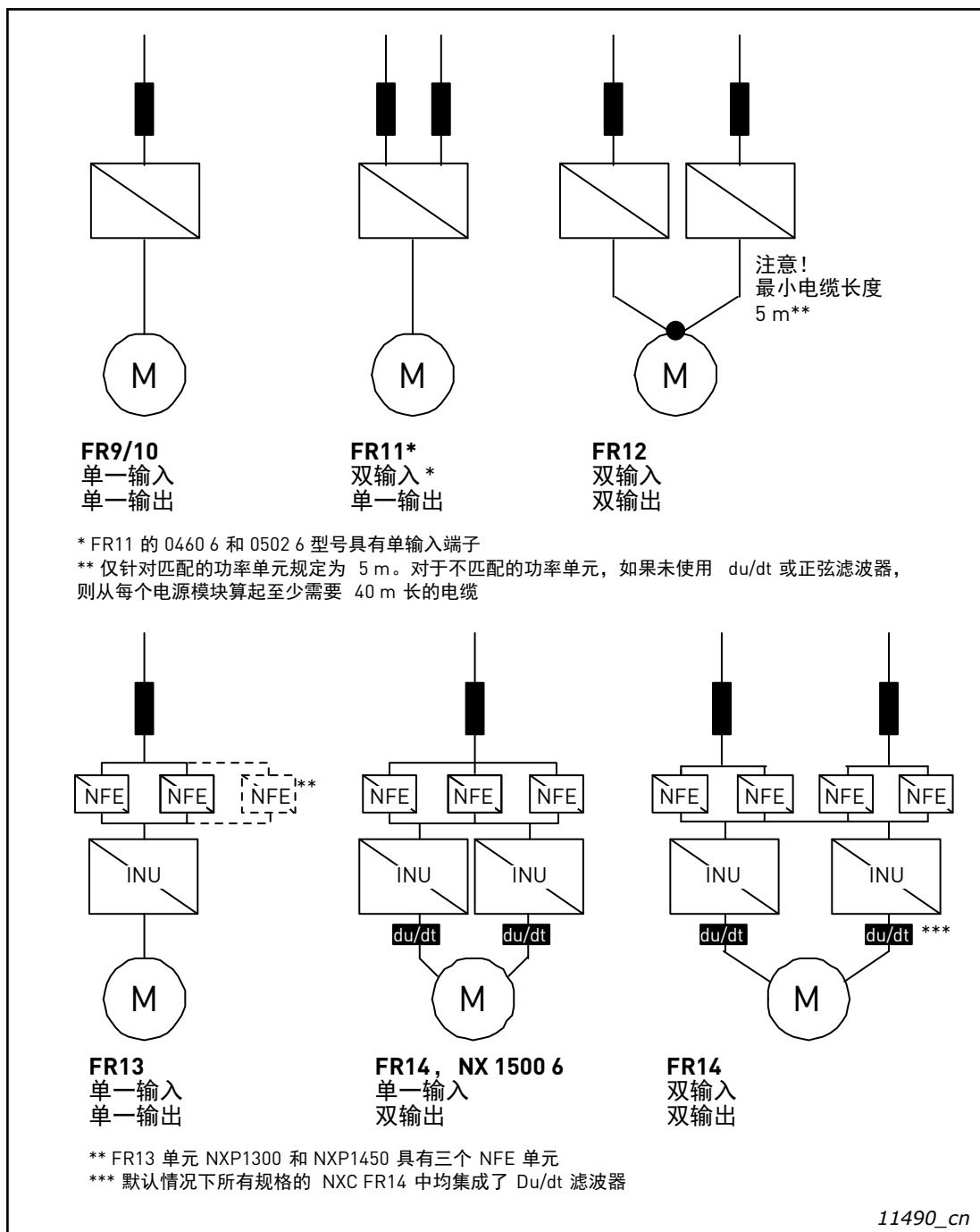
图 9. 机械尺寸 FR9–FR14、6/12 脉冲电源的拓扑结构
