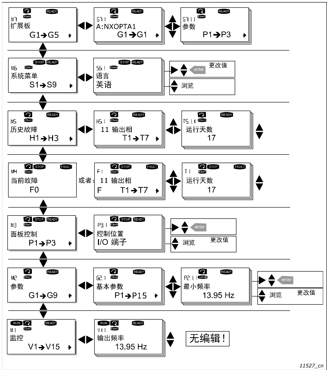
图 44. 面板导航图
