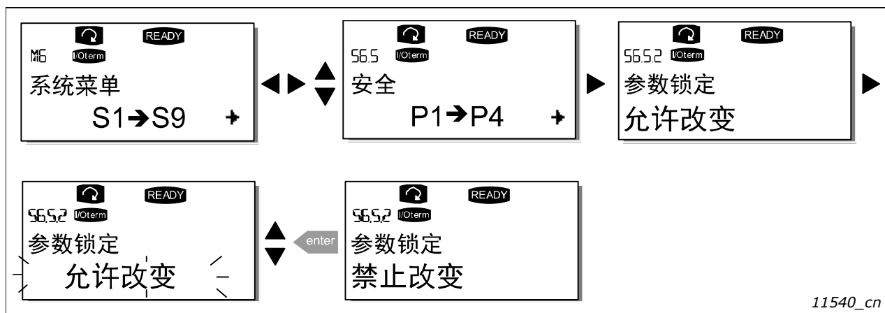
图 56. 参数锁定
