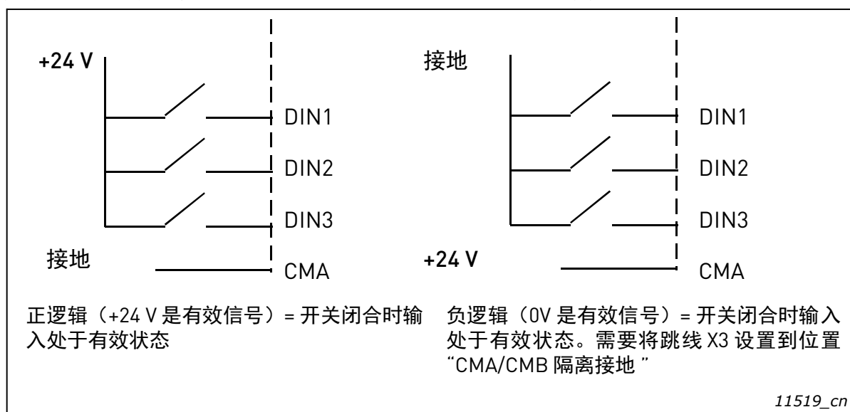
图 37. 正 / 负逻辑
