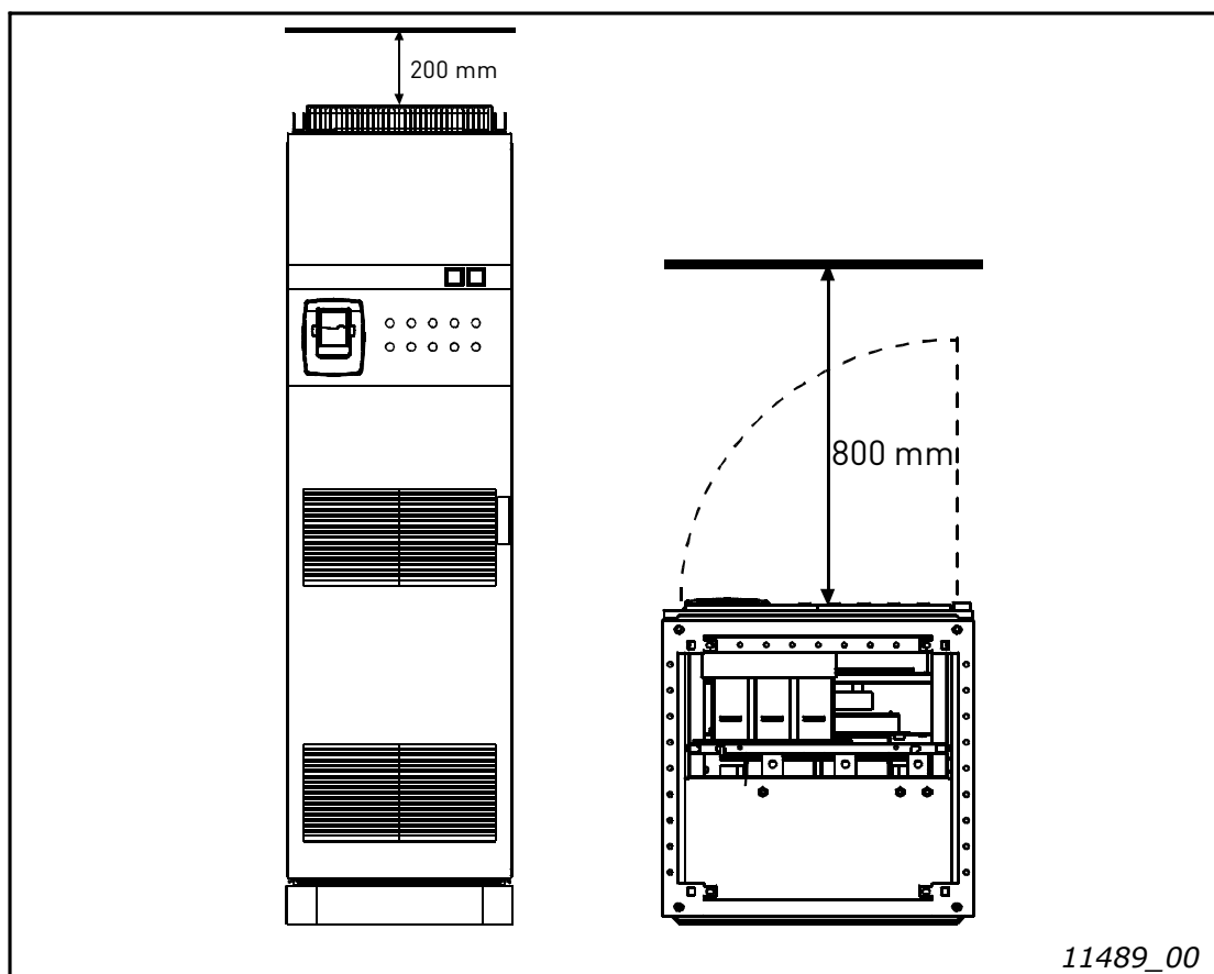
图 8. 在机柜上方（左侧）和前方（右侧）预留的空间
