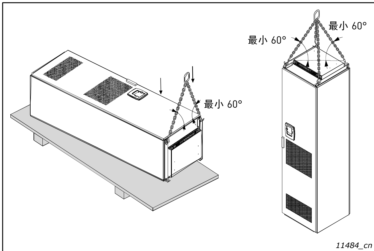
图 3. 吊起装置
