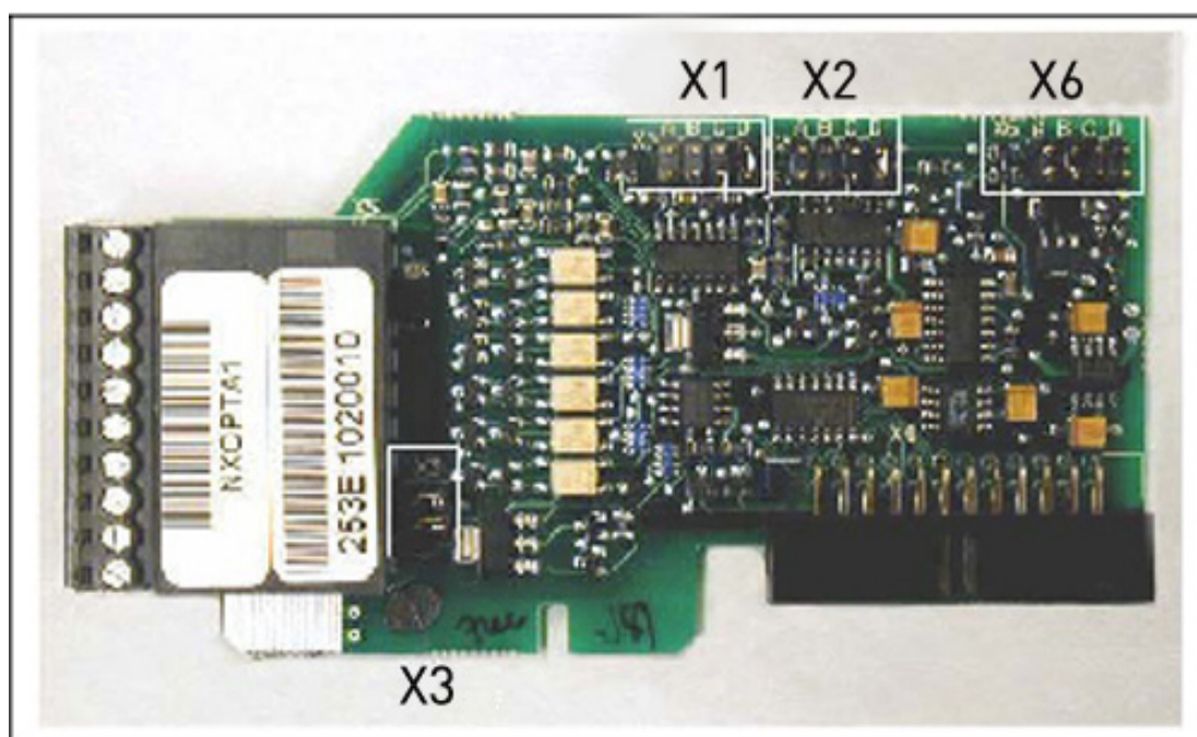
图 38. OPTA1 上的跳线块
