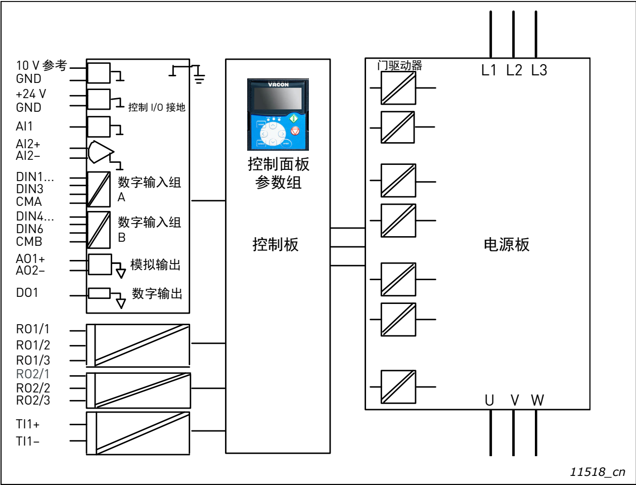
图 36. 电隔离
