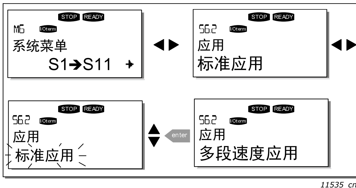
图 51. 应用程序的更改
