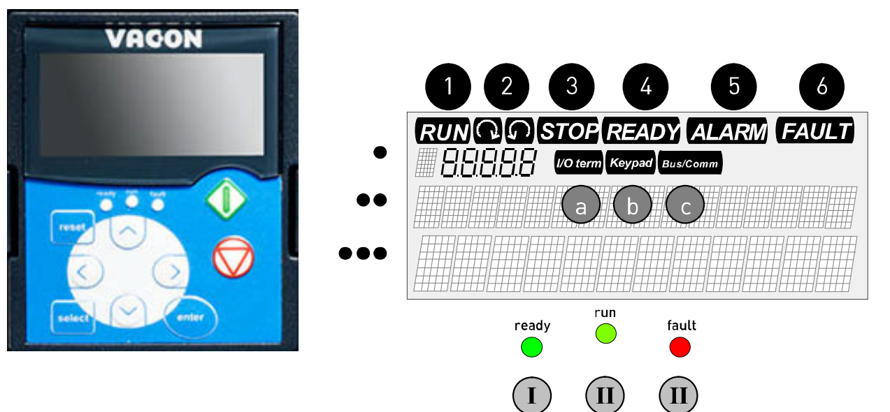
图 42. Vacon 控制键盘和变频器状态指示
