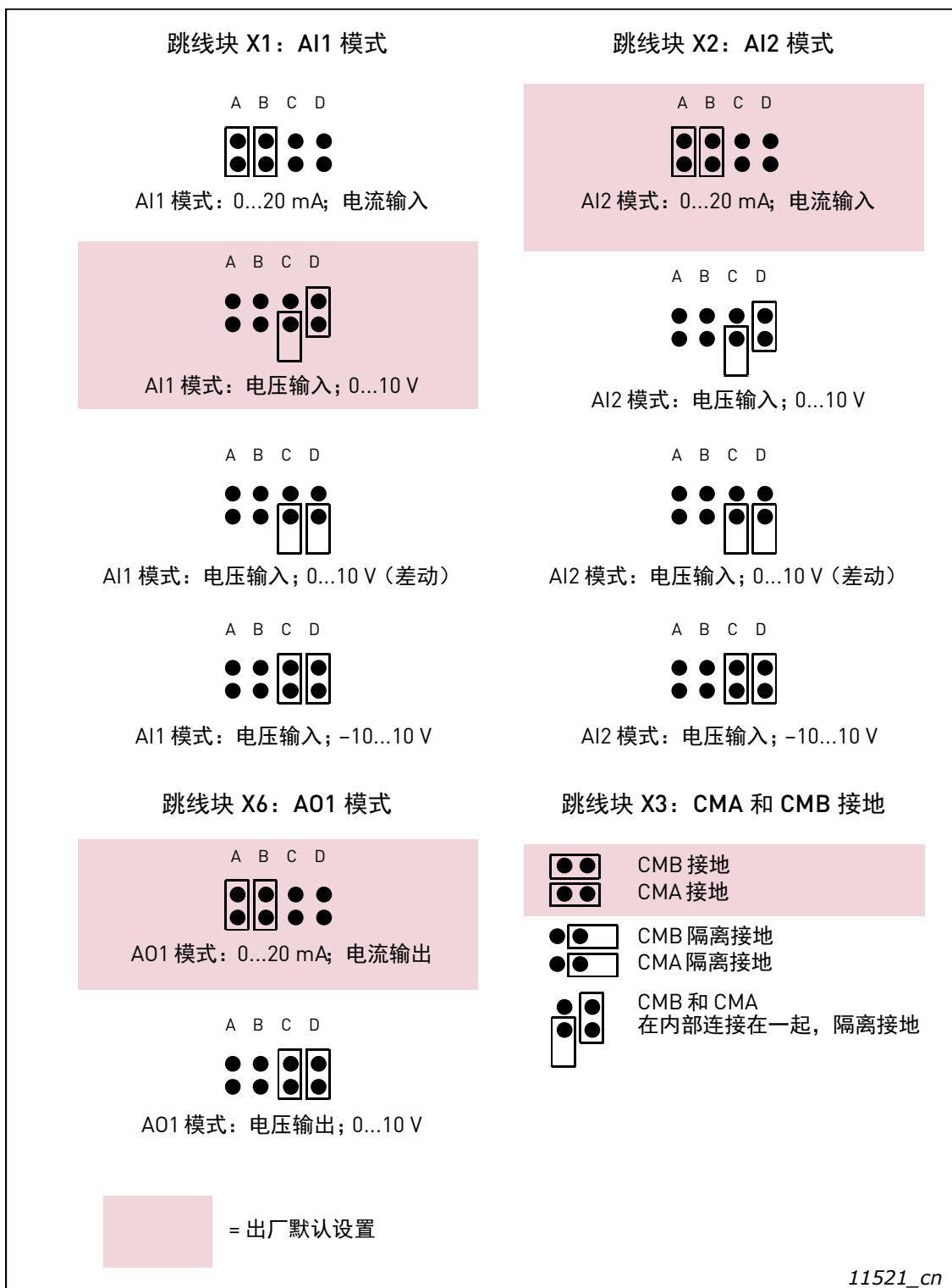
图 39. OPT-A1 的跳线选择
