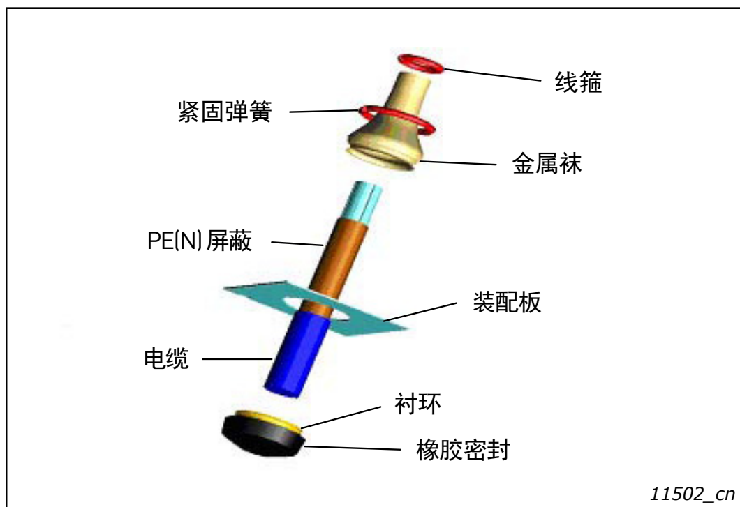
图 23. 电缆密封套组的组件
