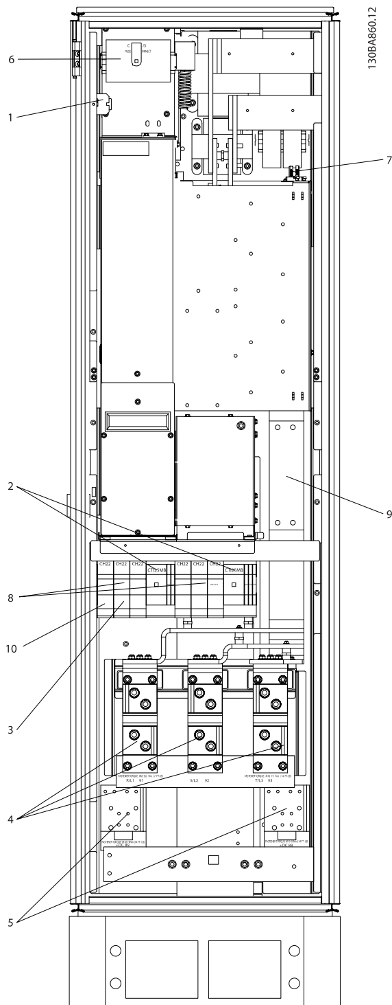
Illustration 4.31: Vekselretterkabinet, stelstørrelse F17
