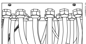
Illustration 4.24: Eksempel på korrekt installation af tætningspladen.
