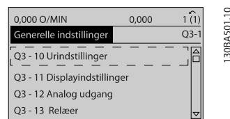
Illustration 6.6: Trin 5: Brug pil op/ned til at rulle ned til f.eks. 03-12 Analoge udgange . Tryk på [OK].
