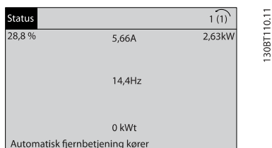
Illustration 6.2: Trin 1: Tænd frekvensomformeren (aktive LED-lamper)
