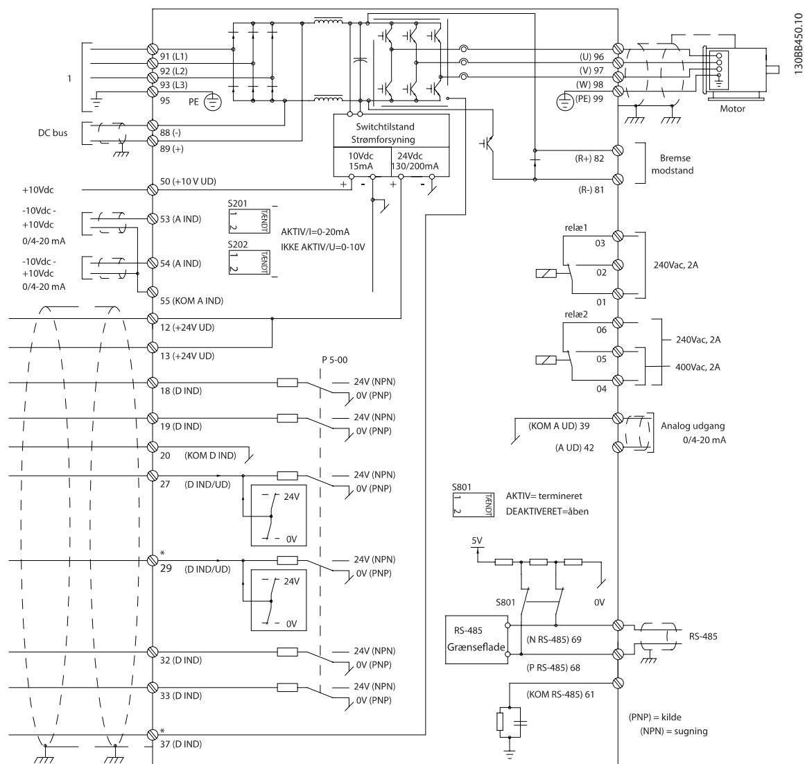
Illustration 4.34: Kurvebladet viser alle elektriske klemmer uden optioner.
