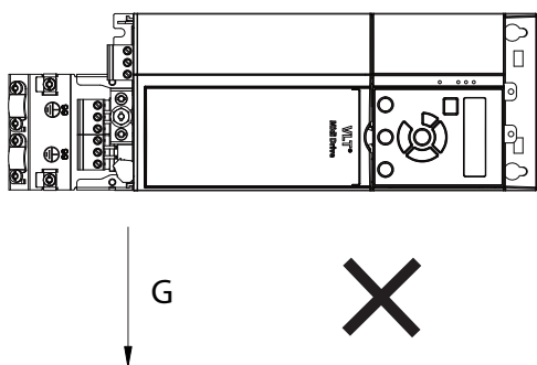
Illustration 3.4 Montage horizontal incorrect (côté droit vers le bas)
