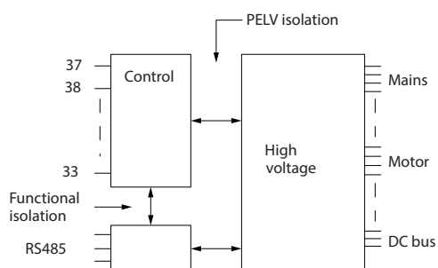
Slika 9.1 Galvanska izolacija
