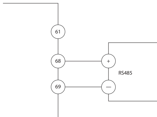
Illustration 4.12 Forbindelsesdiagram for seriel kommunikation
