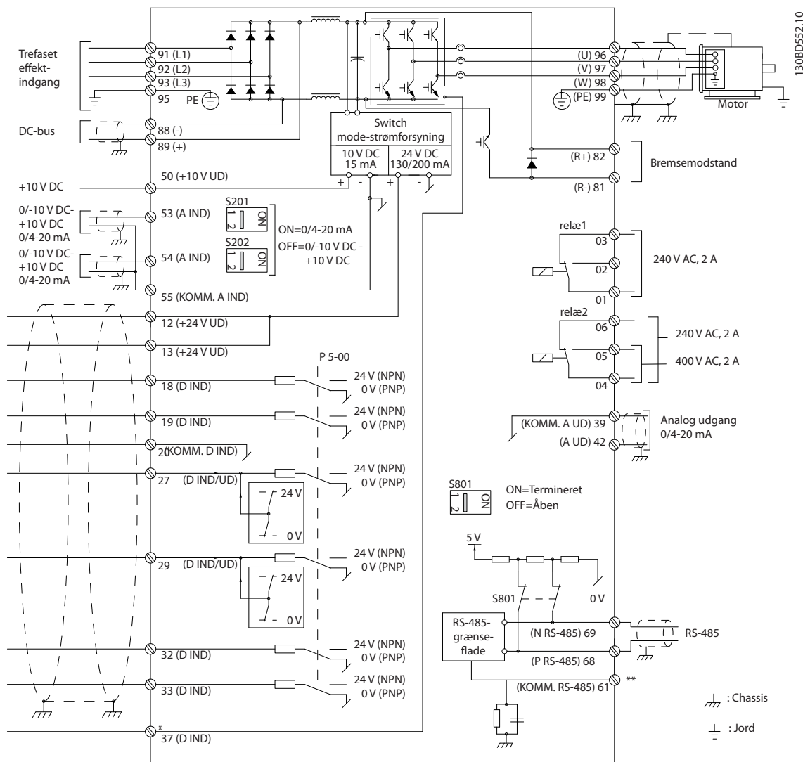
Illustration 4.2 Grundlæggende ledningsdiagram
