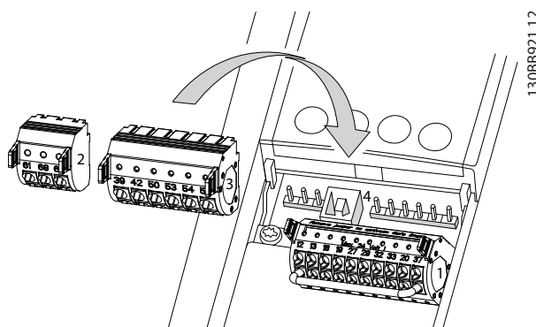
Illustration 4.8 Styreklemmeplaceringer
