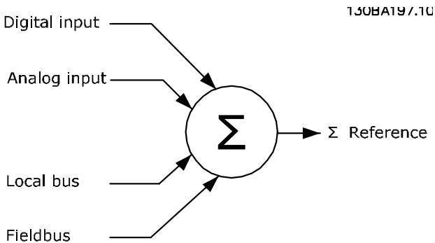
Abbildung 4.2 Sollwert
