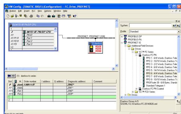
Abbildung 3.6 Einstellen der peripheren Eingangs- und Ausgangsdaten
