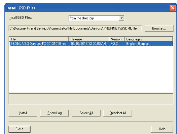
Abbildung 3.2 Fügen Sie eine neue GSDML-Datei im Simatic Manager-Software-Tool hinzu.
