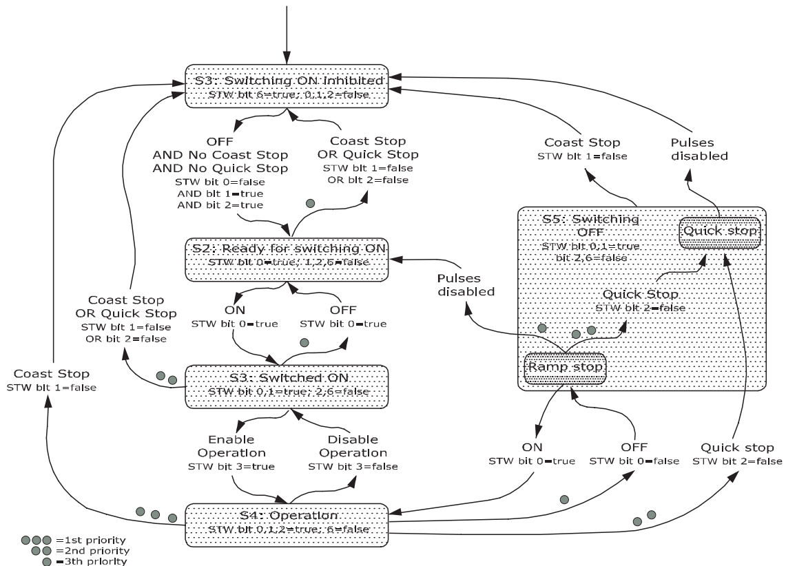
Abbildung 4.4 Übergangsdiagramm PROFIdrive-Zustand
