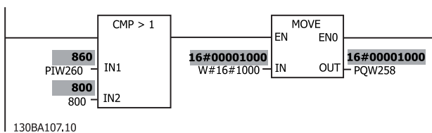
Abbildung 7.4 Netzwerk liest das Motordrehmoment
