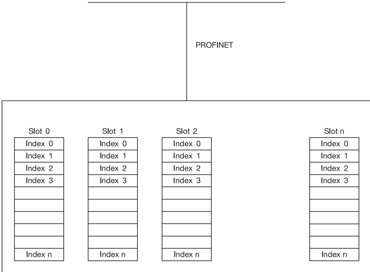
Abbildung 5.1 PROFINET I/O-Gerätestruktur
