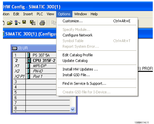
Abbildung 3.1 Importieren Sie die GSDML-Datei in das Konfigurations-Tool.
