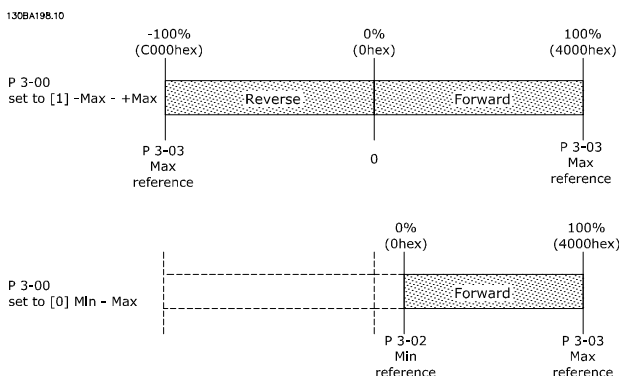
Abbildung 4.3 Sollwert (MRV) und Istwert (HIW), Skaliert
