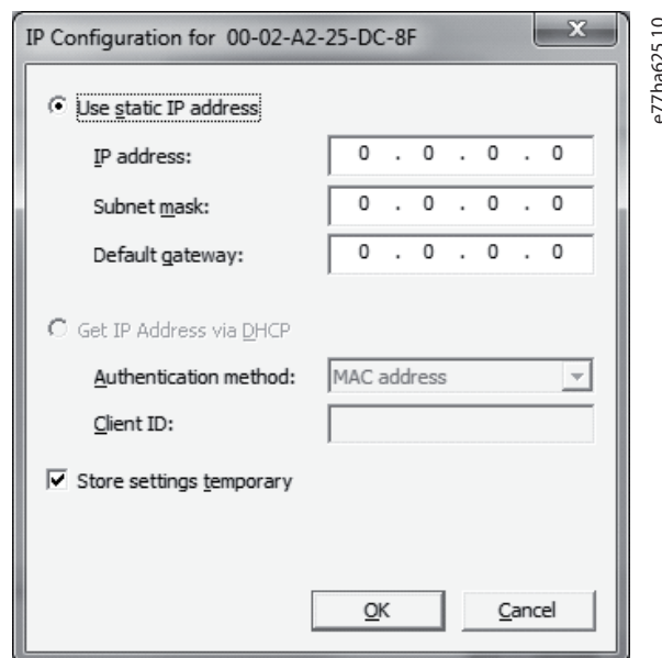
Ilustracja 5.3 Ustawianie statycznego adresu IP
