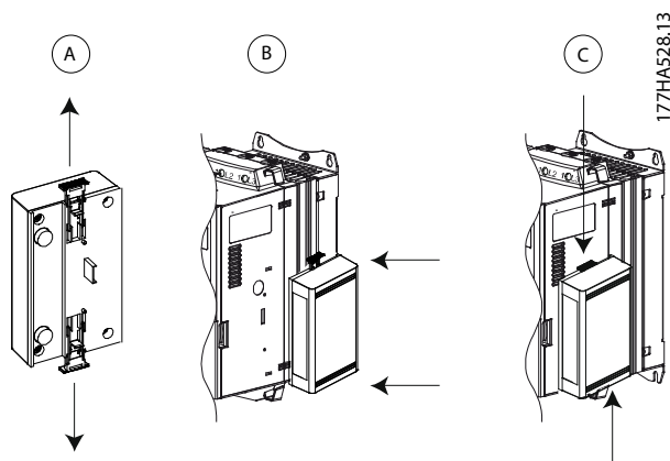
Ilustracja 3.1 Instalowanie modułu PROFINET
