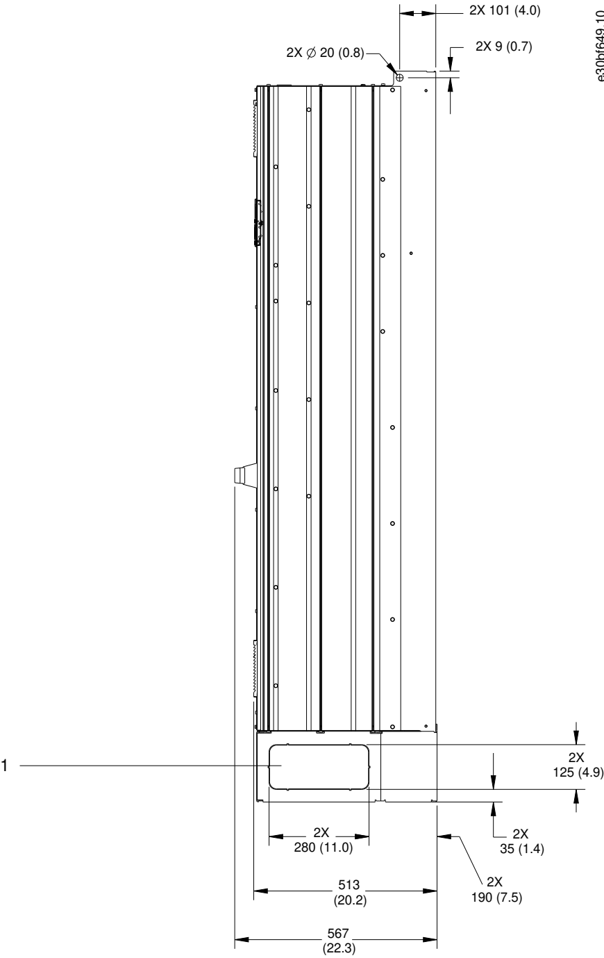
图解 54: E1h 的侧视图
