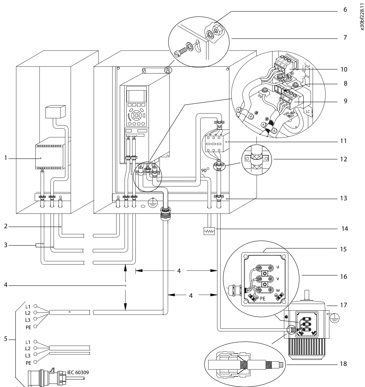
图解 17: 正确的 EMC 合规安装示例
