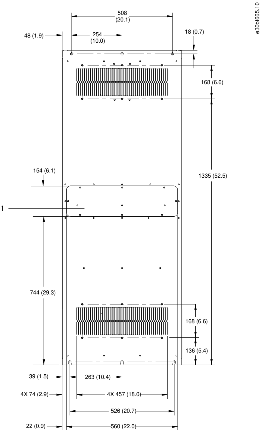
图解 67: E4h 的后视图
