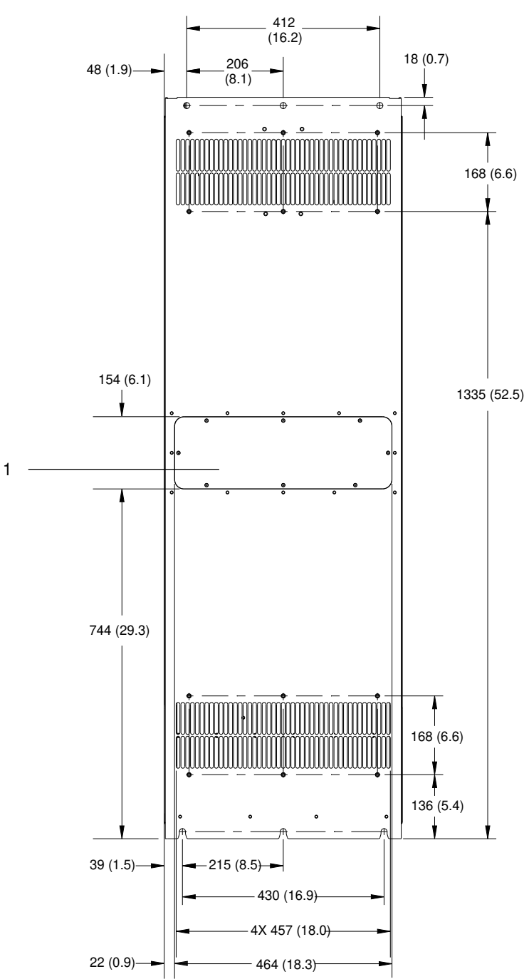
图解 63: E3h 的后视图
