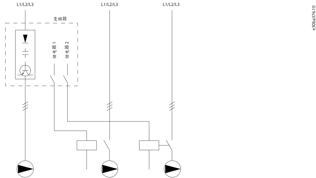
图解 46: 恒速泵/变速泵接线图
