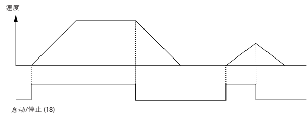
图解 41: 带 Safe Torque Off 选项的启动/停止命令
