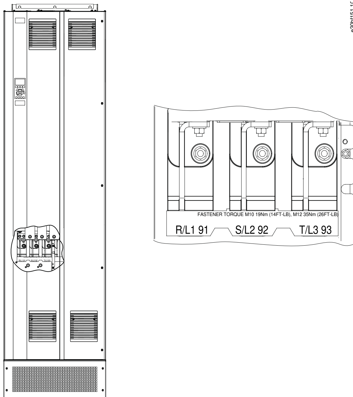
图解 20: 交流主电源端子（所示为 E1h）。
