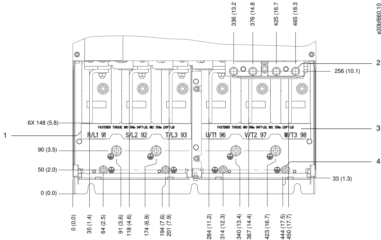
图解 26: E3h 端子尺寸 (正视图)
