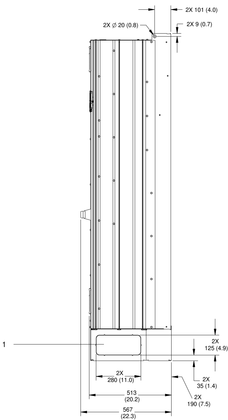
图解 58: E2h 的侧视图
