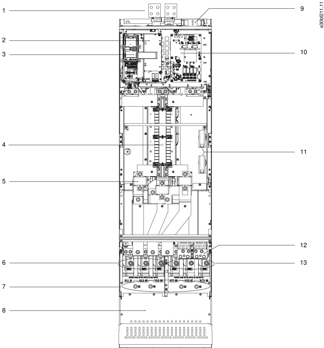
图解 3: 机箱 E3h 的内部视图 (机箱 E4h 与此类似)
