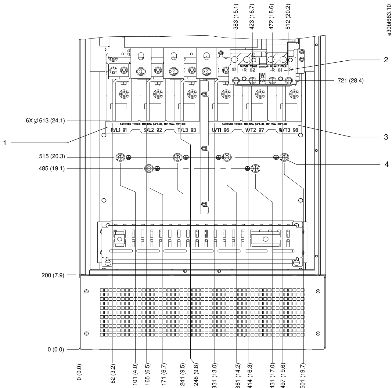
图解 22: E1h 端子尺寸 (正视图)
