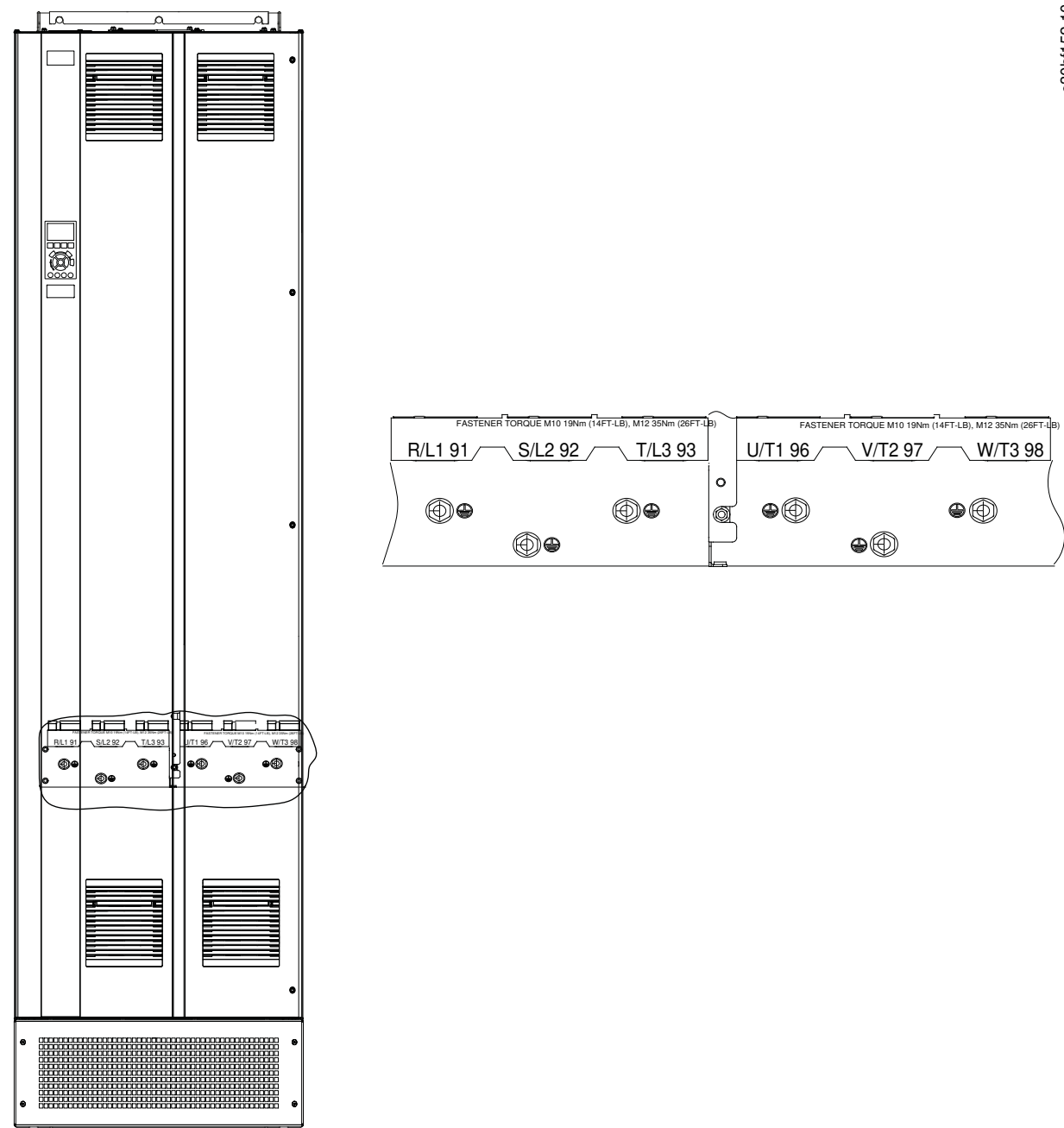
图解 21: 接地端子（所示为 E1h）。
