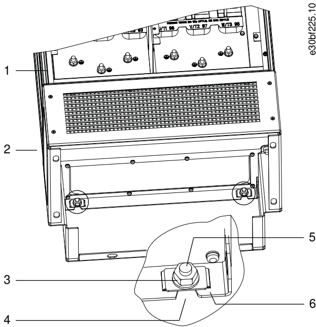
图解 11: 机箱背部的底座安装点
