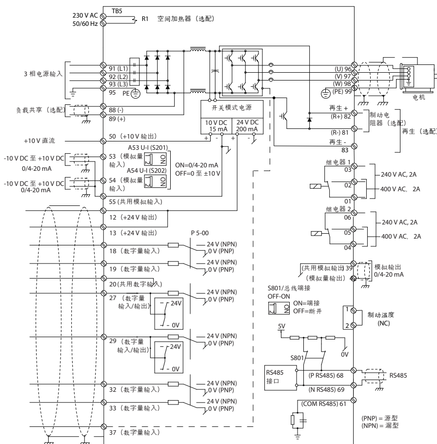
图解 18: 基本接线示意图
