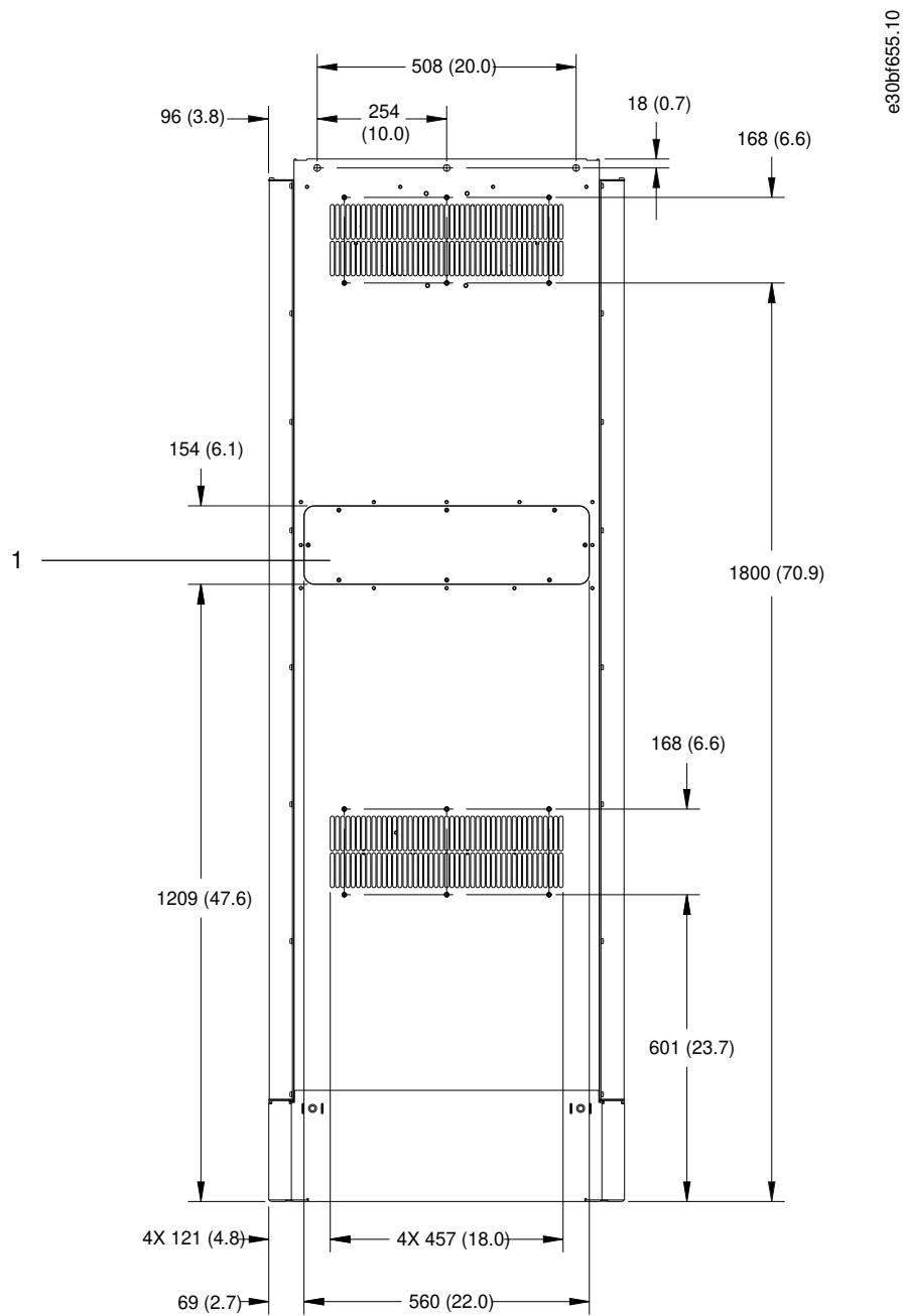
图解 59: E2h 的后视图
