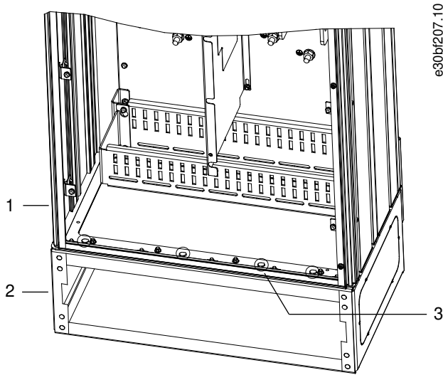
图解 12: 机箱上的底座安装点
