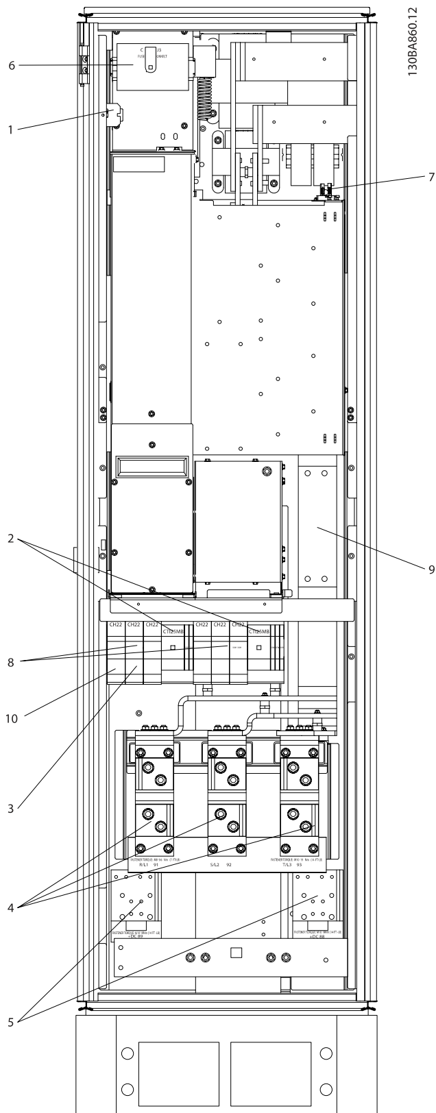
Ilustracja 4.31: Szafka prostownika, rozmiar ramy F17
