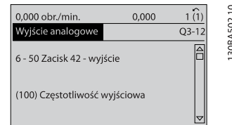
Ilustracja 6.7: Krok 6: Wybrać parametr 6-50 Zacisk 42 . Wyjście . Nacisnąć przycisk [OK].
