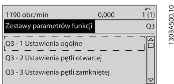
Ilustracja 6.5: Krok 4: Na ekranie pojawią się opcje zestawów parametrów funkcji. Wybrać 03-1 Ustawienia ogólne . Nacisnąć przycisk [OK].
