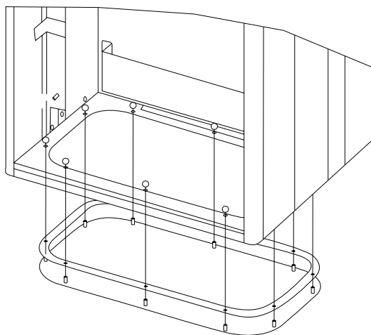
Ilustracja 4.25: Montaż dolnej płyty, E7
