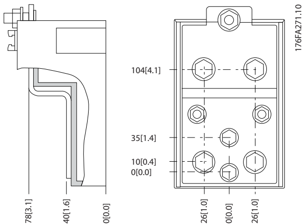
图 3.15 端子特写图
