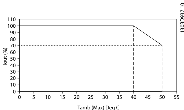
图 8.11 输入/输出与 最高环境温度
