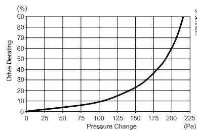
Рисунок 4.23: Корпус F, снижение значений относит. Изменение давления Воздушный поток привода: 580 куб. футов/мин (985 м 3 /час)
