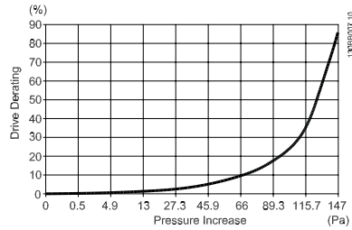
Рисунок 4.20: Корпус D Снижение значений относит. Изменение давления Воздушный поток привода: 450 куб. футов/мин (765 м 3 /час)
