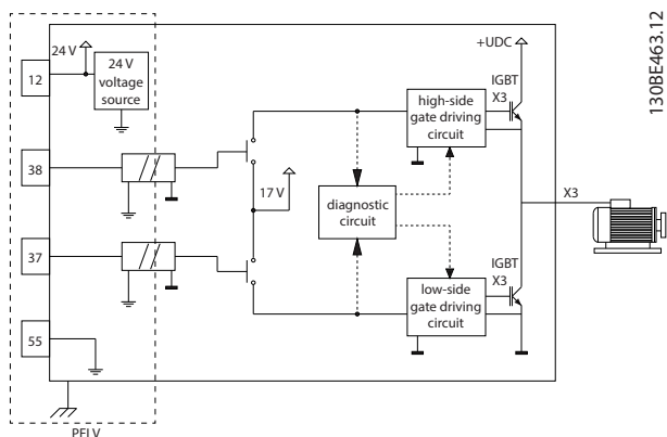
図 6.1 STO アーキテクチャ
