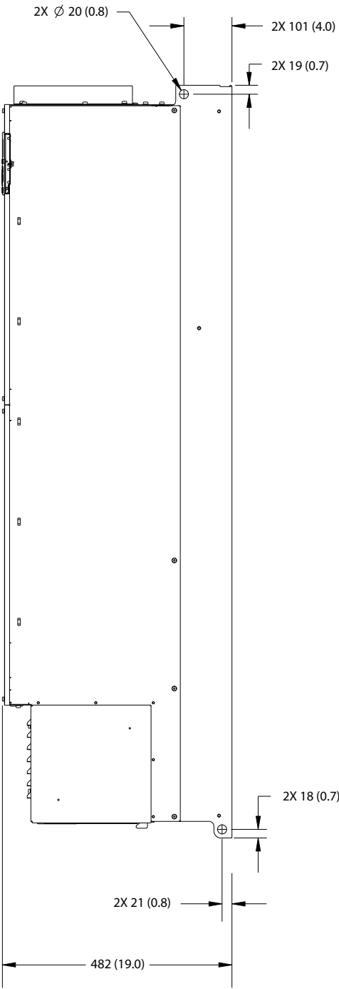
Illustration 62: Vue latérale du boîtier E3h
