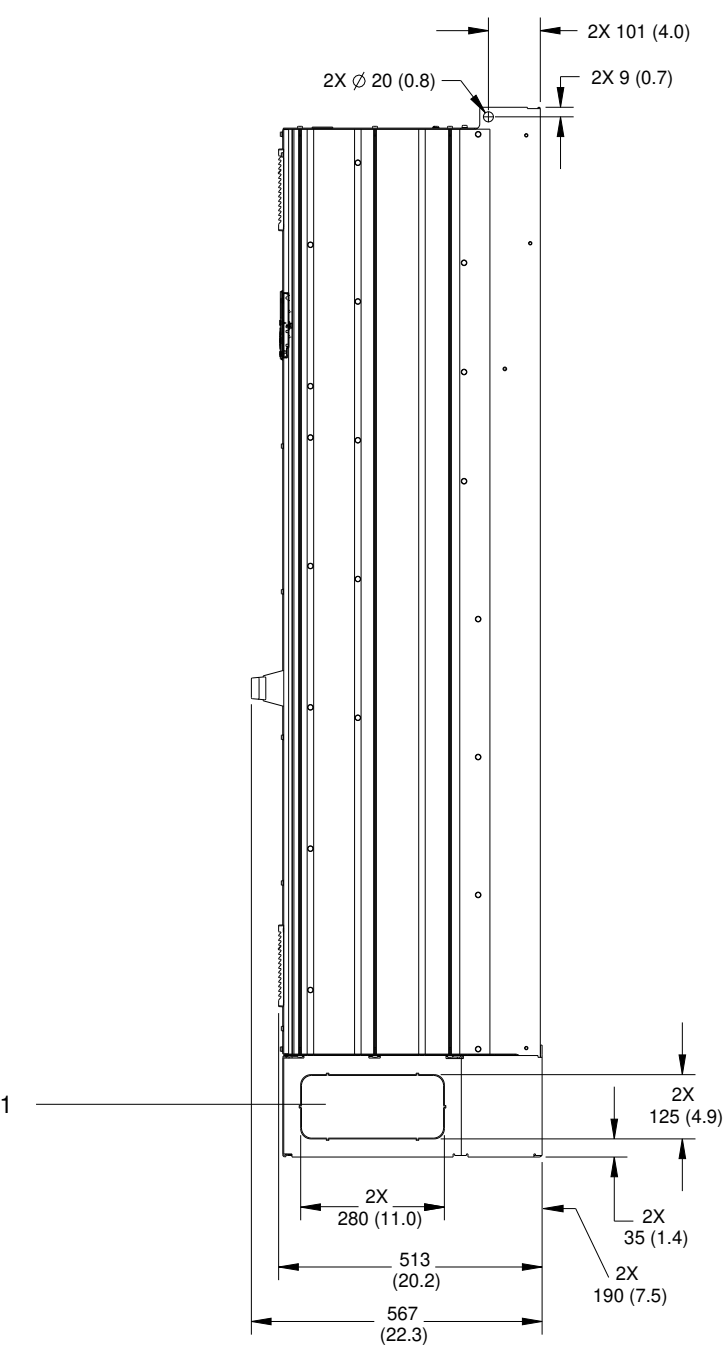
Illustration 58: Vue latérale du boîtier E2h
