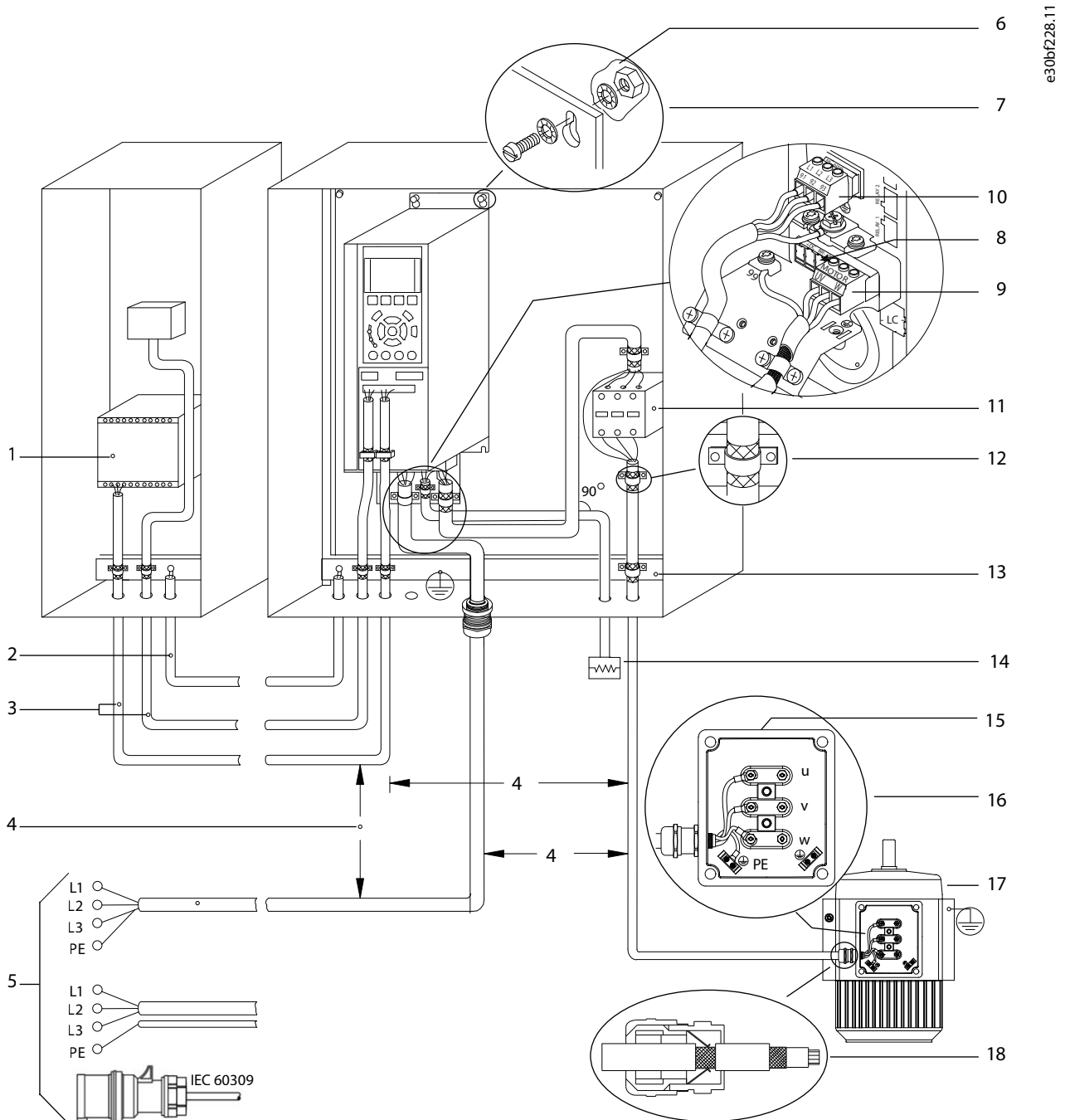
Illustration 17: Exemple d'installation conforme aux exigences CEM
