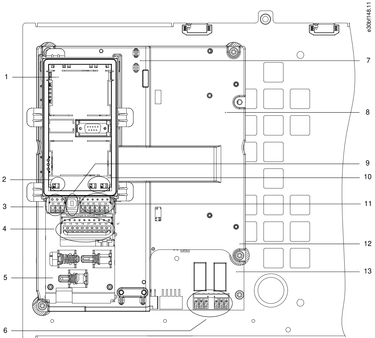
Illustration 4: Vue de la platine de contrôle
