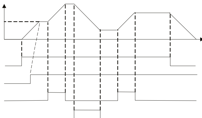
Illustration 41: Accélération/décélération
