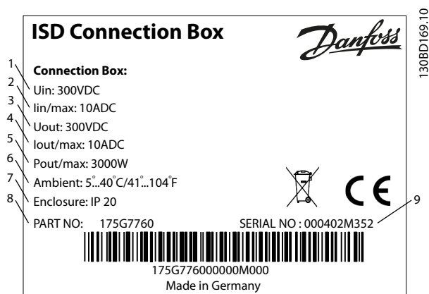
Disegno 11.1 Targhetta
