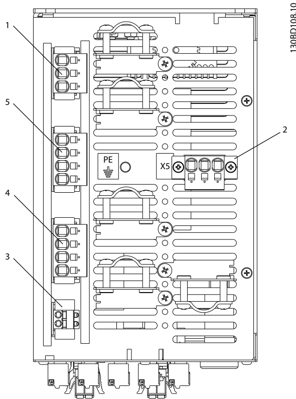
Disegno 4.9 Connessioni sul lato inferiore
