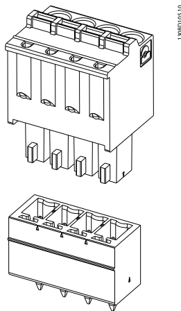
Disegno 4.8 Alloggiamento e spina CAN
