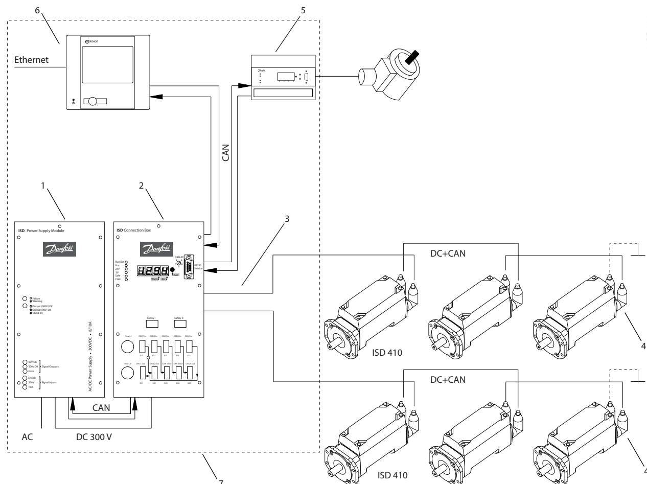
Disegno 4.3 Servosistema ISD con 1 connection box
