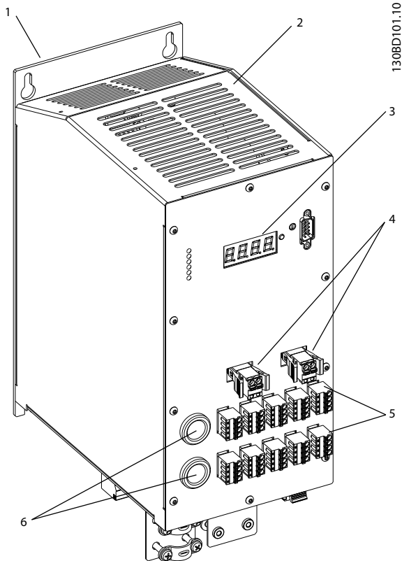
Disegno 4.1 Connection box ISD
