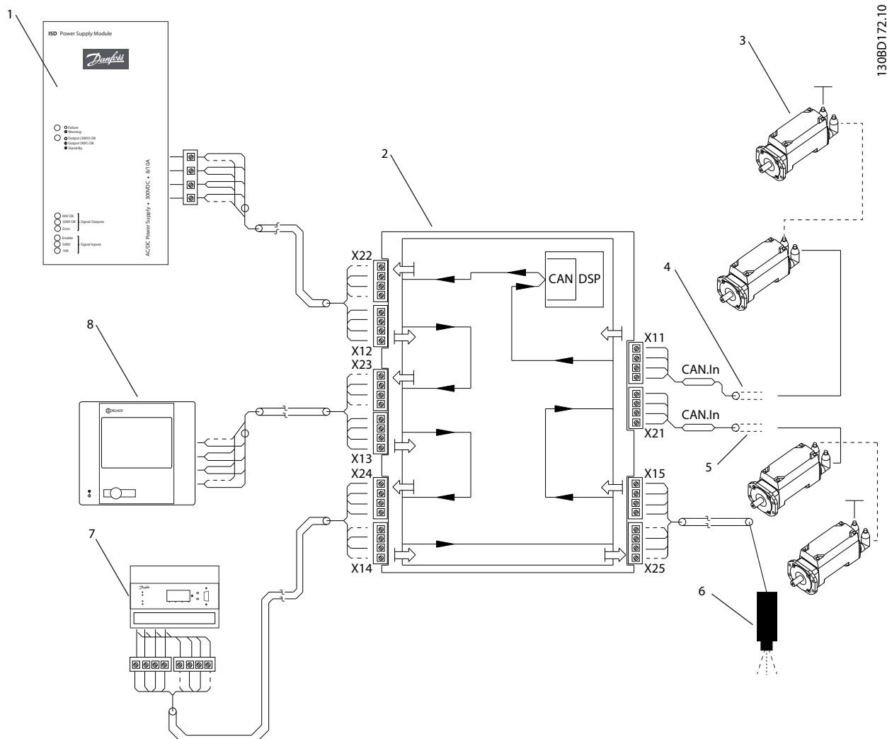
图 5.4 CAN 接线示例 2
