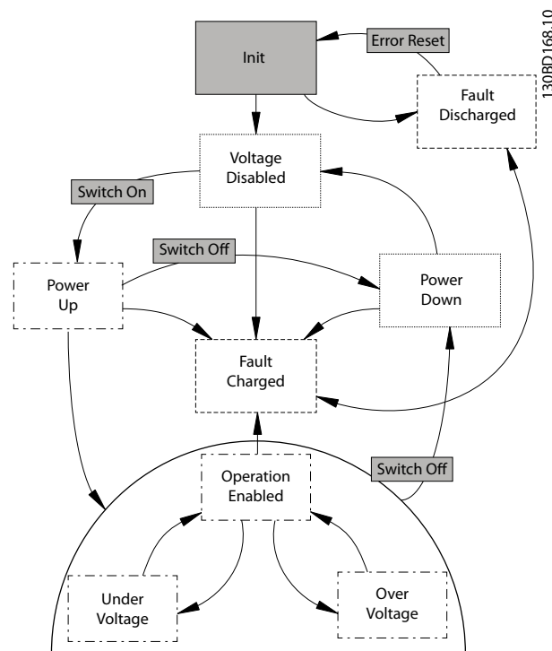
图 7.3 机器状态
