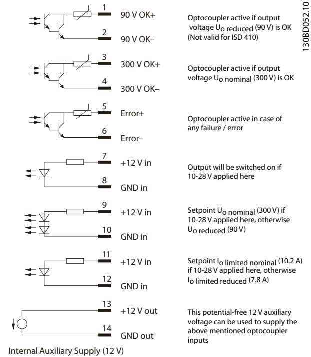
Abbildung 8.5 Signalanschluss X3
