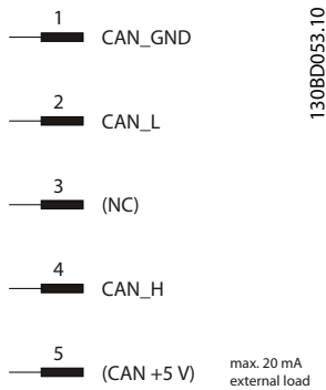
Abbildung 8.6 CAN-Bus-Anschluss X4
