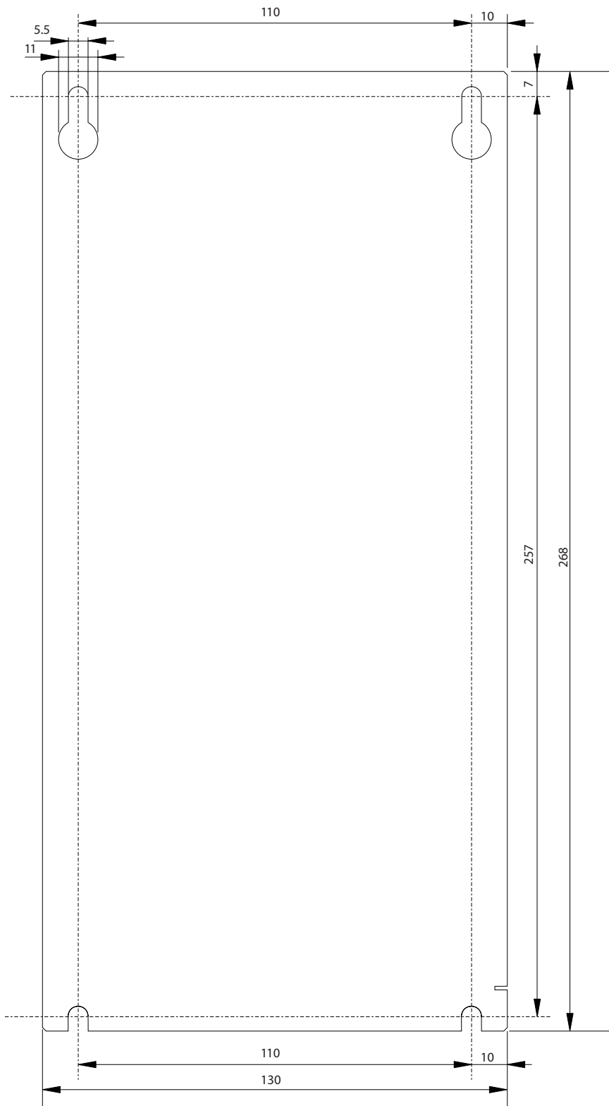
Abbildung 5.1 Abmessungen
