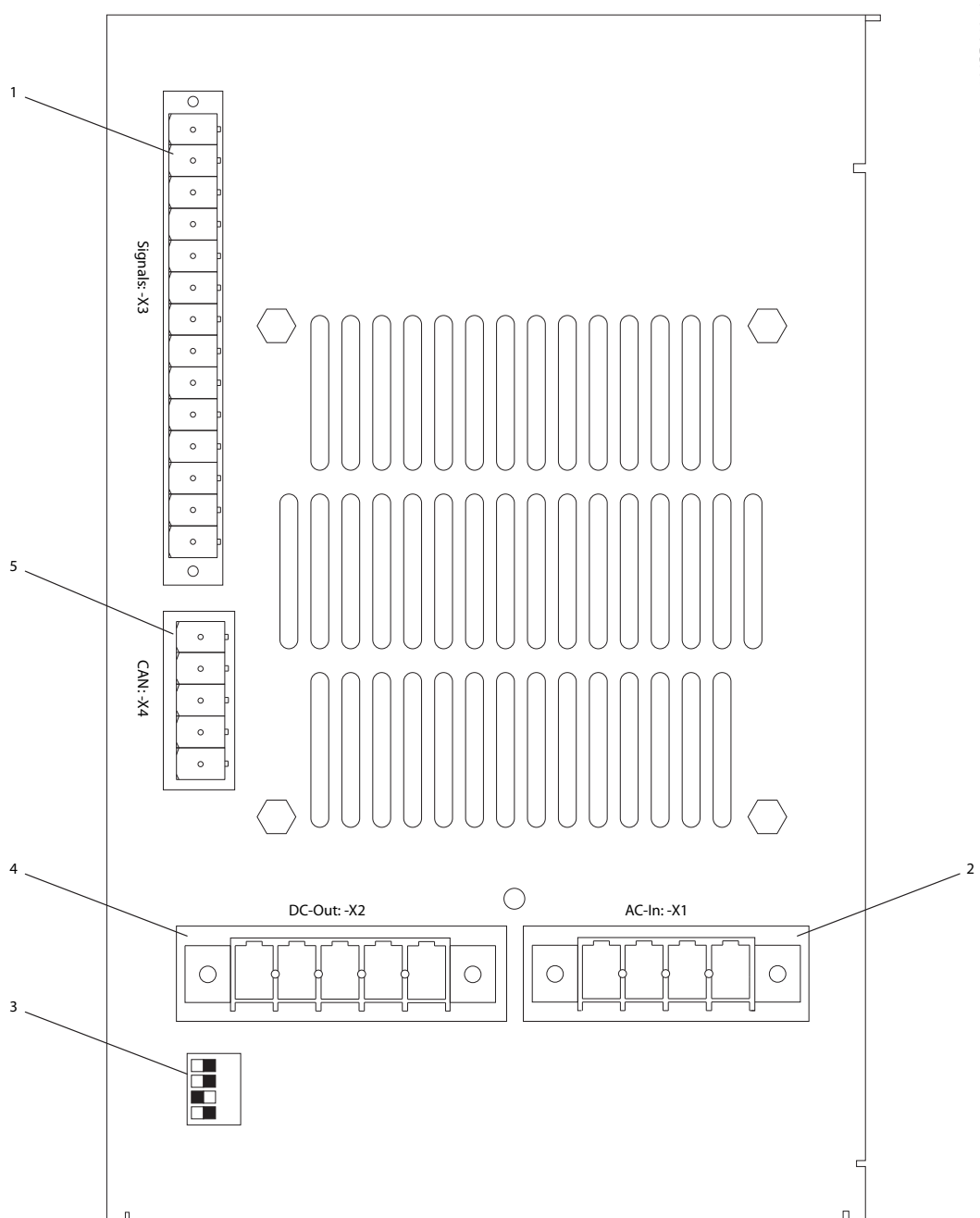
Abbildung 6.1 Anschlüsse
