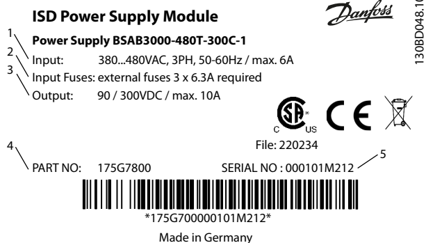
Abbildung 8.1 Typenschild
