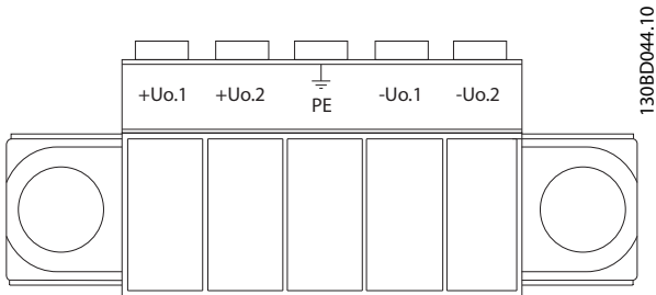
Abbildung 6.3 Netzausgangsstecker
