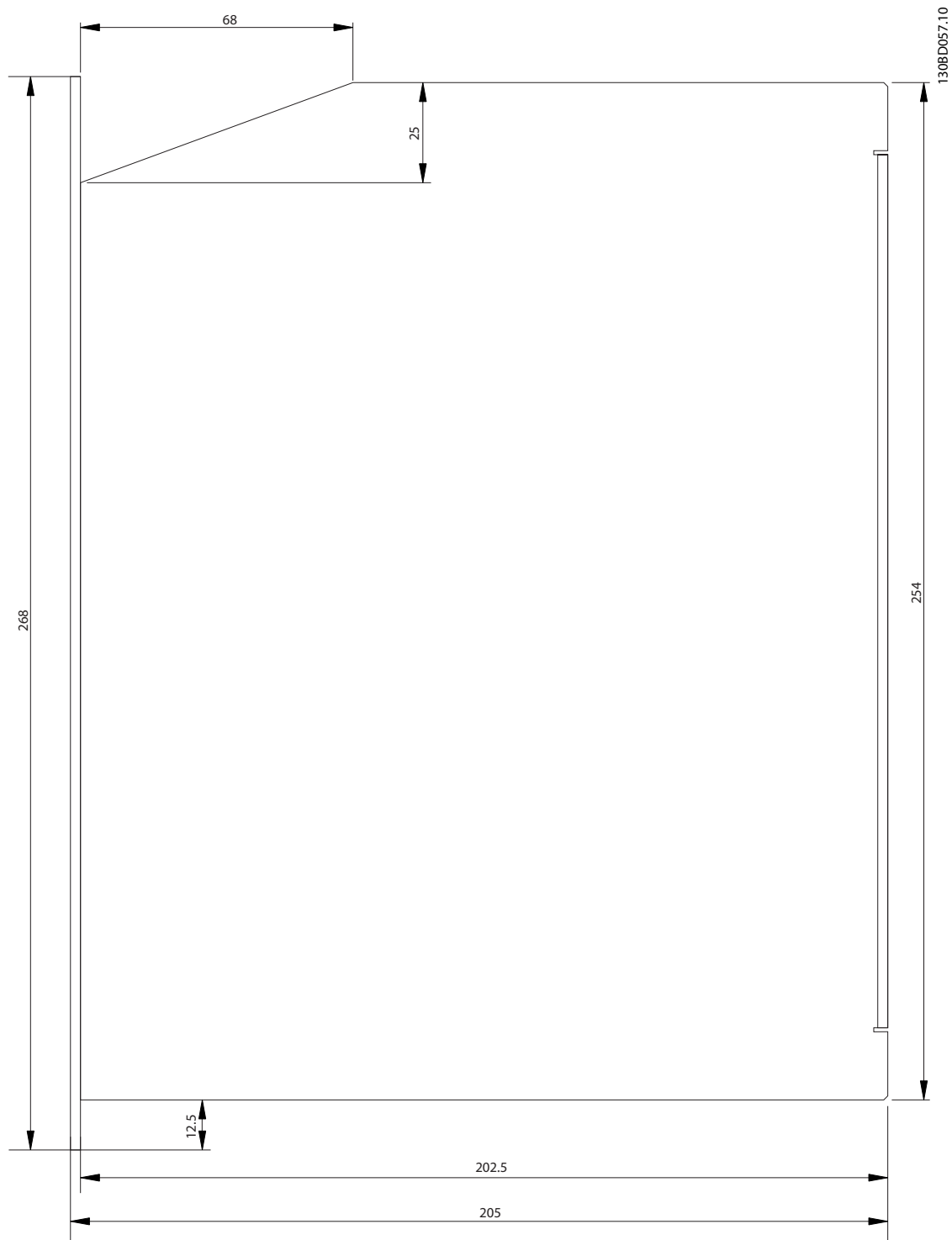
Abbildung 8.9 Seitenansicht
