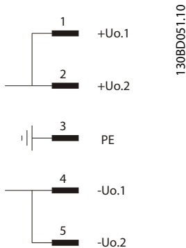
Abbildung 8.4 Eingangsanschluss X2
