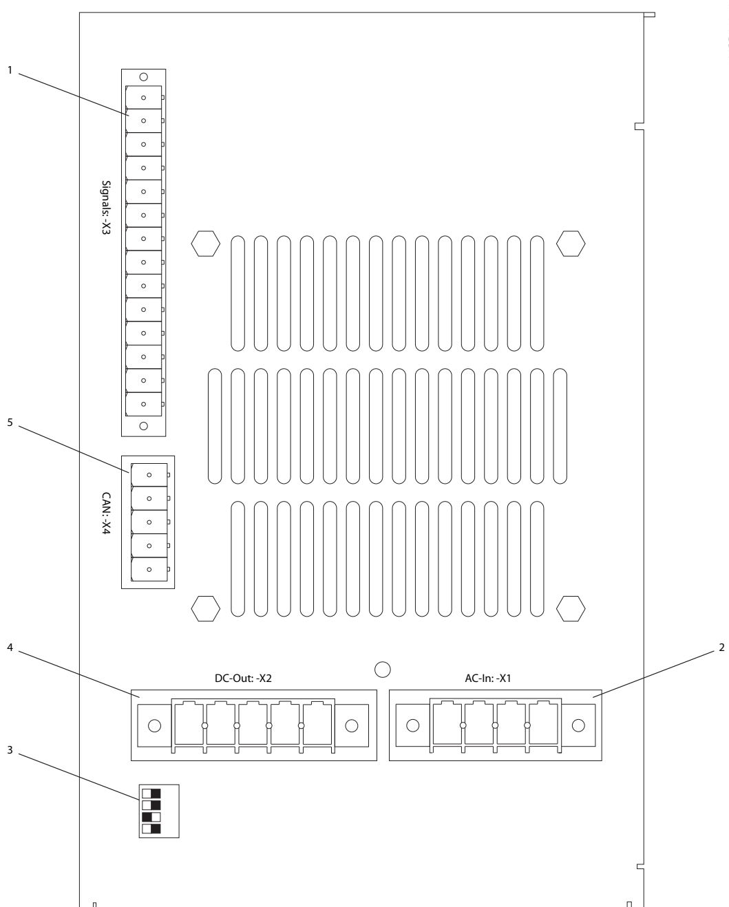
Disegno 6.1 Collegamenti
