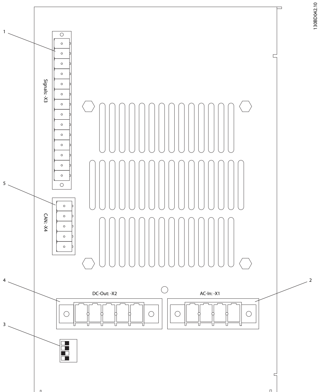
图 6.1 连接
