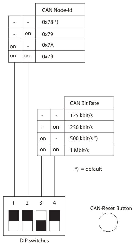
图 8.7 CAN DIP 开关
