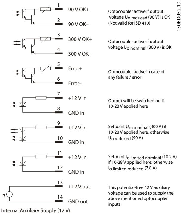
图 8.5 信号连接 X3
