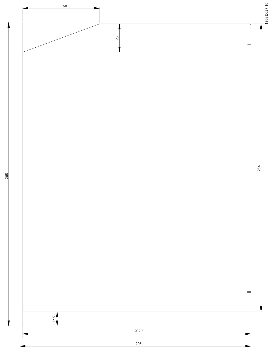
图 8.9 侧视图
