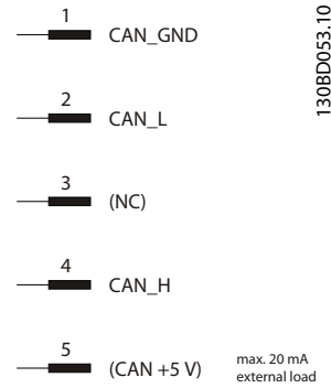
图 8.6 CAN 总线连接 X4
