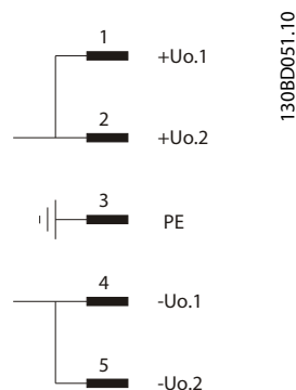
图 8.4 输入连接 X2
