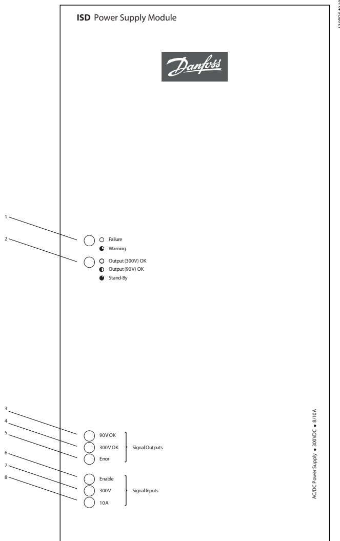
图 8.2 指示灯
