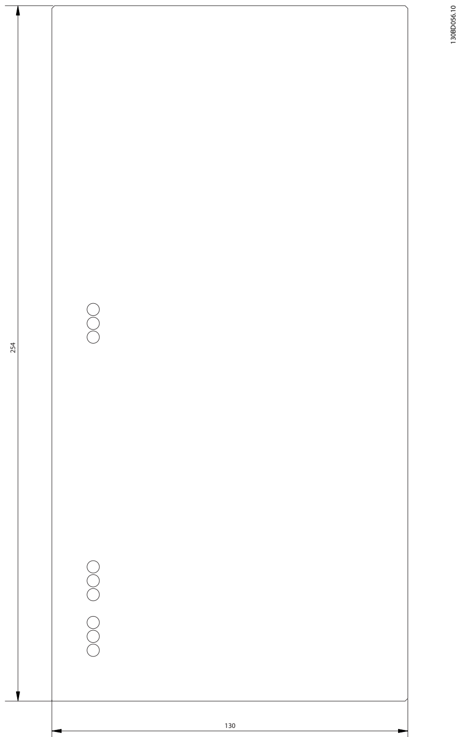
图 8.8 前视图
