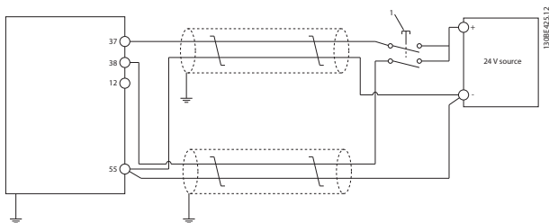
1 Säkerhetsenhet
