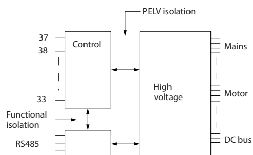
Bild 9.1 Galvanisk isolation
