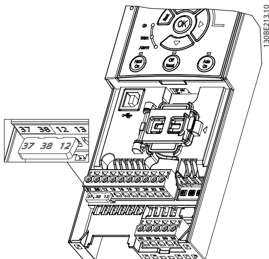
图 6.3 端子 12 (24 V)、37 和 38 之间的跳线
