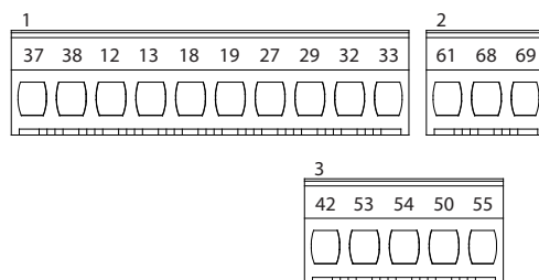
图 4.10 端子号
