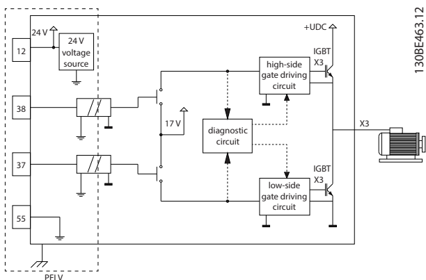
图 6.1 STO 架构
