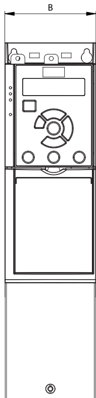
图 9.3 标配底部电缆入口盖（不带顶盖）
