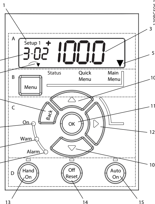
图 5.1 NLCP 视图
