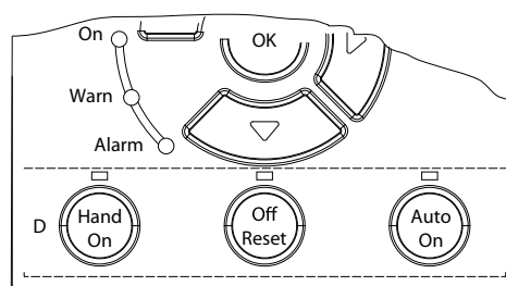
图 8.3 状态指示灯
