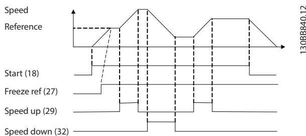
图 7.1 加速/减速
