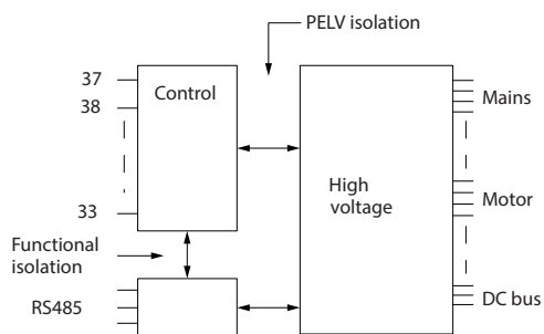
图 9.1 高低压绝缘
