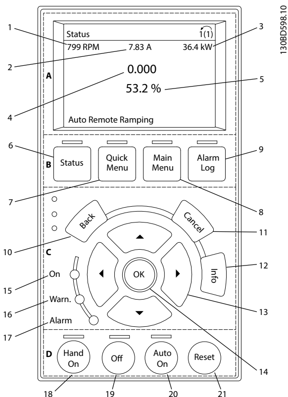
图 5.8 图形化本地控制面板 (GLCP)
