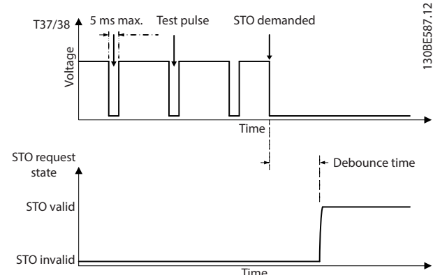
圖 6.2 測試脈衝濾波
