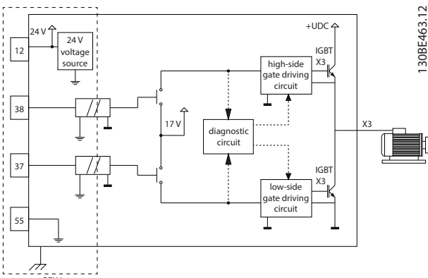
圖 6.1 STO 架構
