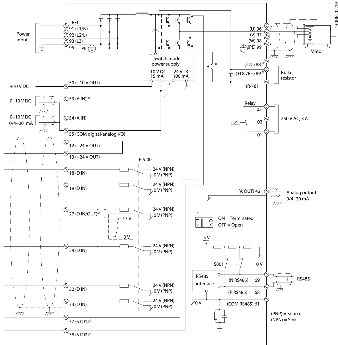
圖 4.2 基本配線概要圖表
