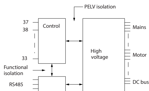
圖 9.1 電氣絕緣
