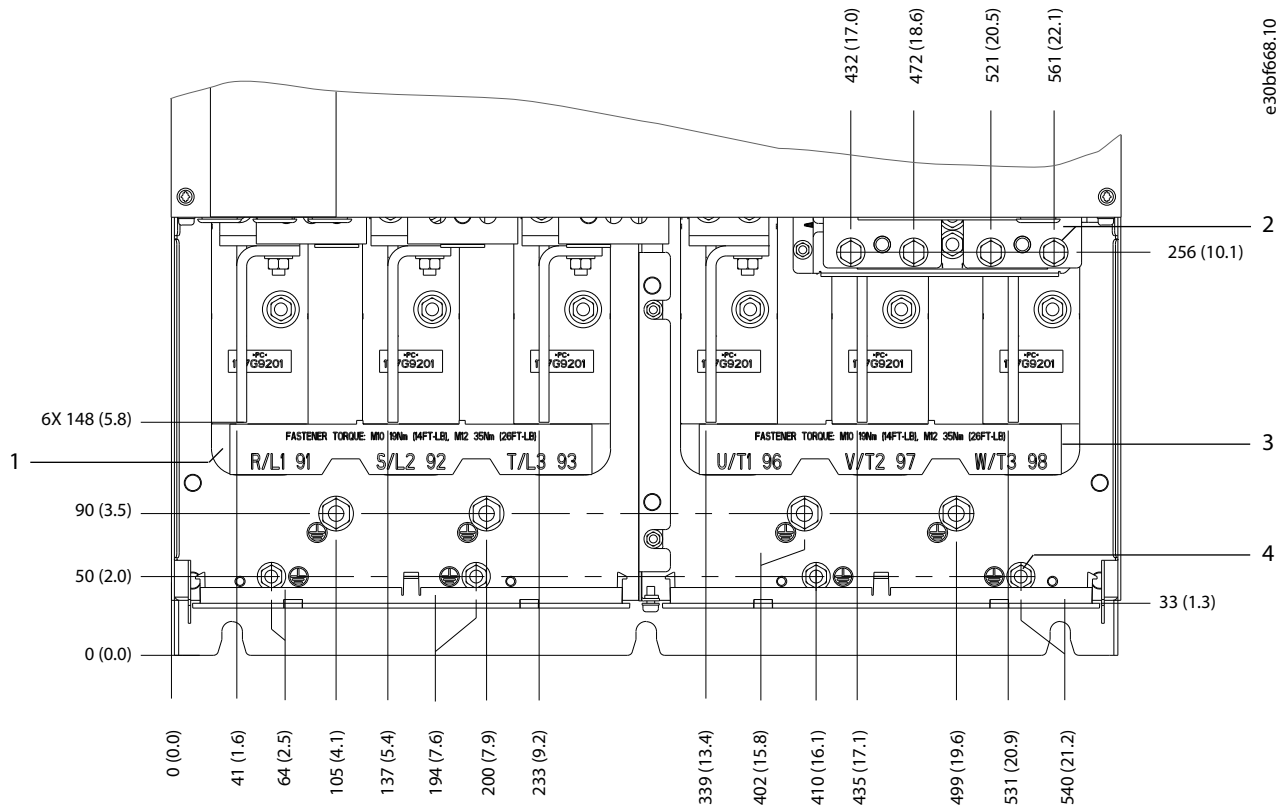
Ilustração 29: Dimensões dos terminais do E4h (vista frontal)
