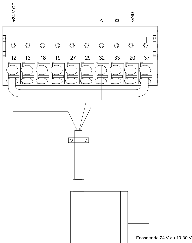
Ilustração 46: Configuração dos fios para o encoder
