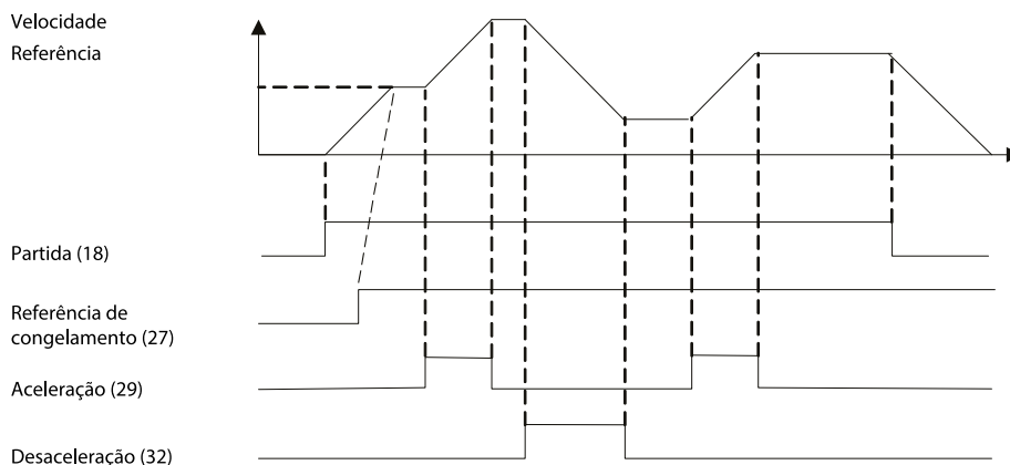
Ilustração 41: Aceleração/Desaceleração
