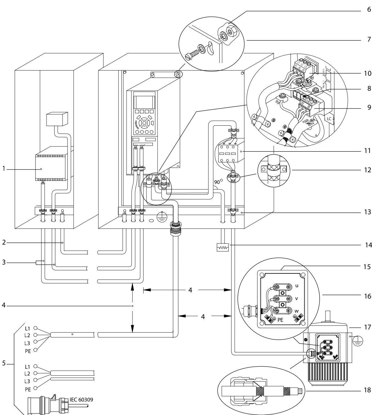
Ilustração 17: Exemplo de instalação de EMC correta
