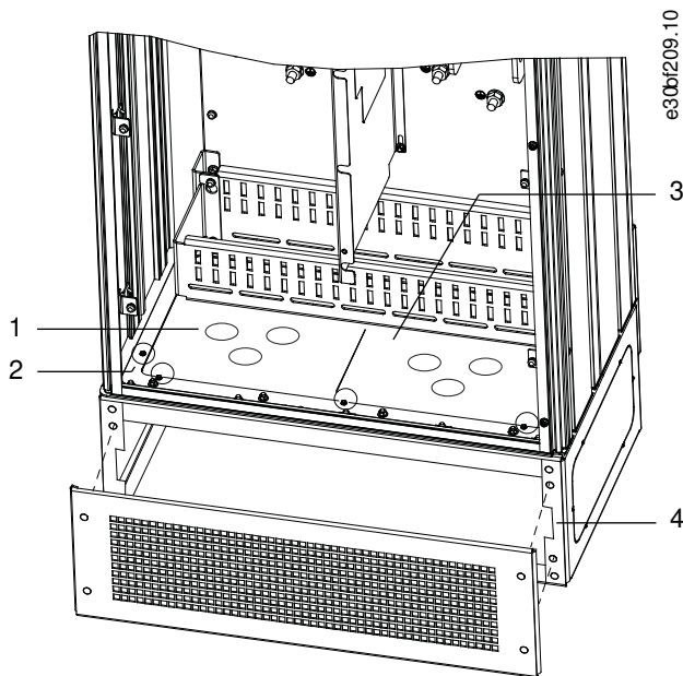
Ilustração 13: Instalação da placa de entrada de cabos
