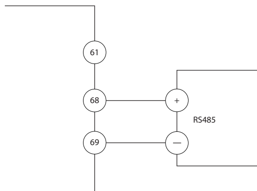
Kuva 4.12 Sarjaliikenteen kytkentäkaavio
