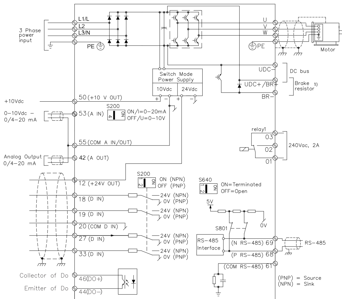
图 1.7 图中显示了所有电气端子
