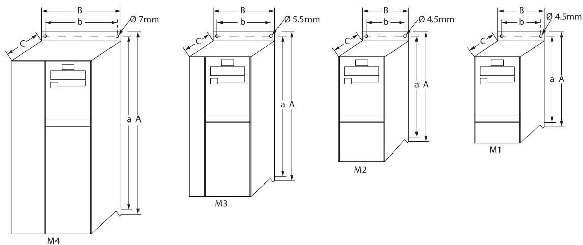
图 1.1 机械尺寸
