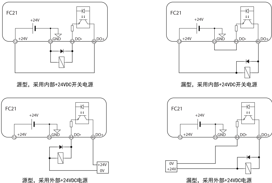
图 1.6 DO 接线图
