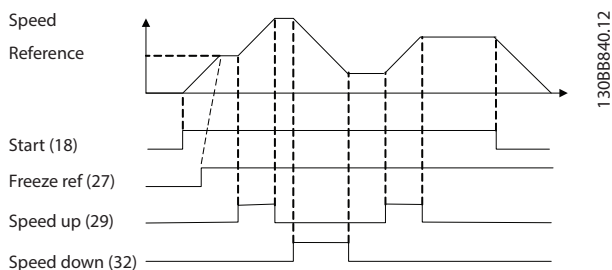
Obrázek 7.1 Zrychlení/zpomalení
