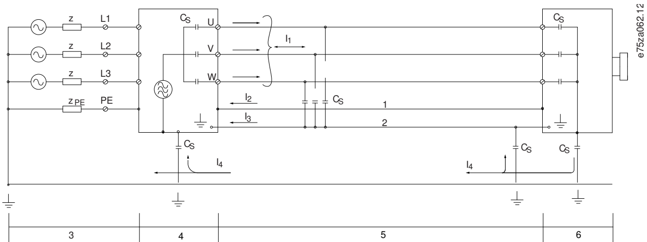
图解 22: 漏电流的产生
