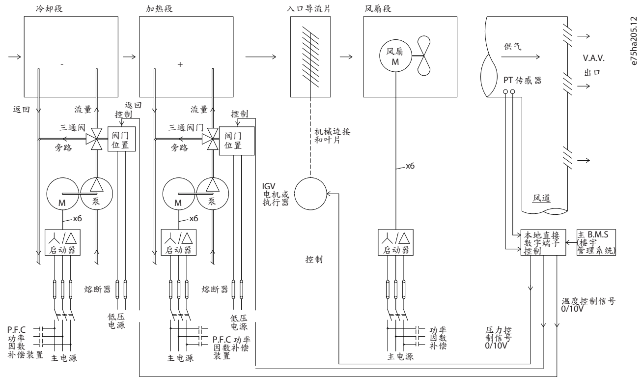
图解 9: 无变频器的传统风扇系统
