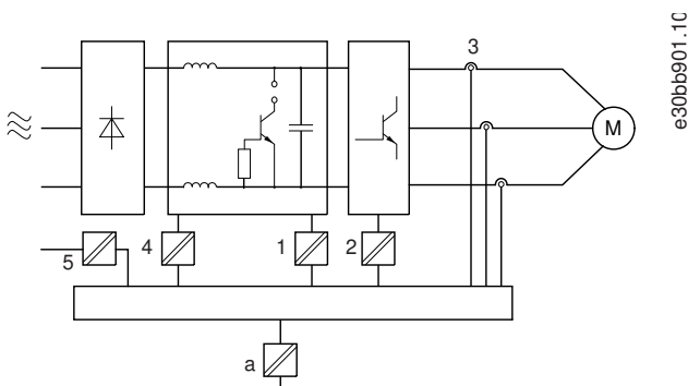
图解 25: 电气隔离 30 - 90 kW (40 - 120 hp)
