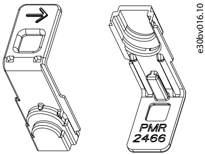
图解 38: 保护罩
