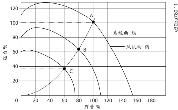
图解 1: 降低风扇流量时的风扇曲线 (A、B 和 C)
