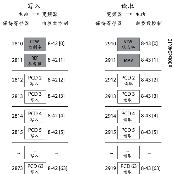
图解 73: 通过 PCD 读/写访问
