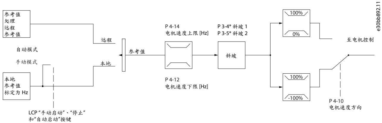
图解 17: 开环结构
