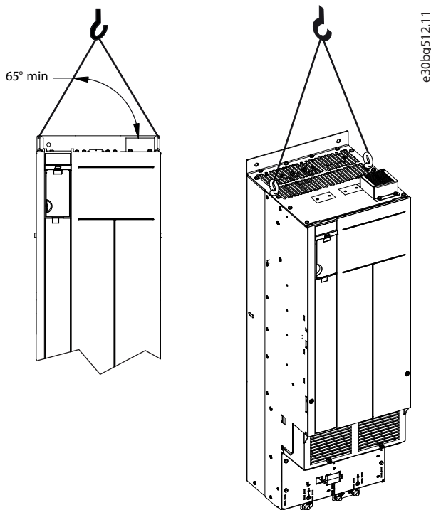
图解 41: 提升变频器
