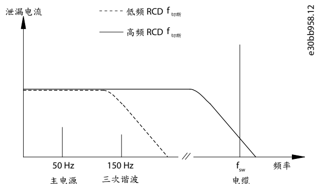
图解 29：主电源造成泄漏电流
