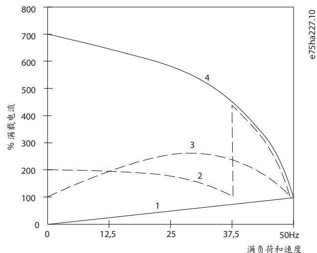
图解 8: 启动电流
