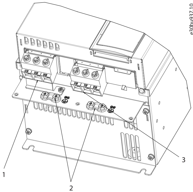
图解 47: 机箱规格 H11、IP20、380-480 V、30-45 kW (40-60 hp)
