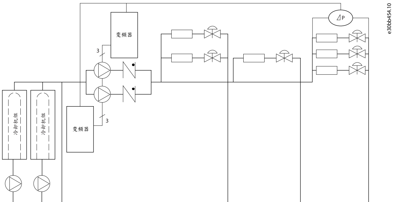
图解 16: 辅助泵
