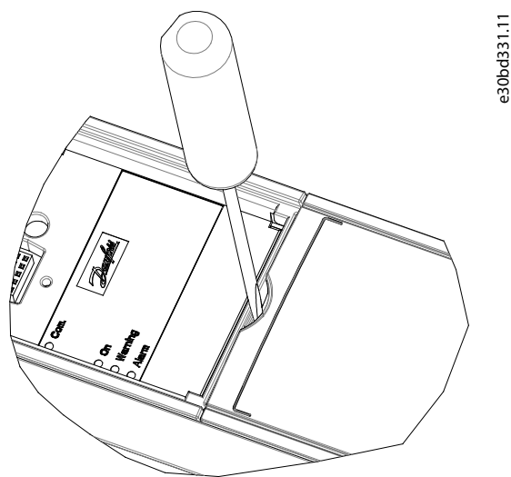
图解 55: 拆下端子盖
