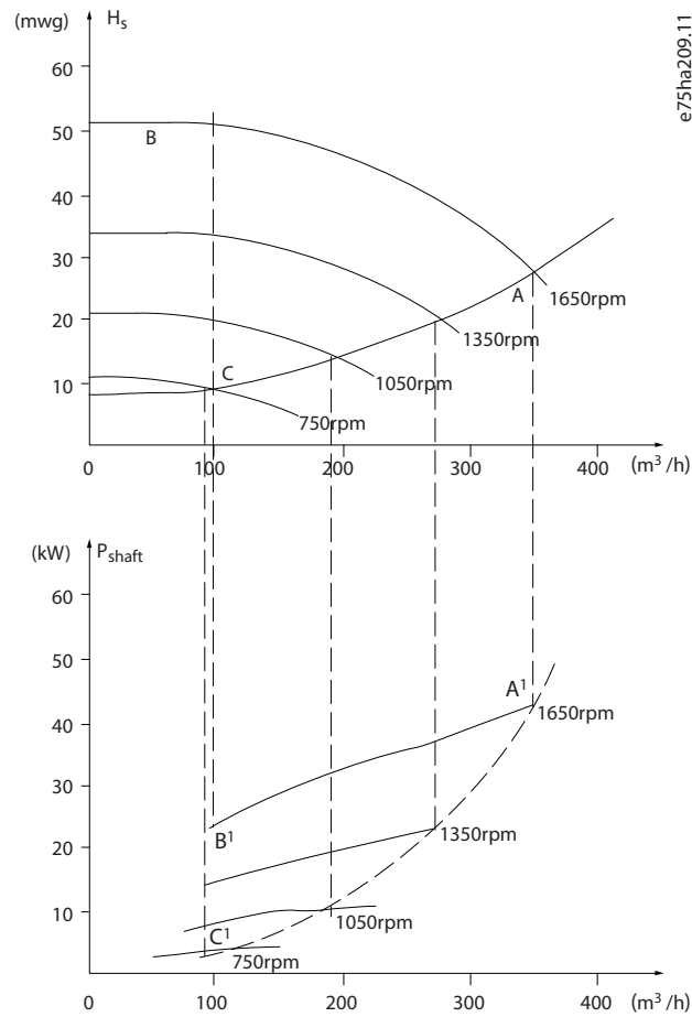
图解 7: 能量
