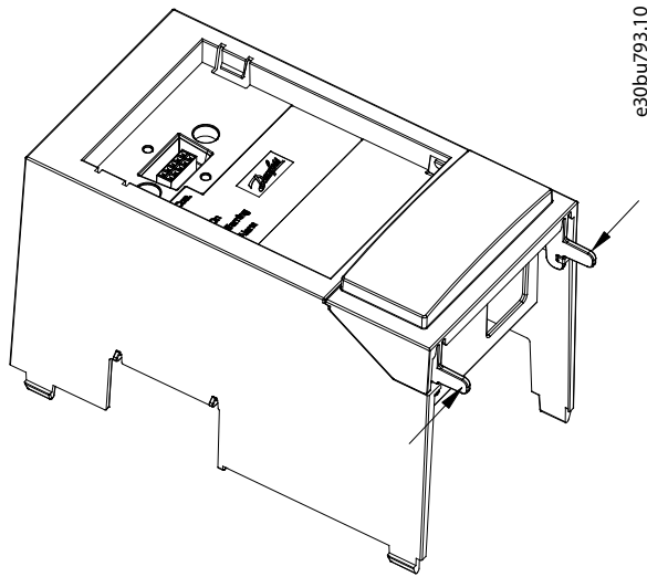
图解 56: 拆除托架盖
