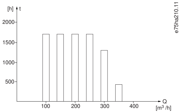
图解 6: 一年的流量分布
