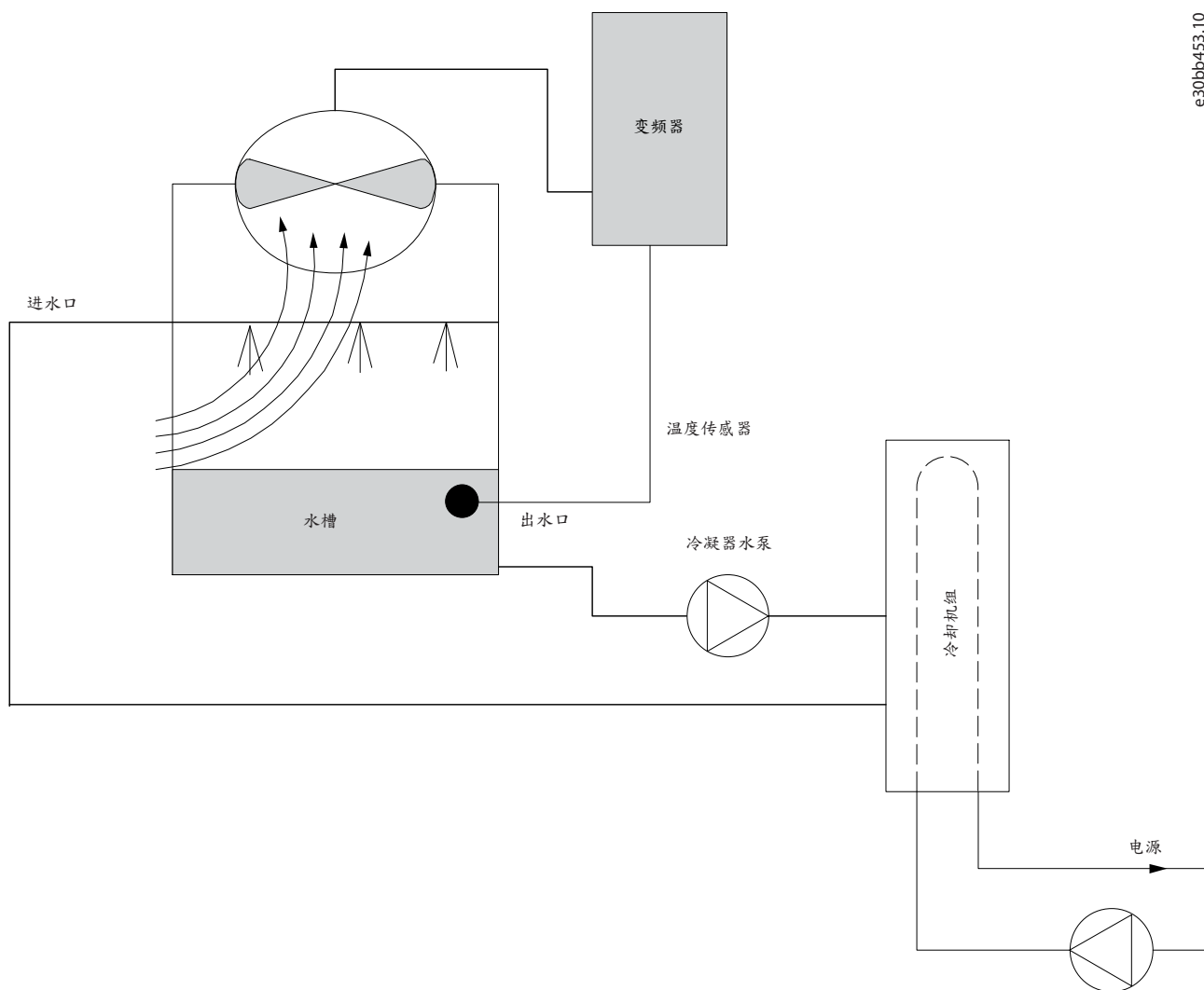
图解 13: 冷却塔风扇
