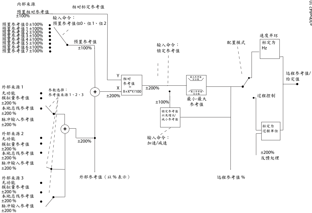
图解 21: 框图显示了远程参考值
