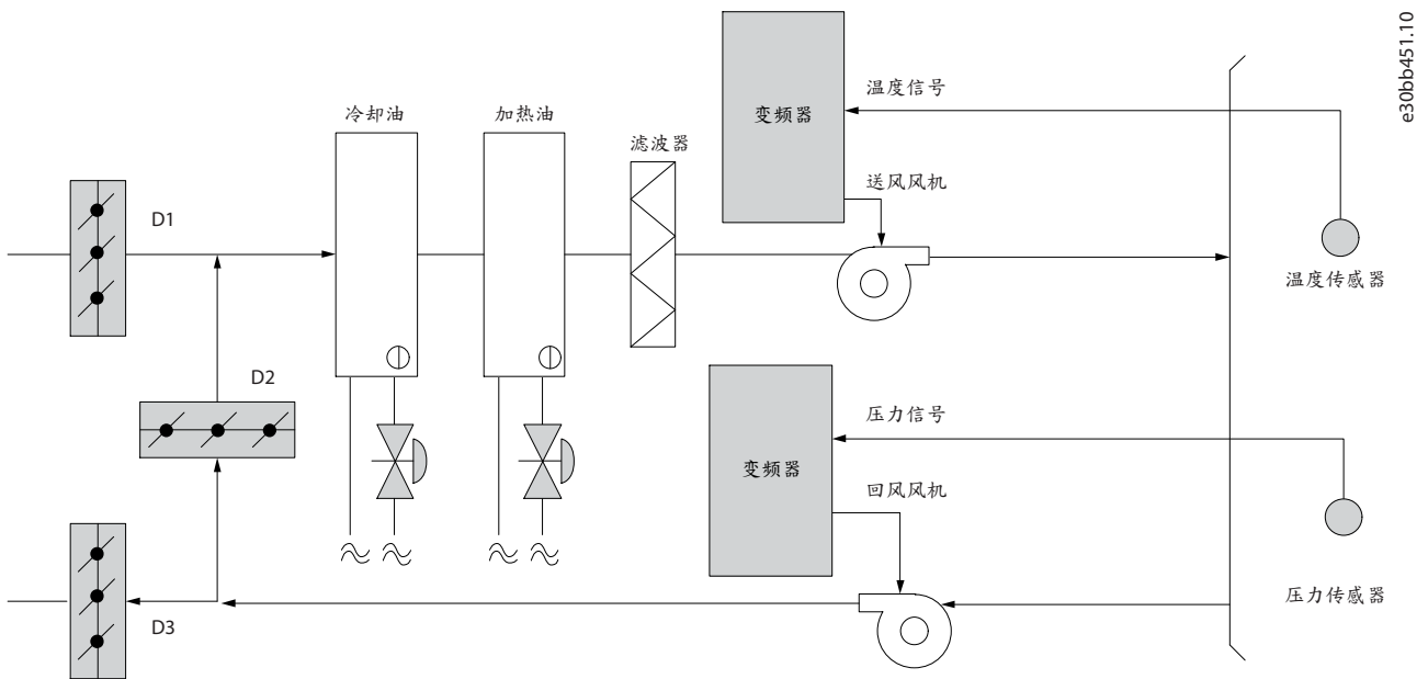
图解 12: 定风量
