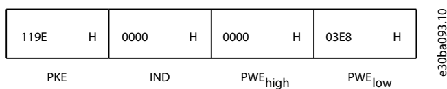
图解 70: 主站响应
