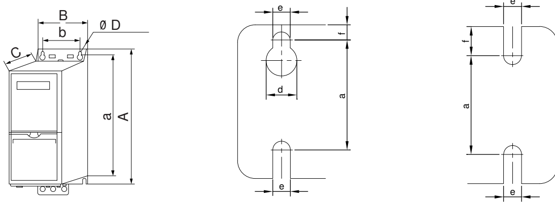
图解 37: 机箱规格为 H1-H5 和 H11-H12 的变频器的尺寸
