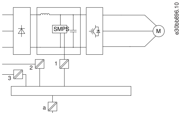
图解 24: 电气隔离 0.37 - 22 kW (0.5 - 30 hp)
