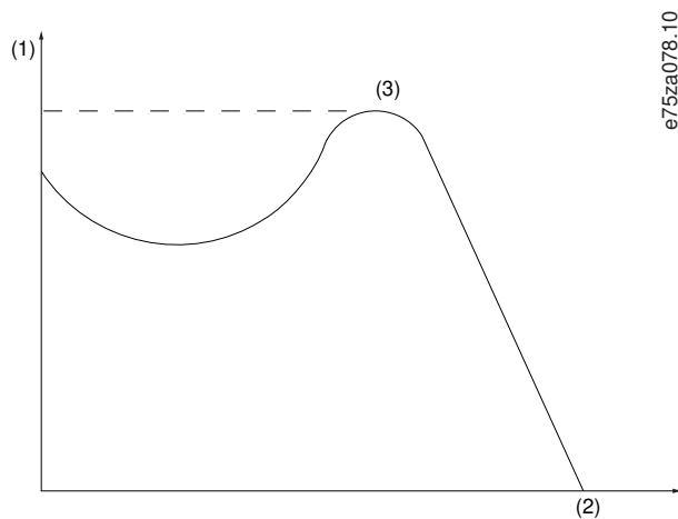
图解 78：起步转矩
