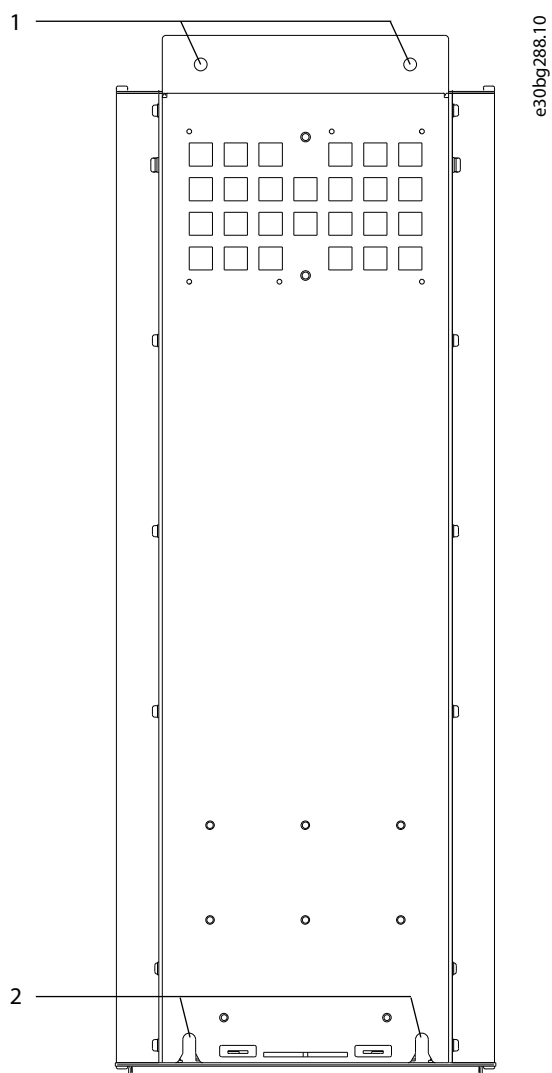
图解 42: 变频器壁装孔
