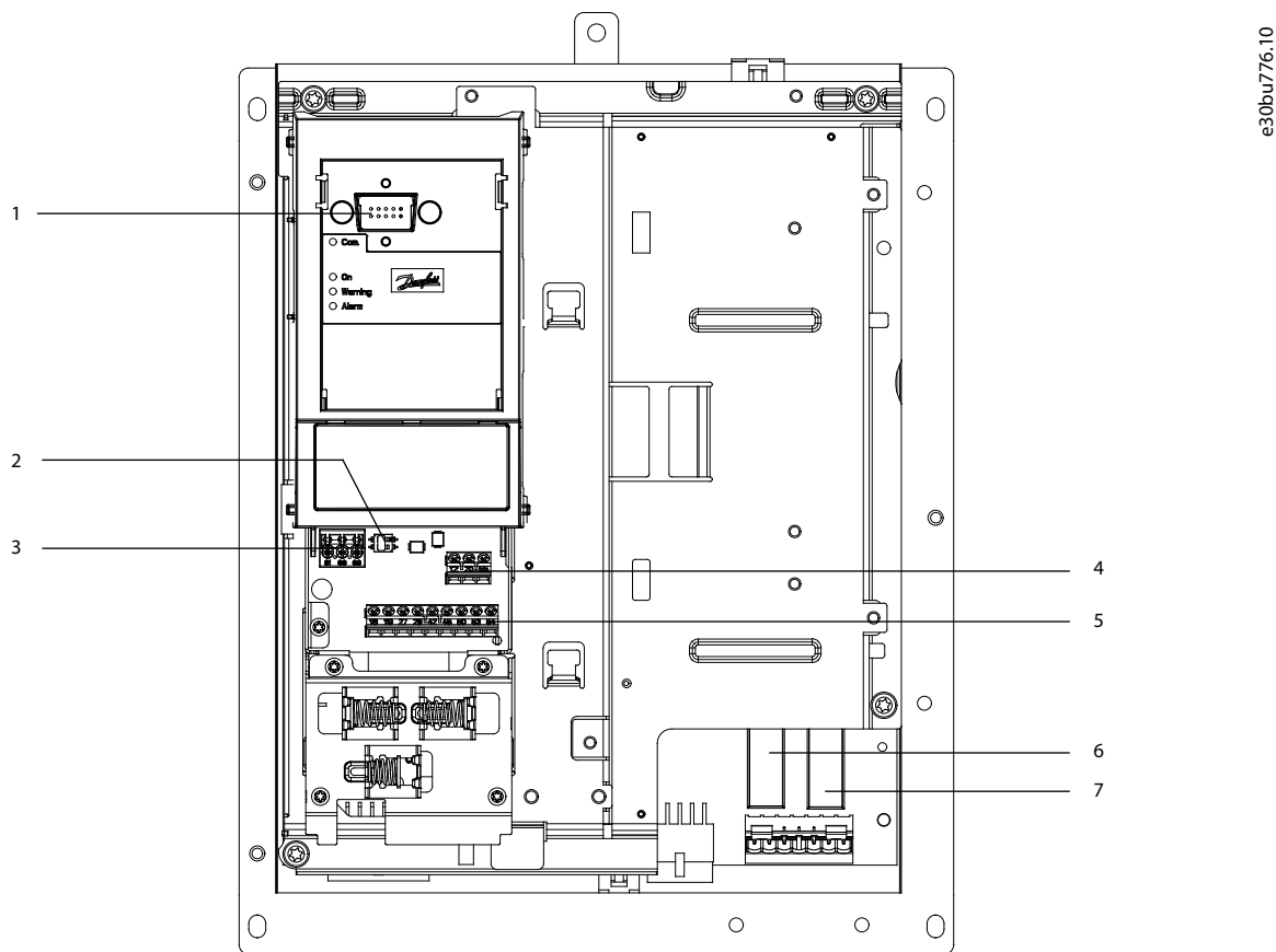
图解 51: H13-H14 中的支架视图
