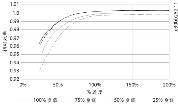
图解 58: 典型效率曲线
