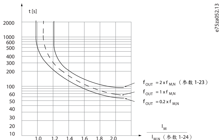
图解 31: 电机热保护特性
