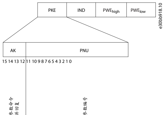
图解 68: PKE 字段
