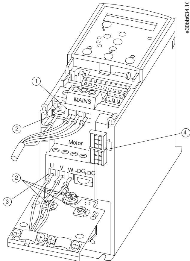
图解 46: 机箱规格 H1 - H5 IP20, 380 - 480 V, 0.37-22 kW (0.5-30 hp)
