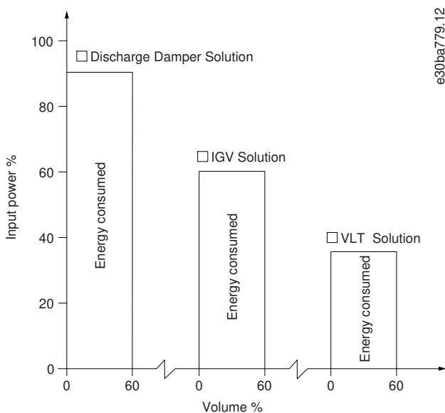
图解 5: 节能
