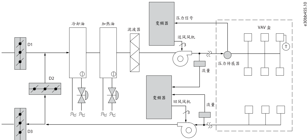
图解 11: 变风量
