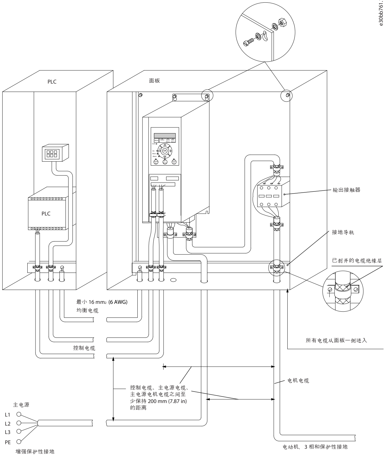
图解 45: 符合 EMC 规范的安装
