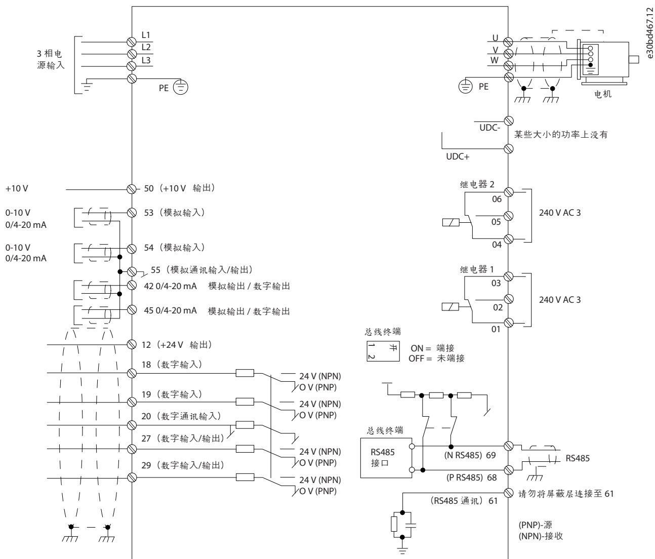
图解 44: 基本接线示意图
