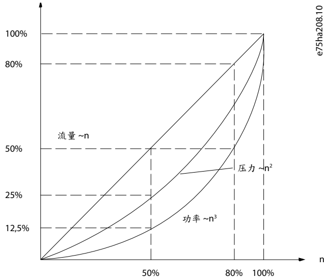
图解 3: 比例法则
