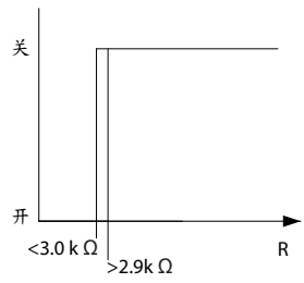
图解 34: 模拟输入/10 V 电源
