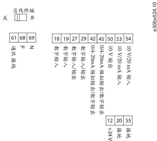
图解 57: 控制端子
