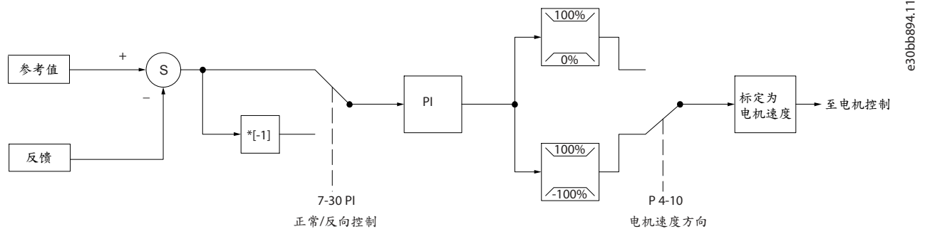
图解 19: 闭环控制结构
