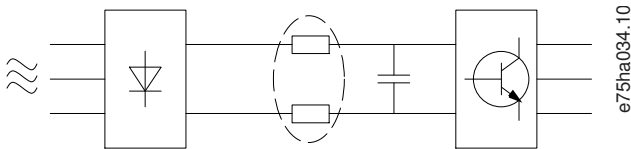
图解 23: 直流回路电抗
