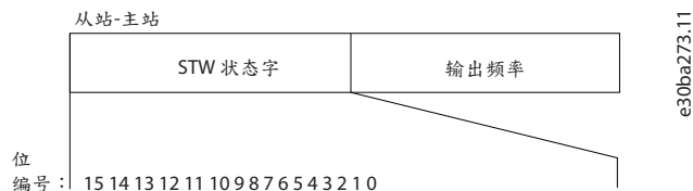
图解 75: 状态字
