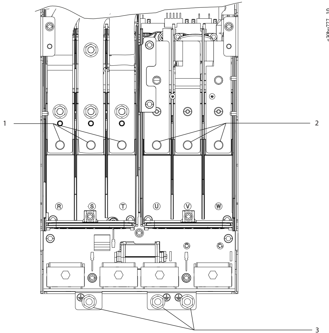
图解 49: 机箱规格 H13 - H14 IP20, 380 - 480 V, 110-315 kW (150-450 hp)
