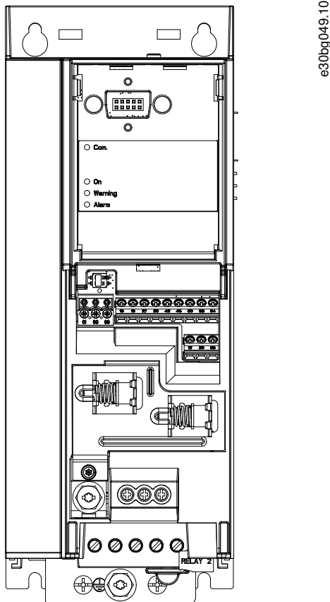
图解 61: 终端电阻拨码开关的出厂设置
