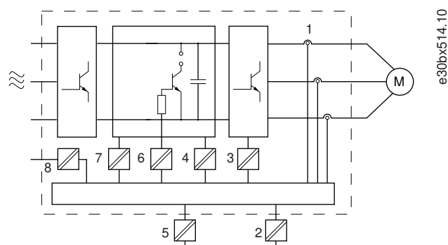
图解 26: 电气隔离 110-315 kW (150-450 hp)
