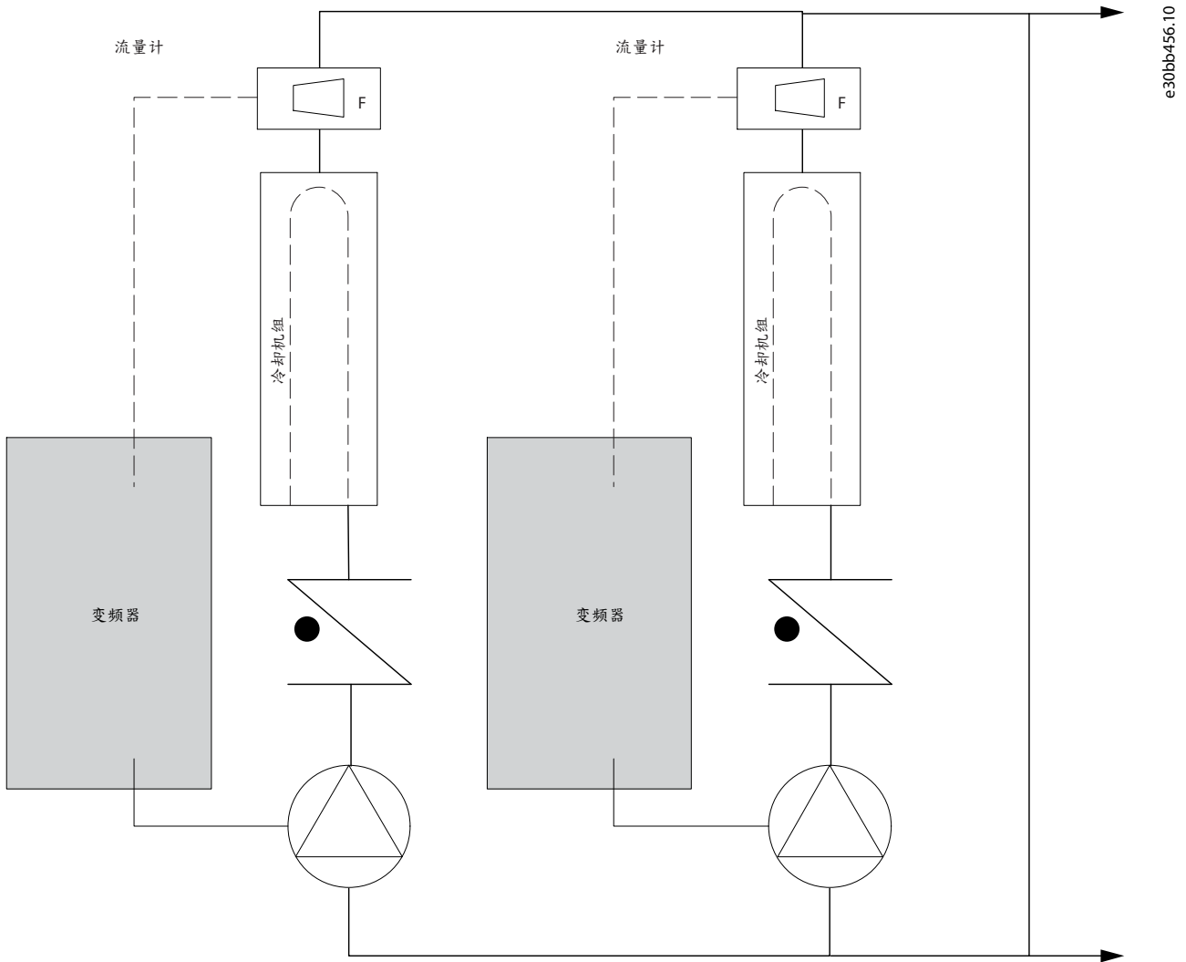
图解 15: 主泵
