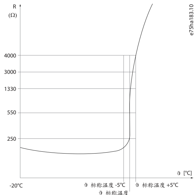
图解 32: 电机温度过高时, 变频器将跳闸
