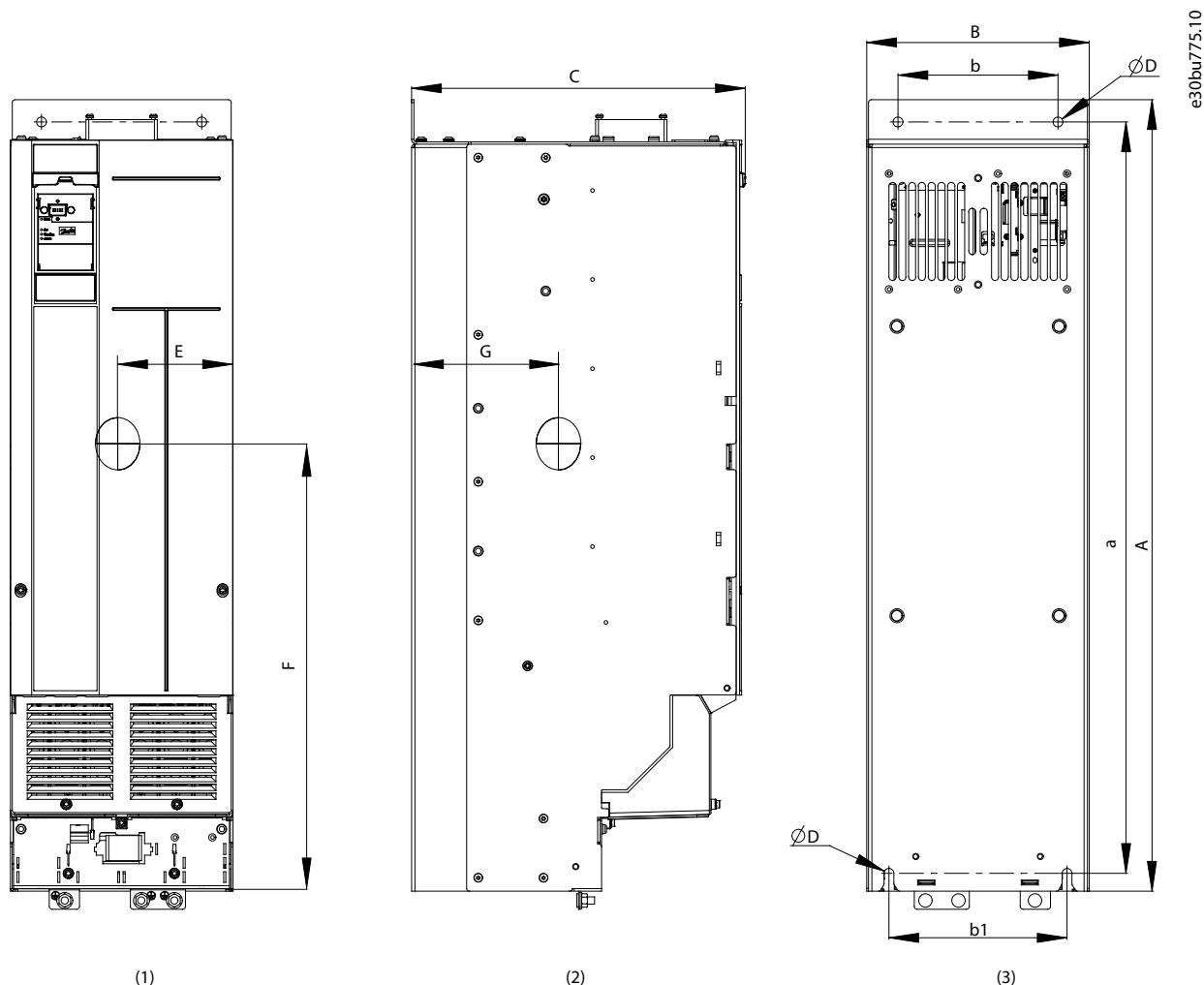
图解 40: 机箱规格为 H13-H14 的变频器的尺寸
