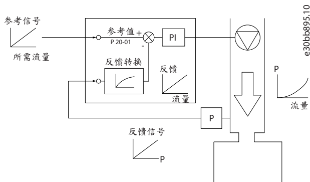
图解 20: 反馈信号转换
