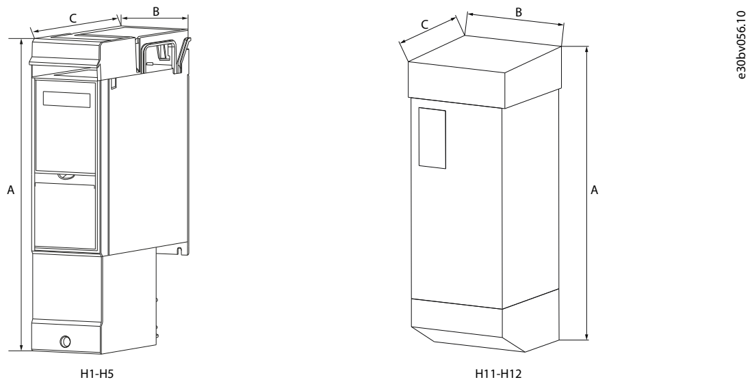
图解 39: 机箱规格为 H1-H5 和 H11-H12 且带 IP21/ 类型 1 转换套件的变频器的尺寸
