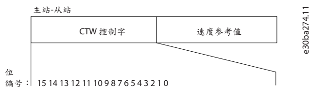
图解 74: 与 FC 协议对应的控制字
