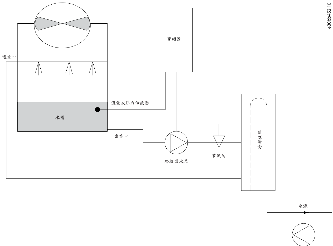
图解 14: 冷凝器泵
