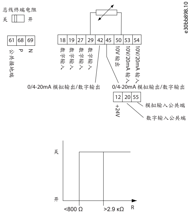
图解 33: 数字输入/10 V 电源
