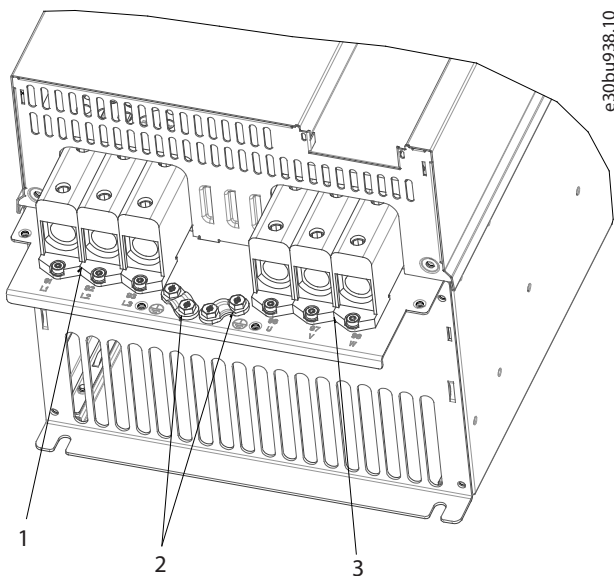
图解 48: 机箱规格 H12、IP20、380-480 V、55-90 kW (75-125 hp)
