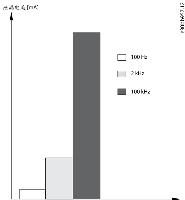
图解 30: RCD 的截止频率对做出的响应/执行的测量的影响
