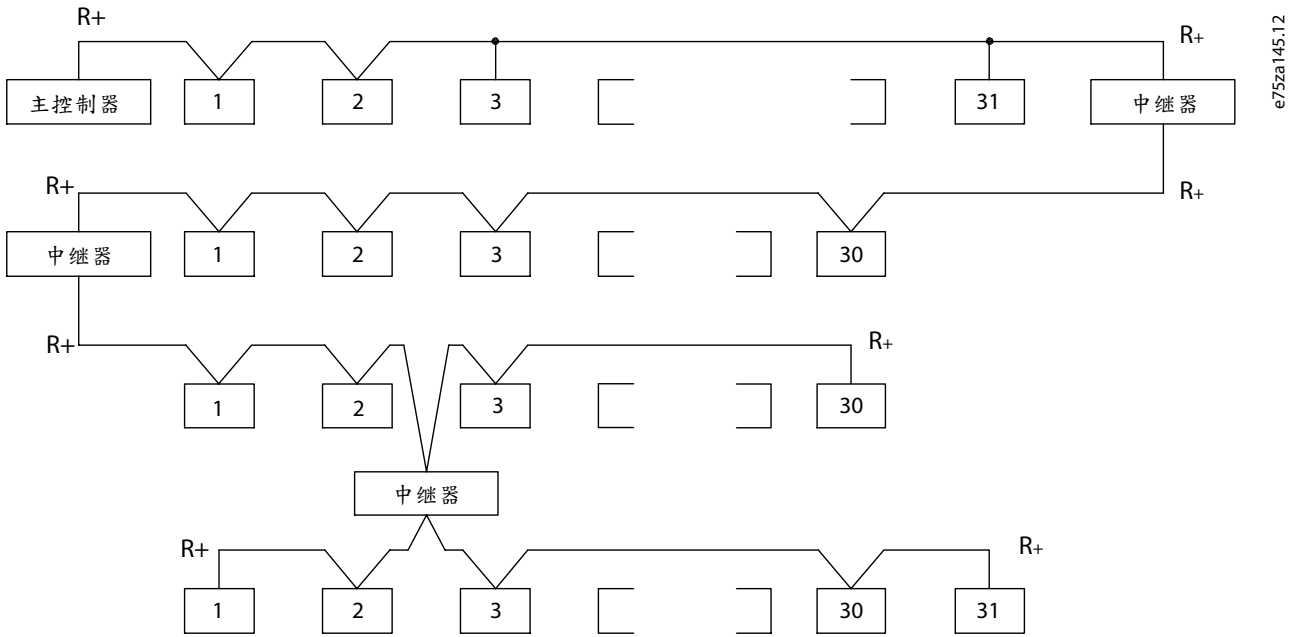
图解 59: RS 485 总线接口
