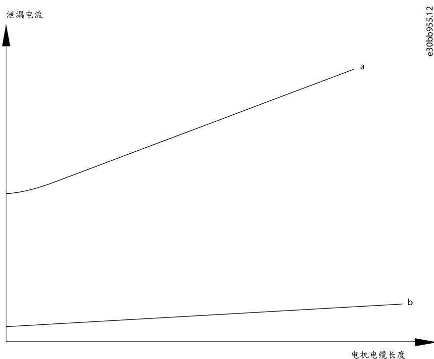
图解 27: 电缆长度和功率规格对泄漏电流的影响, 功率规格 a > 功率规格 B
