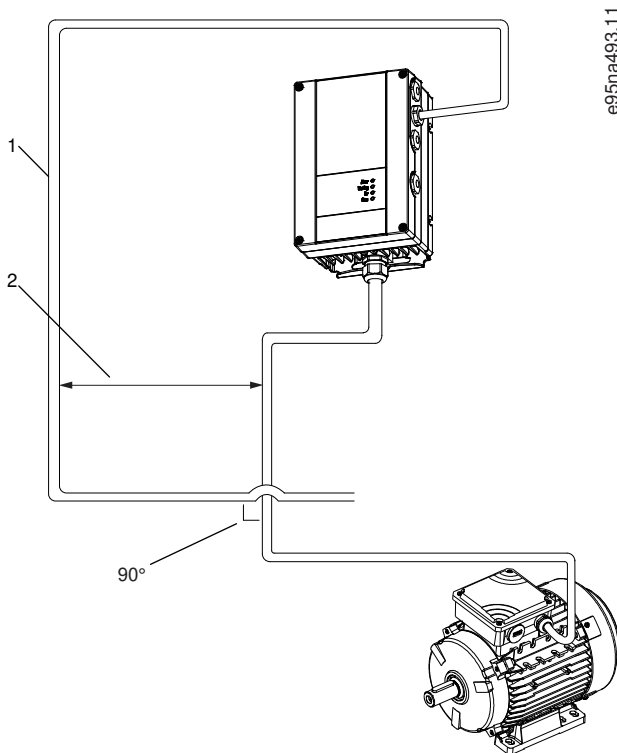
图解 62: 通信电缆与电源电缆之间的最短距离
