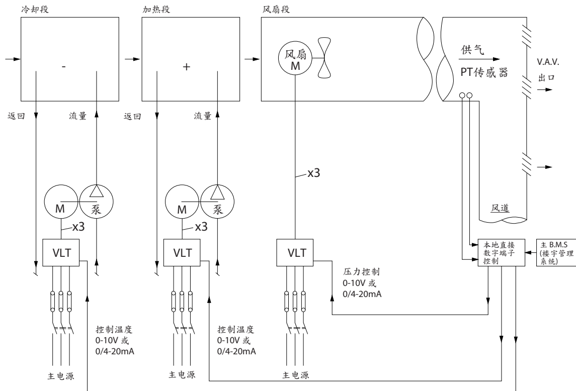
图解 10: 由变频器控制的鼓风机系统
