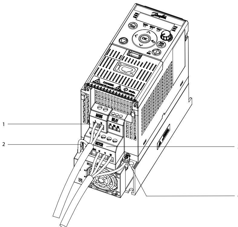
Рисунок 37: Подключение сетевого питания, двигателя и заземления на однофазных блоках (на примере MA02c)
