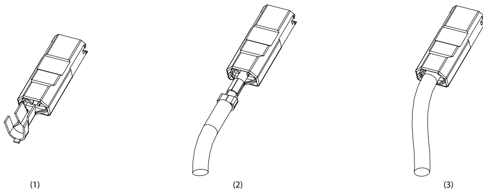
Рисунок 43: Подключение разъема для распределения нагрузки и тормоза
