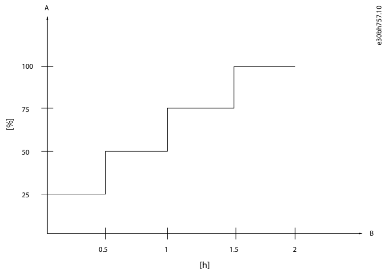
Рисунок 23: Процедура повторной формовки конденсаторов постоянного тока
