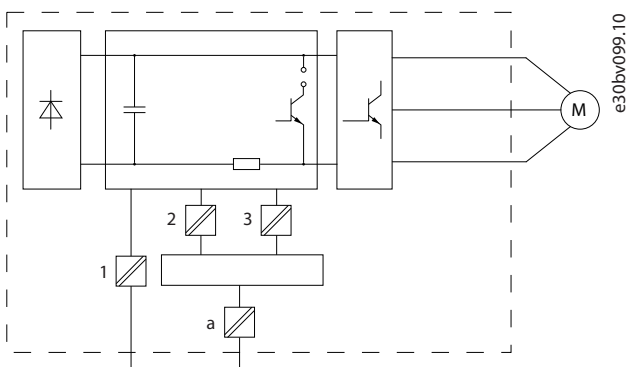
Рисунок 33: Гальваническая развязка
