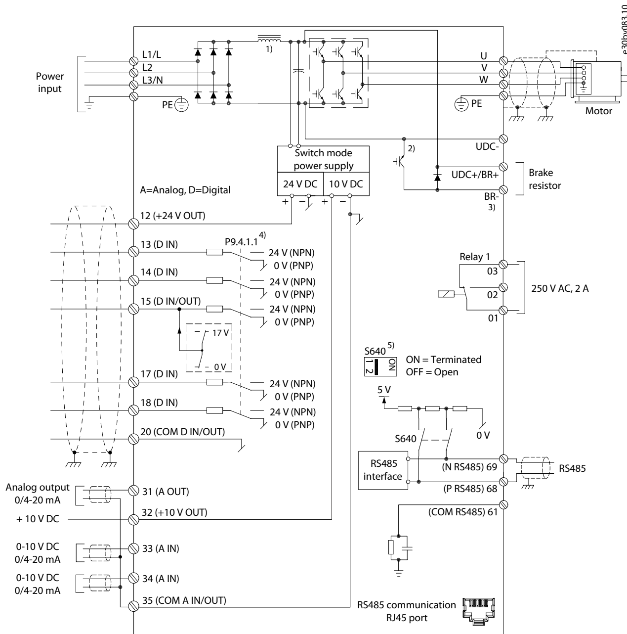
Рисунок 28: Схема соединений
