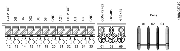
Рисунок 5: Обзор клемм управления
