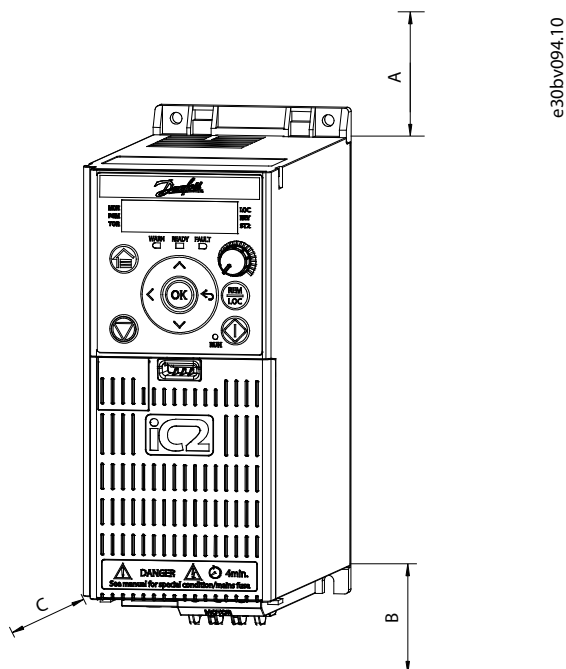
Рисунок 27: Рекомендуемый зазор для обеспечения доступа для обслуживания
