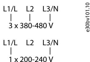
Рисунок 39: Однофазные и трехфазные проводные соединения
