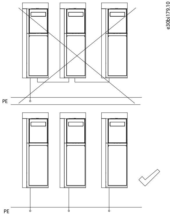
Рисунок 32: Принцип заземления
