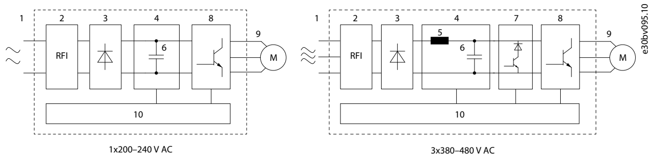
Рисунок 1: Блок-схема для изделий «iC2-Micro Frequency Converters»
