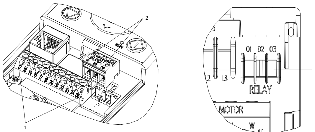
Рисунок 40: Номера и расположение клемм управления
