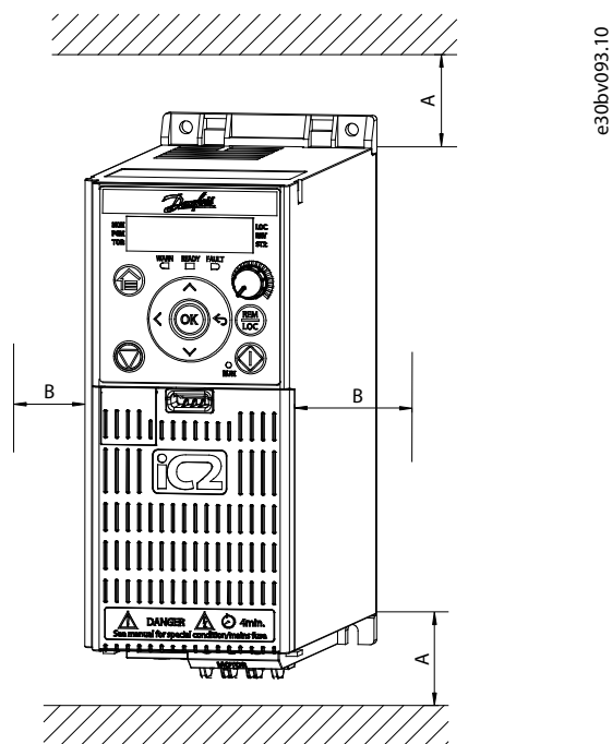
Рисунок 26: Минимальные зазоры для охлаждения
