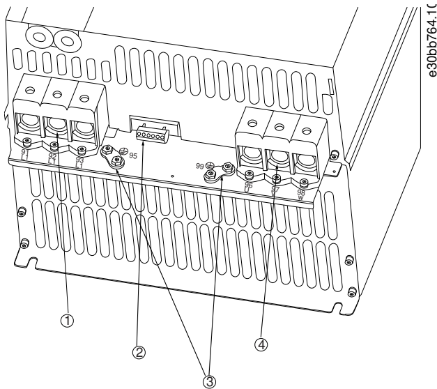
Илюстрация 7: Корпус с размер Н8, IP20, 380 – 480 V, 90 kW (125 к.с.), IP20, 200 – 240 V, 37 – 45 kW (50 – 60 к.с.), IP20, 525 – 600 V, 75 – 90 kW (100 – 125 к.с.)
