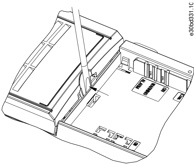
Илюстрация 23: Сваляне на клемния капак
