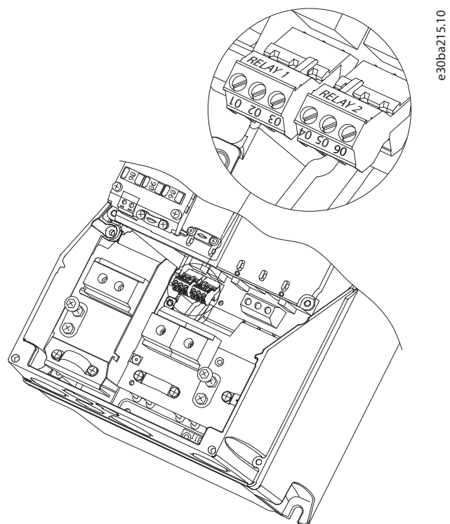
Obrázek 20: Relé na konstrukční velikosti I6, IP54, 380–480 V, 22–37 kW (30–50 hp)
