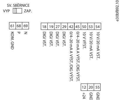
Obrázek 24: Řídicí svorky
