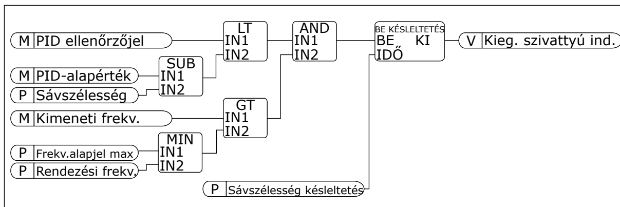
Ábra 101: Rendezési frekvencia
