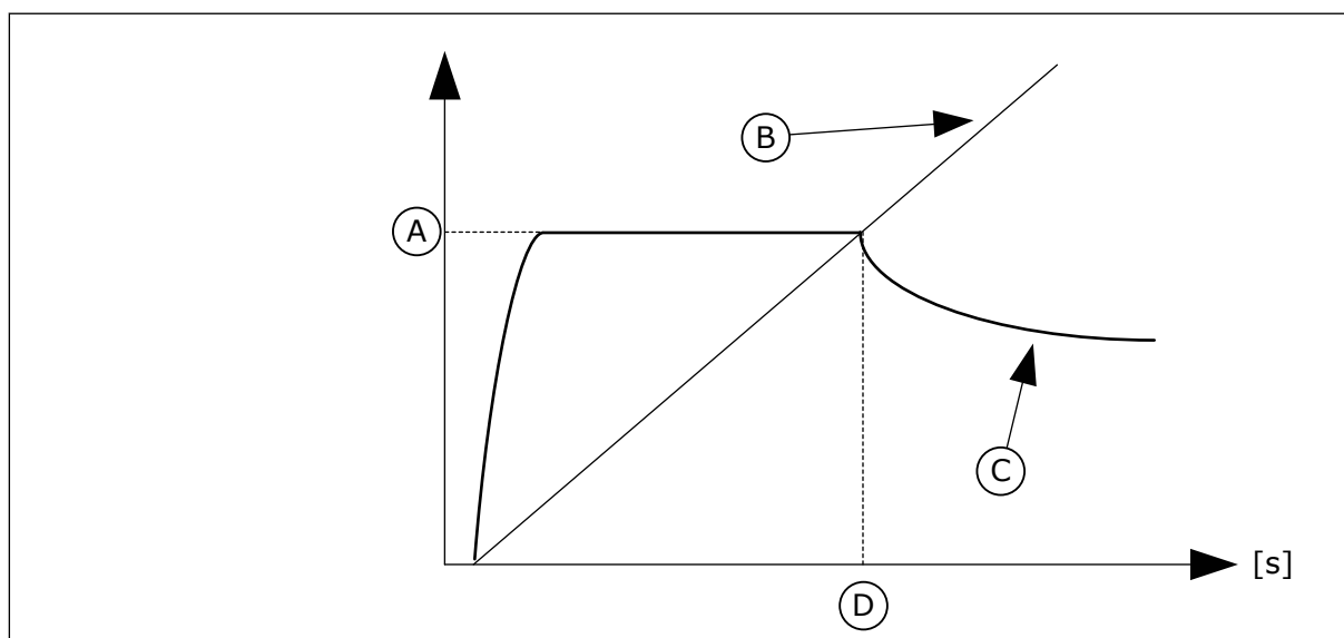
Ábra 40: Az I/f-indítás paraméterei
