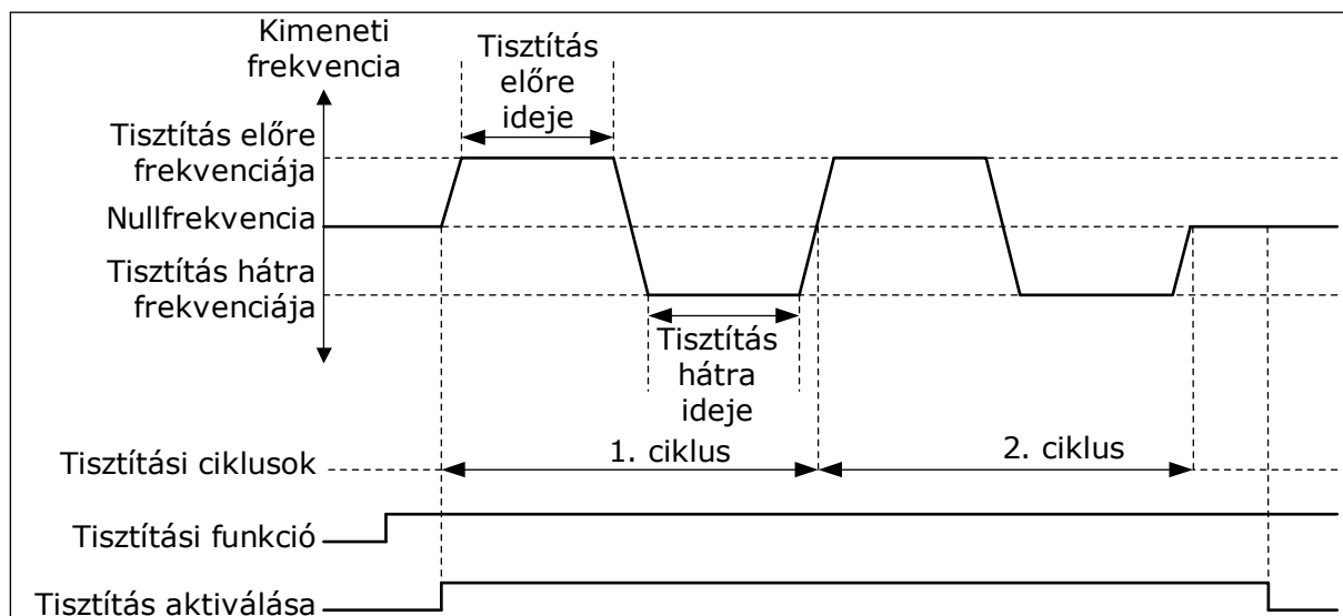
Ábra 104: Az Automatikus tisztítás funkció
