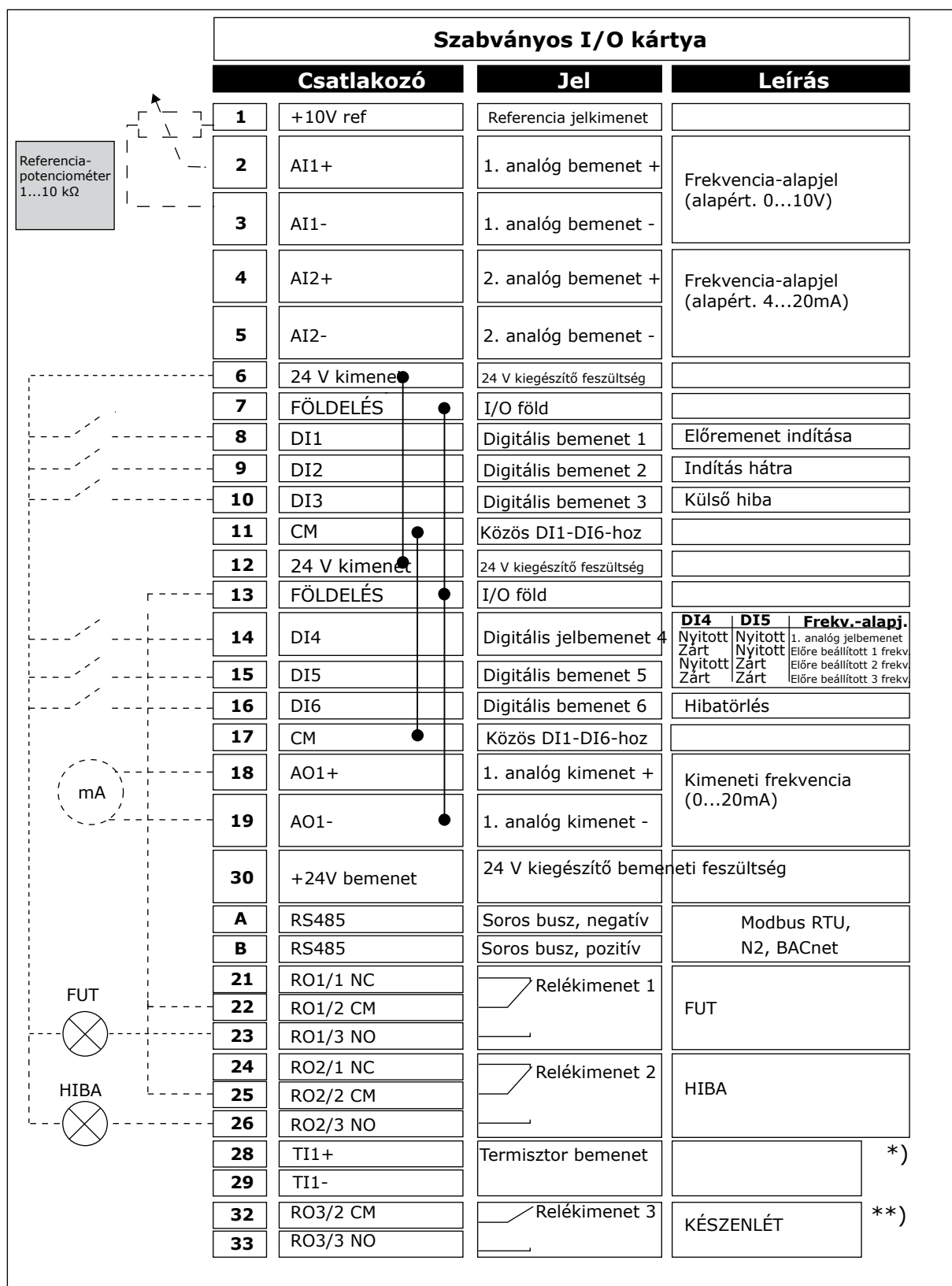
Ábra 4: A Szabványos és HVAC alkalmazások alapértelmezett vezérlőcsatlakozásai
