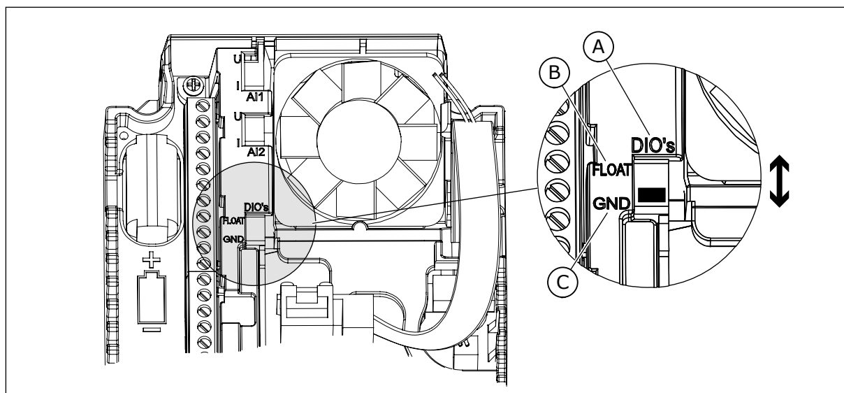
Ábra 97: Elkülönítő DIP-kapcsoló
