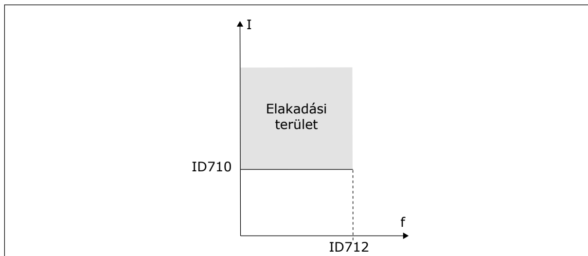
Ábra 68: Elakadási beállítások
