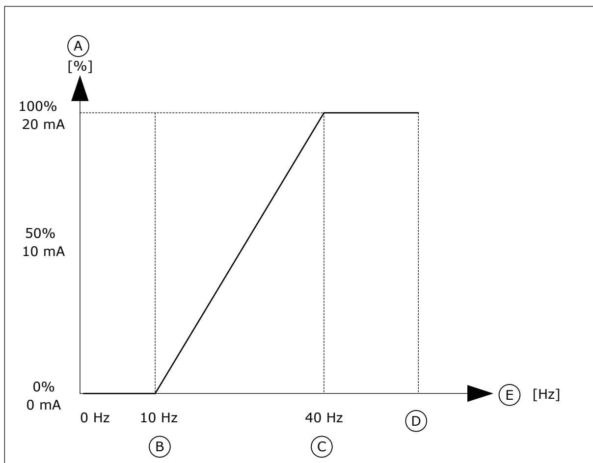
Ábra 62: Az A01 jel skálázása
