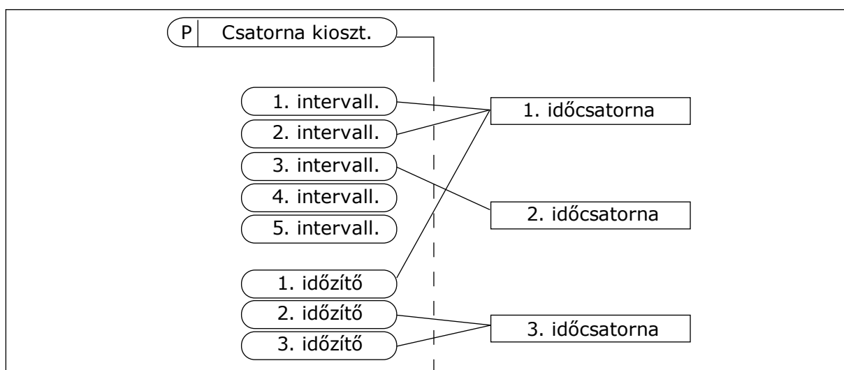
Ábra 73: Az időcsatornához rugalmasan lehet intervallumokat vagy időzítőket rendelni. Minden intervallum vagy időzítő rendelkezik egy paraméterrel, mellyel hozzárendelheti őket egy időcsatornához.
