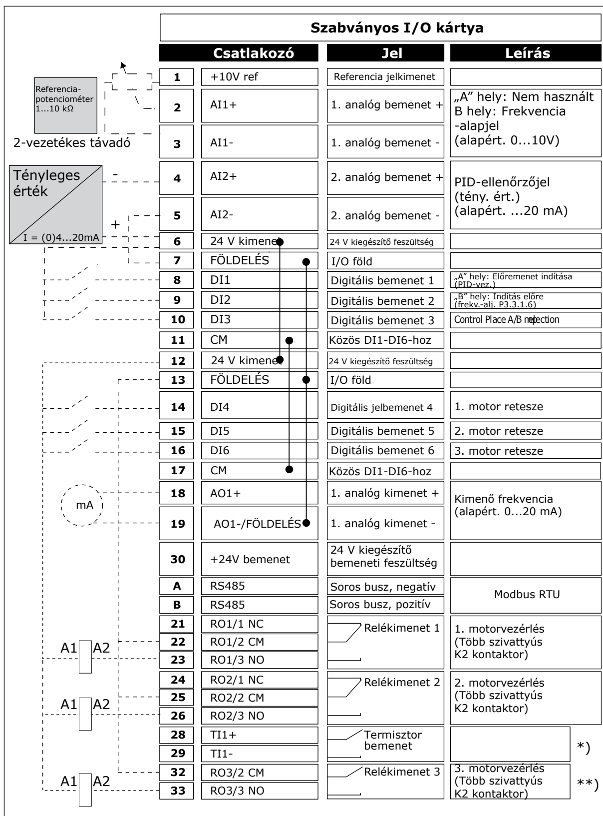
Ábra 11: A Többszivattyús (egy frekvenciaváltós) alkalmazás alapértelmezett vezérlőcsatlakozásai
