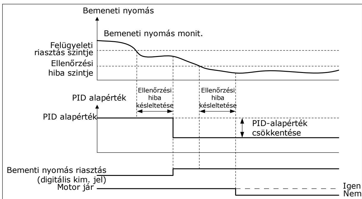
Ábra 87: A Bemeneti nyomás felügyelete funkció
