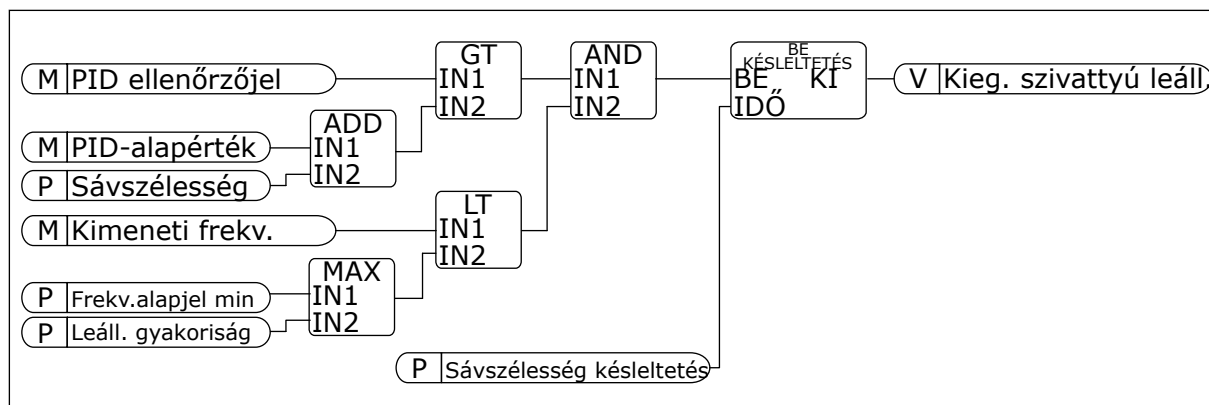
Ábra 102: Visszarendezési frekvencia
