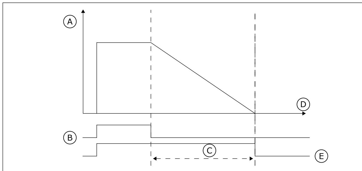
Ábra 74: Az aktiválási jel egy digitális bemenetből vagy egy virtuális digitális bemenetből, például időcsatornából érkezik. Az időzítő az eső élről kezdve lefelé számol.
