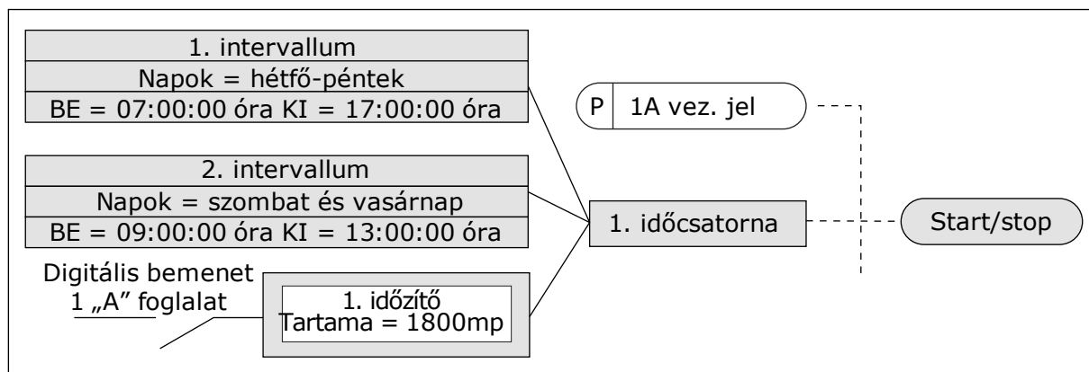
Ábra 78: Digitális bemenet helyett az 1. időcsatorna szolgál az indítási parancs vezérlési jeleként
