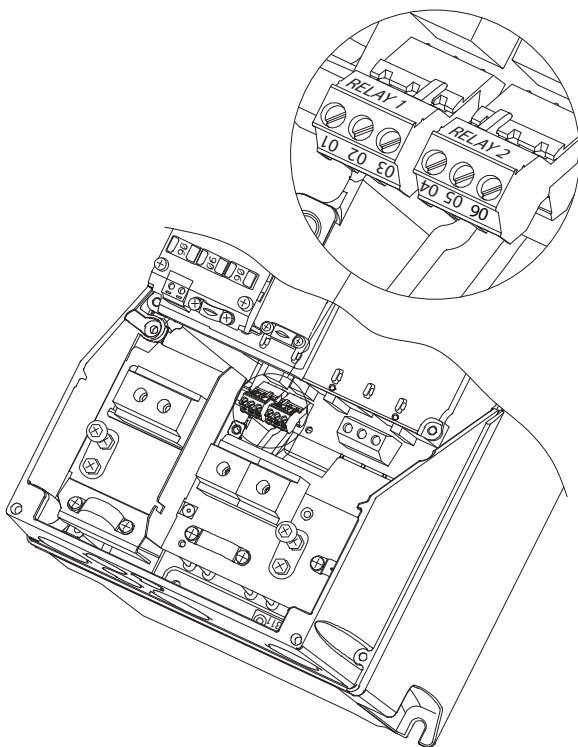
Illustration 20: Relæer på kapslingsstørrelse I6, IP54, 380–480 V, 22–37 kW (30–50 hk)
