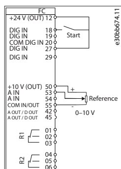
Illustration 27: Frekvensomformerens ledningsføring
