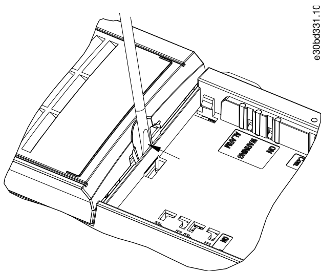
Illustration 23: Afmontering af klemmeafdækning
