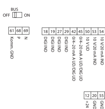
Illustration 24: Styreklemmer
