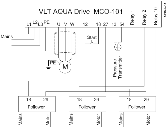
圖 8.2: 電氣配線。在主變頻器上的端子 27 可作為脈衝輸出的設定值。在從變頻器上的端子 29 可作為脈衝輸入設定值。所有的從變頻器與主電源連接的方式與標注為主電源與馬達的主變頻器連接方式相同。
