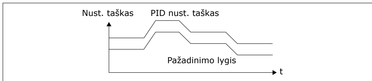
Pav. 82: Pažadinimo režimas: sant. nust. taškas
