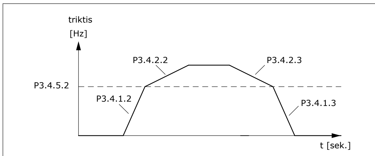
Pav. 50: 2 kreivės suaktyvinimas, kai išeinančios srovės dažnis viršija ribinę vertę. (P3.4.5.2 = kreivės ribinis dažn., P3.4.1.2 = 1 greit. trukmė, P3.4.2.2 = 2 greit. trukmė, P3.4.1.3 = 1 lėt. trukmė, P3.4.2.3 = 2 lėt. trukmė)
