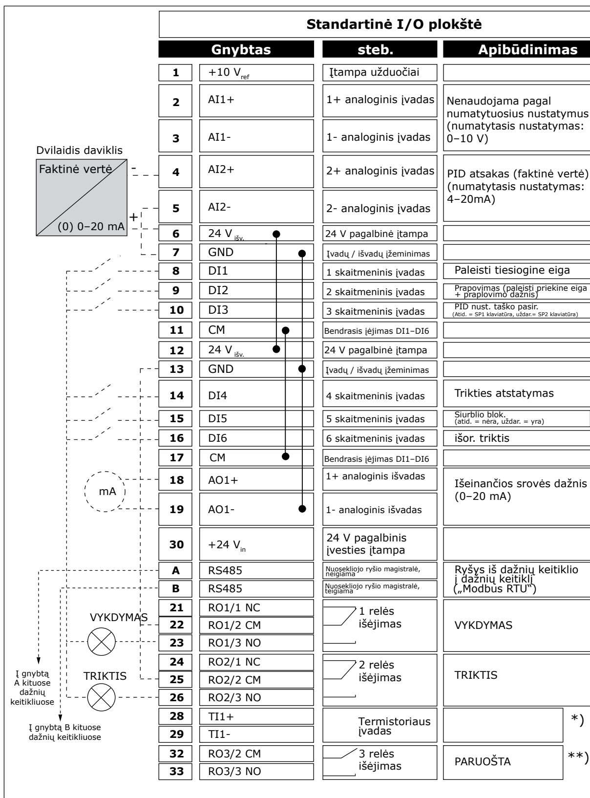
Pav. 16: Numatytosios kelių siurblių (kelių inverterių) programos valdymo jungtys
