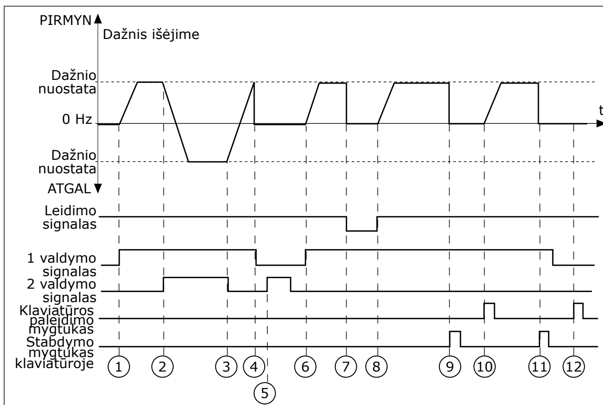
Pav. 45: Įvadų / išvadų A paleidimo / sustabdymo logika = 3
