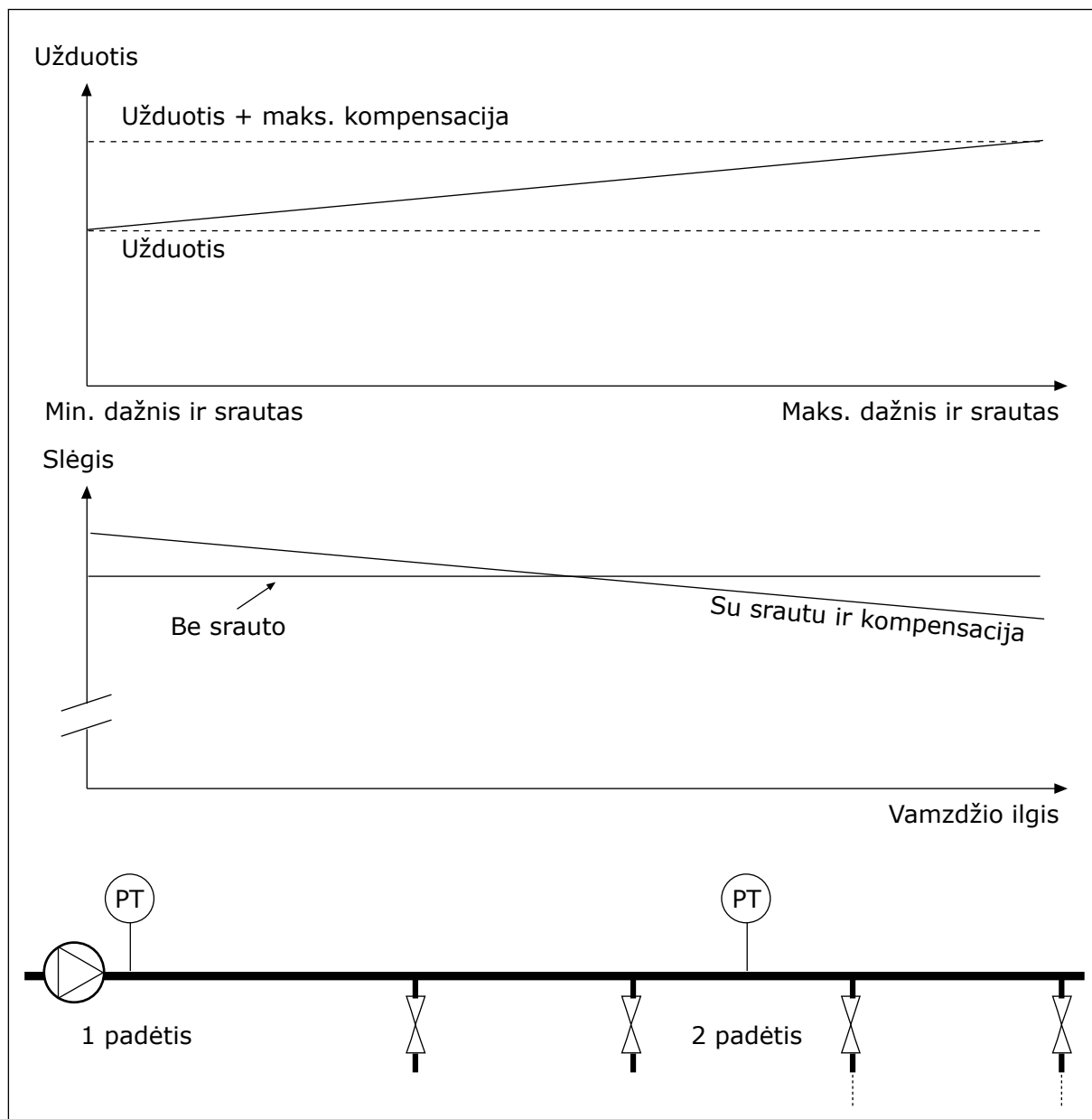
Pav. 85: Įjungti 1 užduotį slėgio nuostoliui kompensuoti
