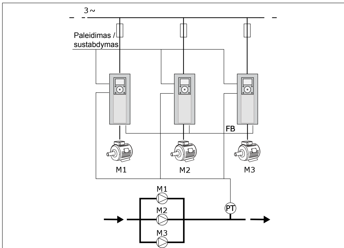
Pav. 13: Kelių siurblių (kelių inverterių) konfigūracija
