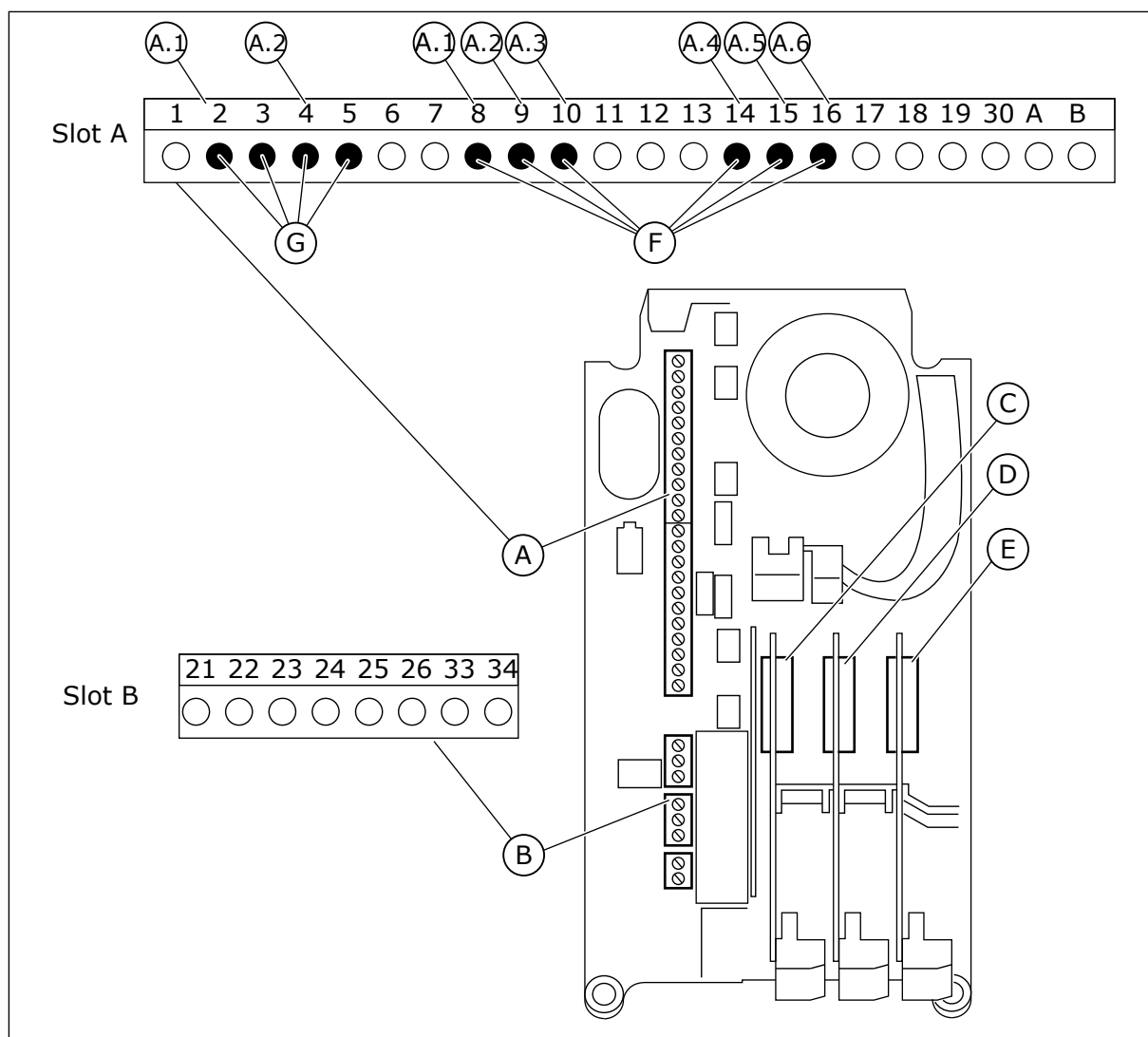
Pav. 51: Pasirenkamųjų plokščių lizdai ir programuojami įvadai
