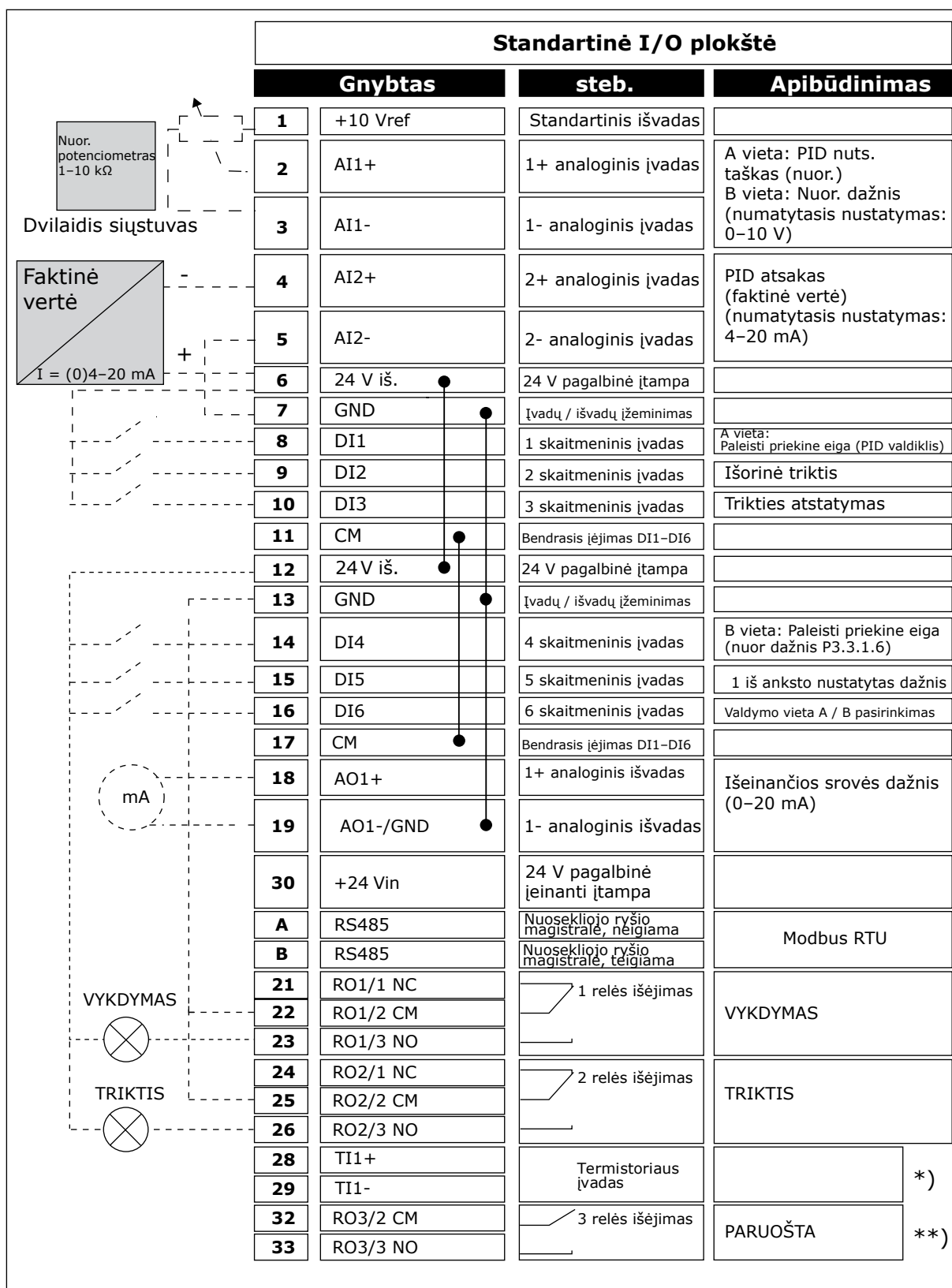
Pav. 6: PID valdymo programos numatytosios valdymo jungtys
