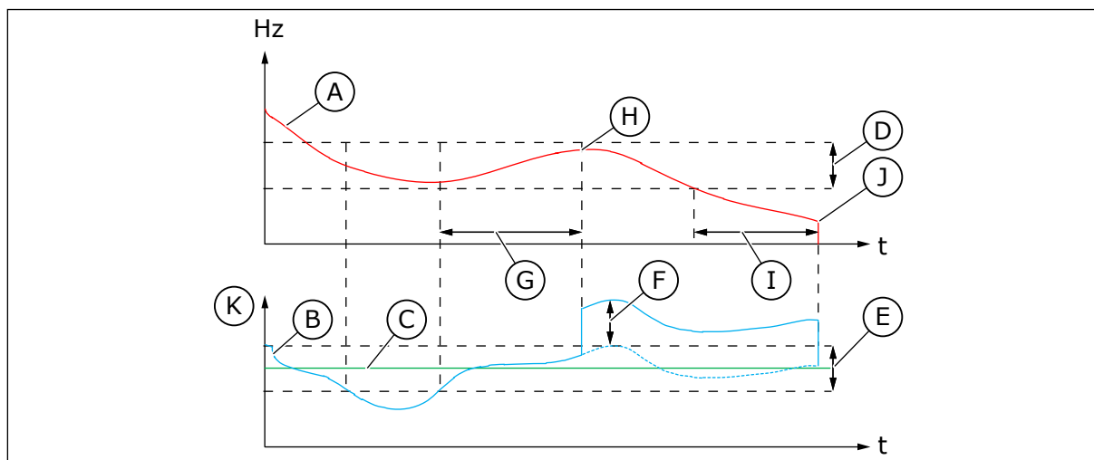
Pav. 88: Miego rež., nenust. joks poreikis
