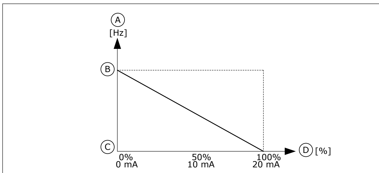
Pav. 61: AI1 signalo inversija, 1 pasirinkimas
