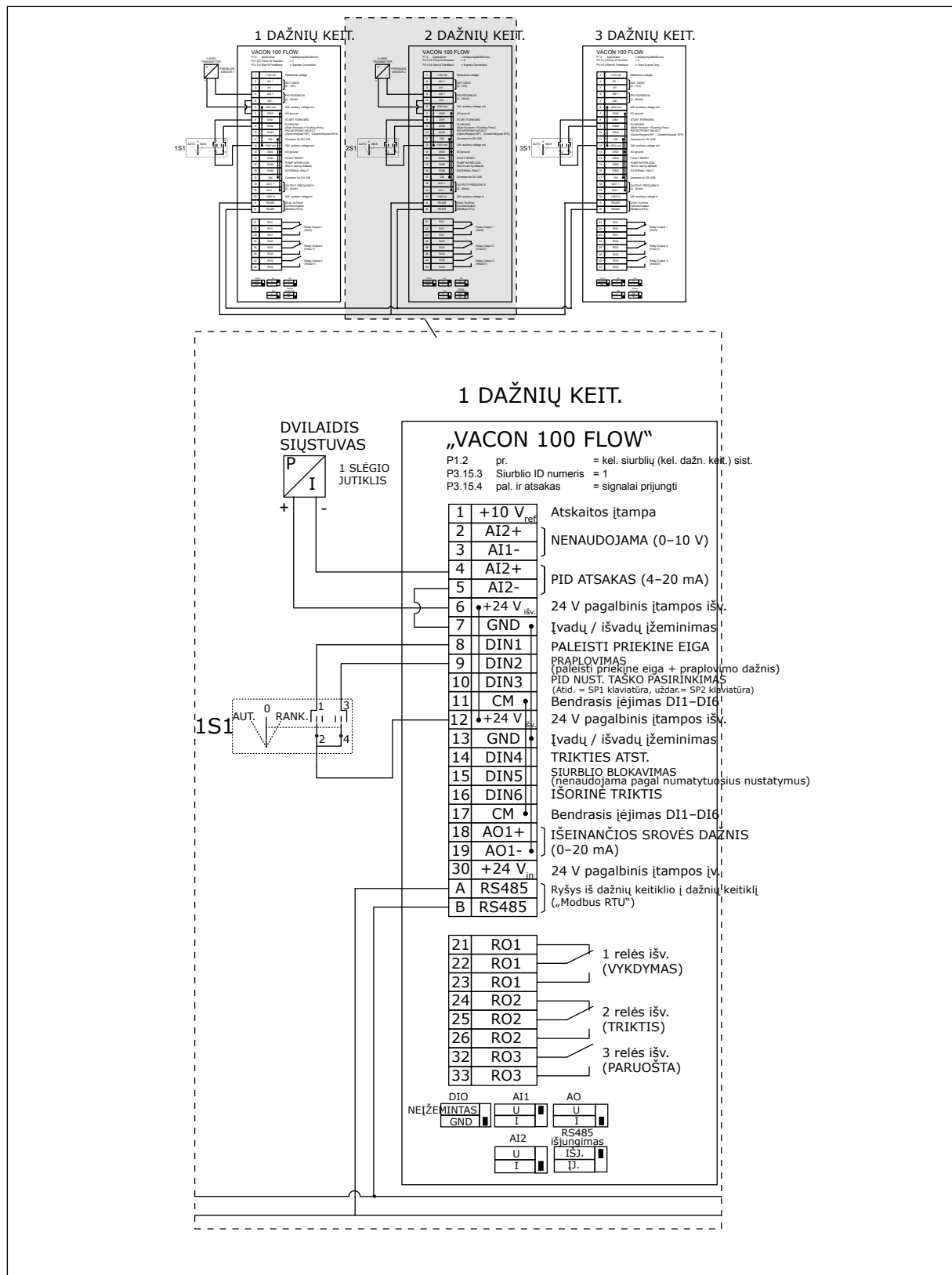
Pav. 25: Kelių siurbių (kelių inverterių) sistemos elektros kabelių schema, 3B pavyzdys
