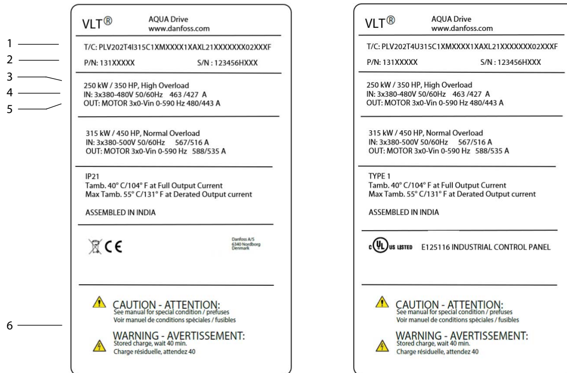
Ілюстрація 12: Приклад паспортної таблички виробу для корпусу Е6н (версія IEC ліворуч, версія UL праворуч)
