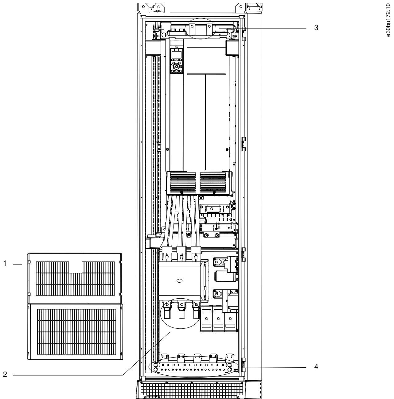
Ілюстрація 48: Точки підключення джерела живлення до вхідної силової опції (привод шафного типу, налаштований без шафа додаткового силового пристрою)
