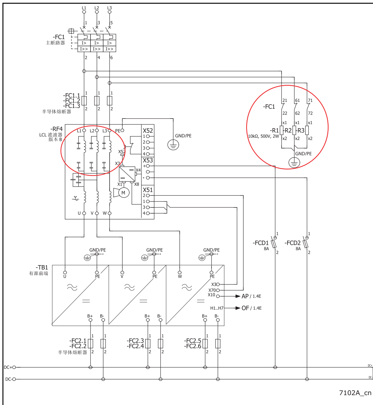
图 16. 以下情况下 LCL 和 AFE 电路的接线图：安装环境中具有接地故障保护继电器； 安装环境为 IT 网络；或者有其他制造商的 AFE 连接到同一变压器二次侧
