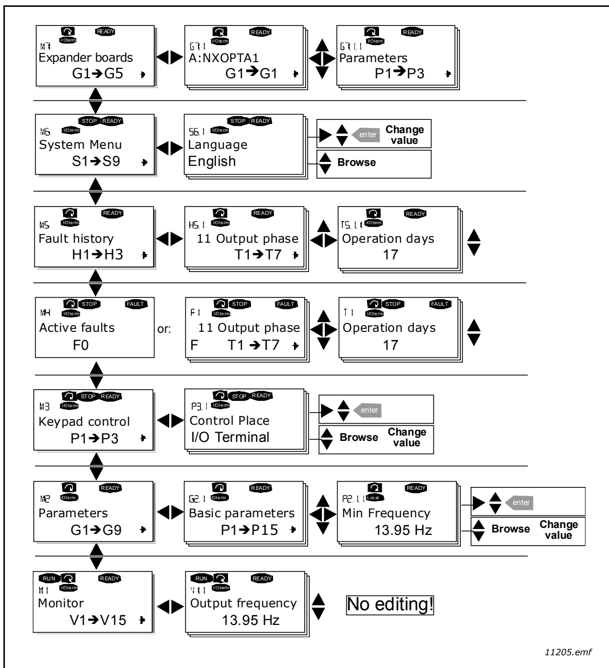
图 58. 键盘导航图
