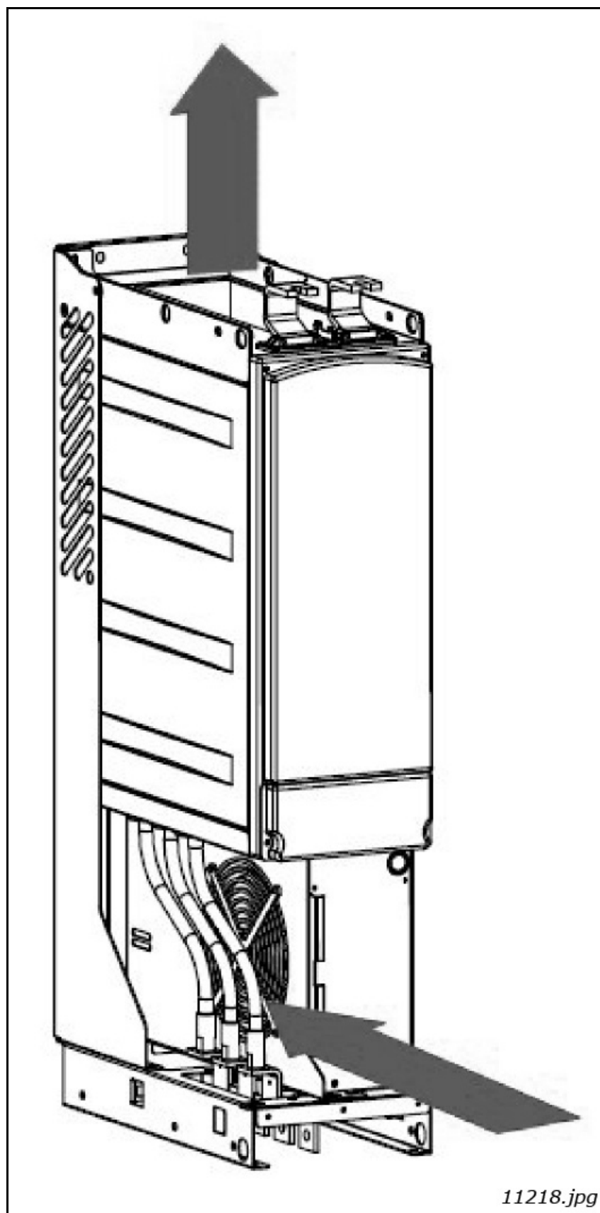
图 31. FI9 和 FI10 单元的冷却气流
