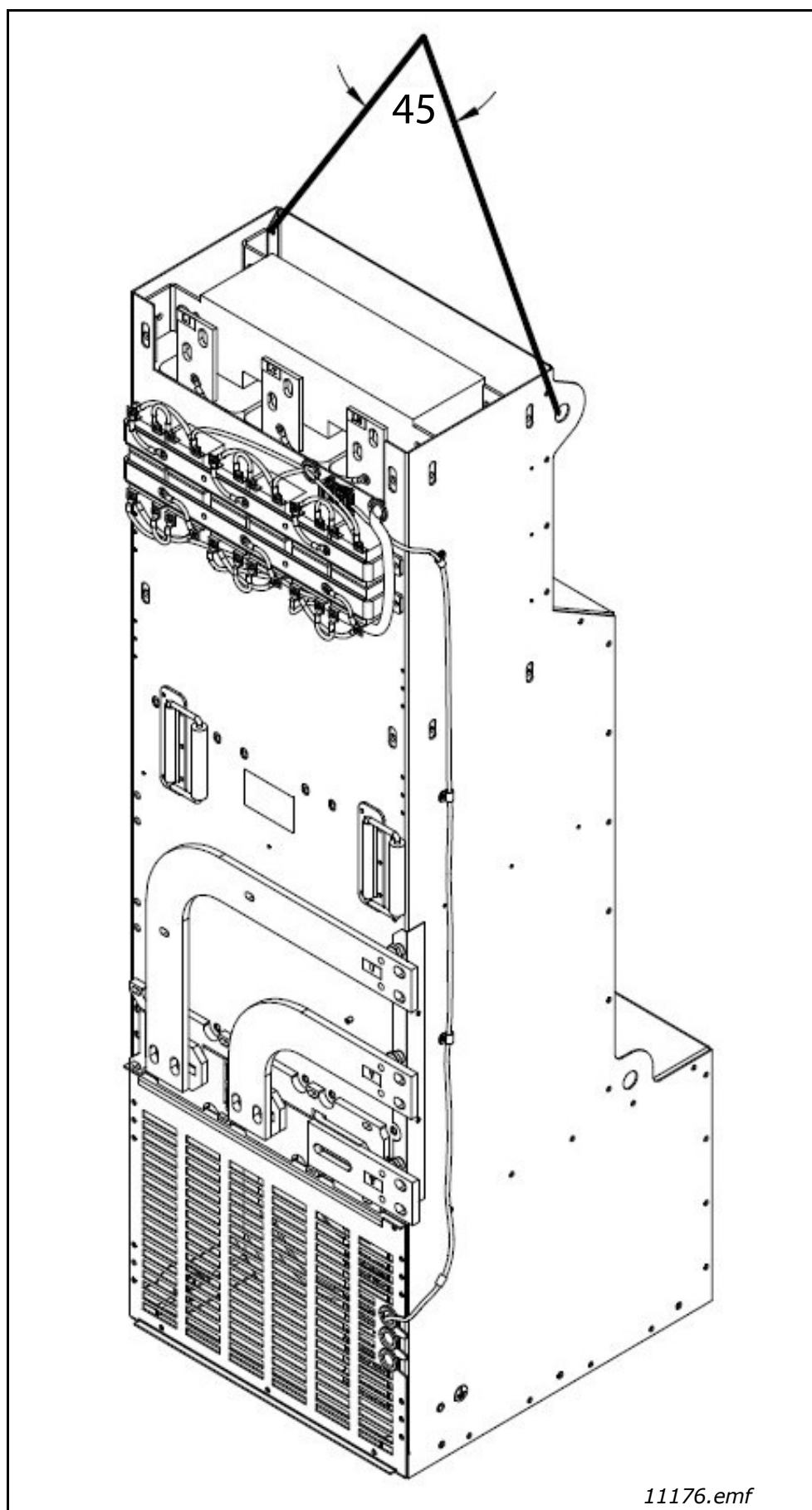
图 4. FI13 LCL 滤波器的提升点
