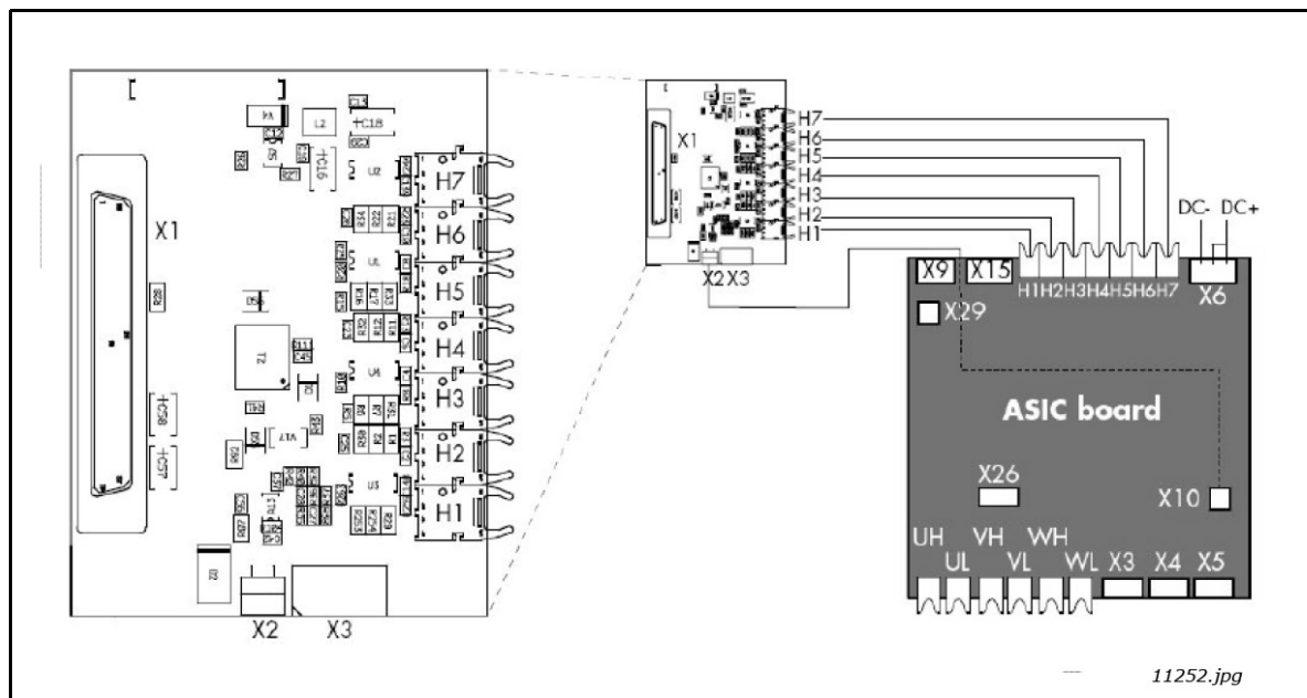
图 11. 光缆适配板
