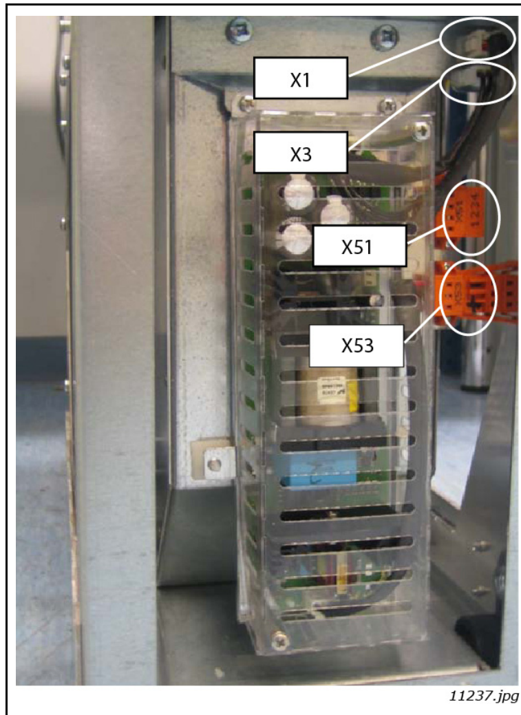
图 41. FI9 和 FI10 LCL 滤波器中的集成直流 / 直流电源
