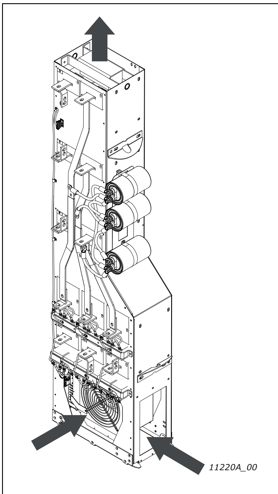
图 34. FI9 和 FI10 LCL 滤波器的冷却气流
