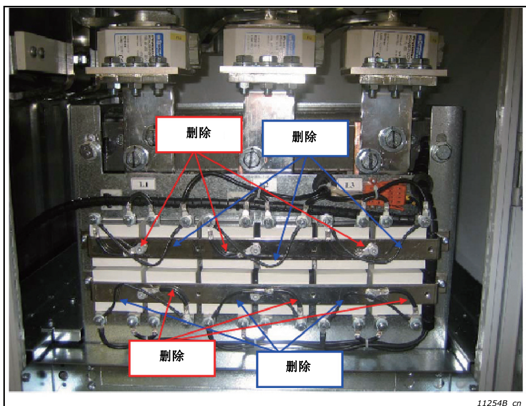
图 18. FI13 LCL 滤波器中的 HF 电容器
