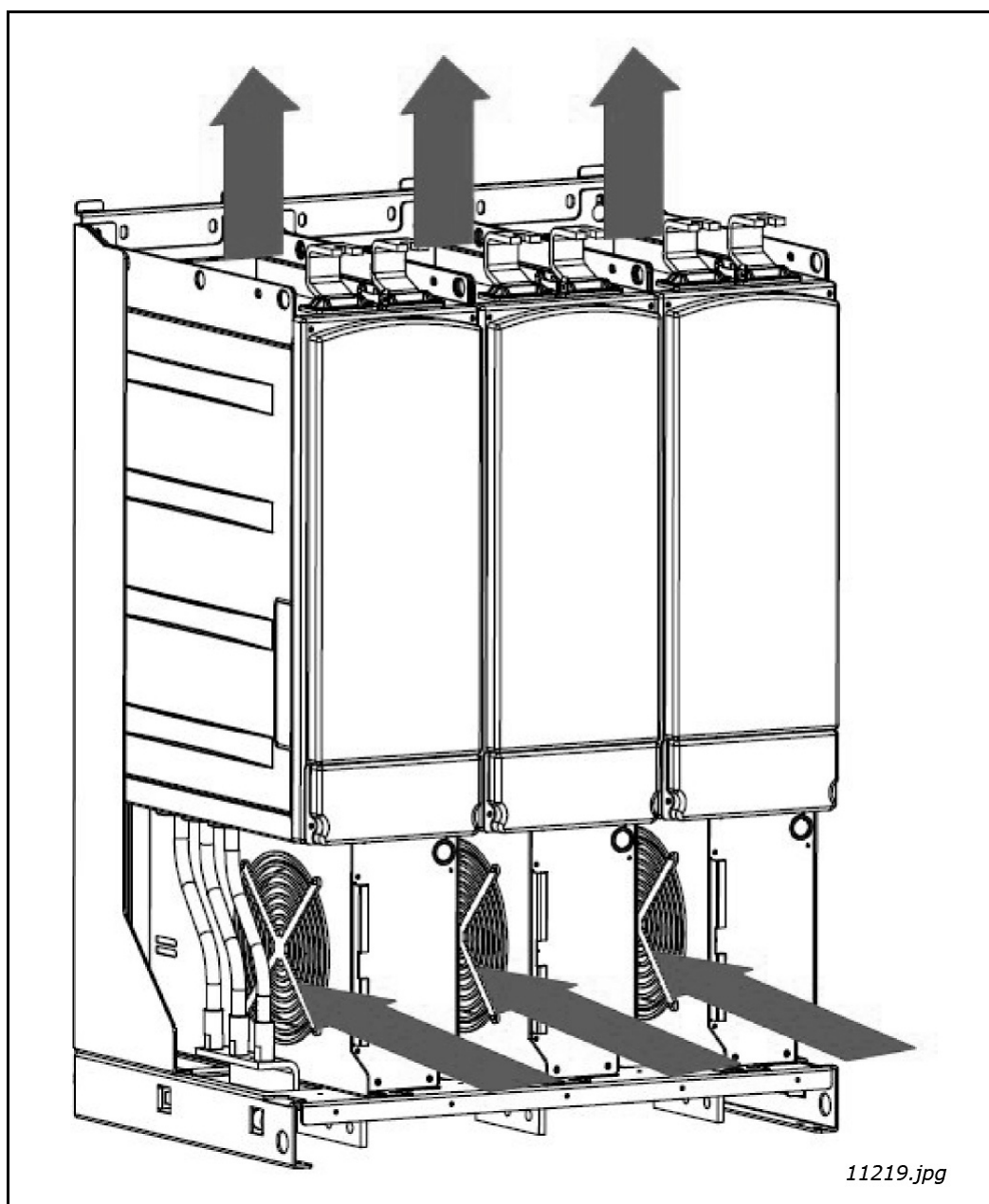
图 32. FI13 单元的冷却气流
