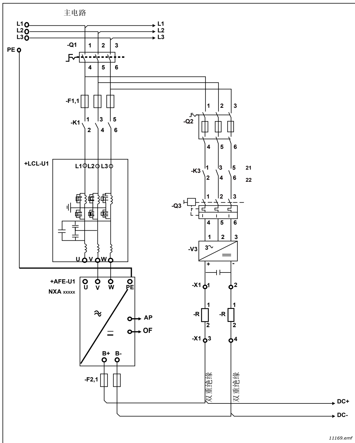
图 6. VACON® 有源前端单一单元连接
