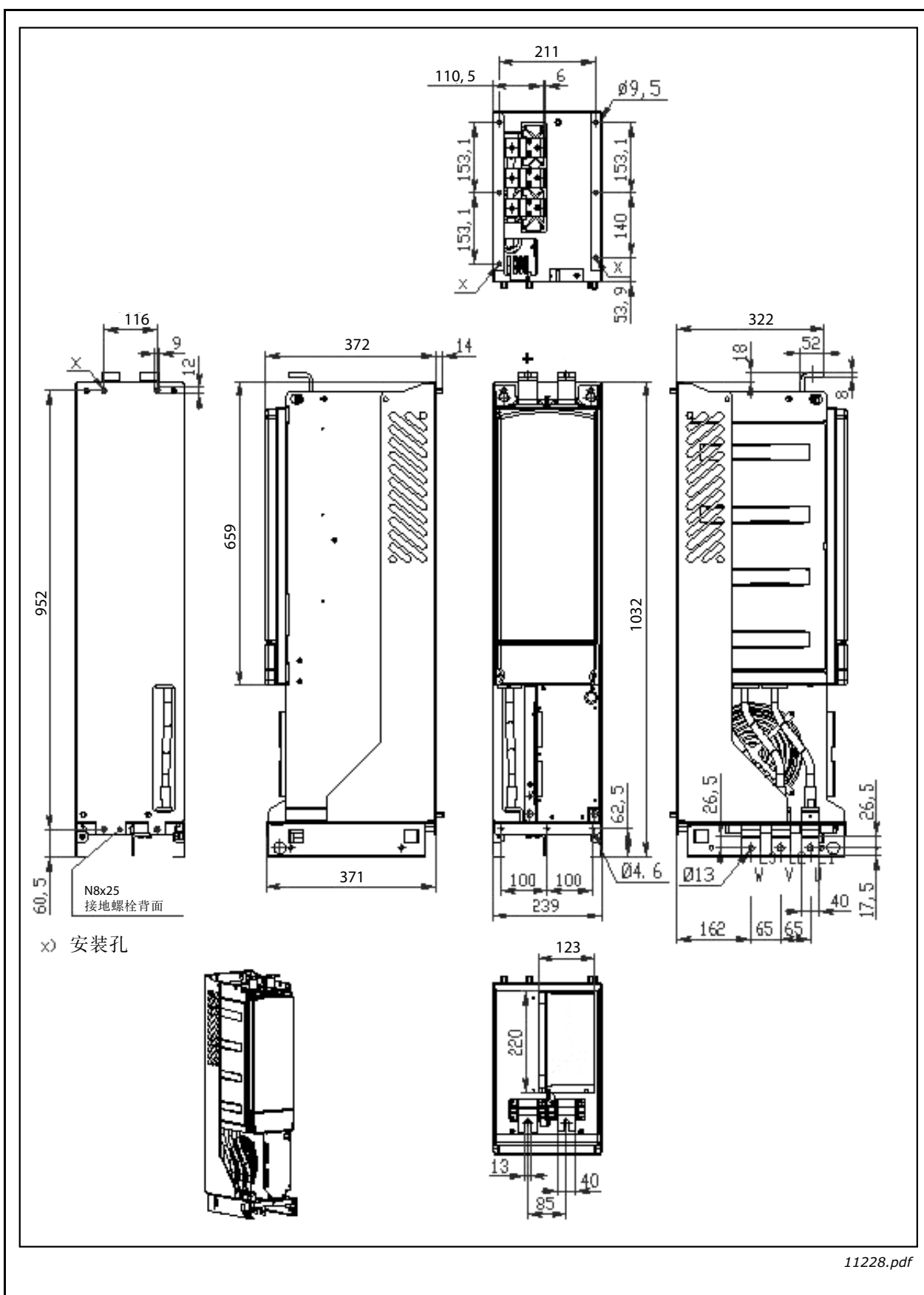
图 77. F19 尺寸
