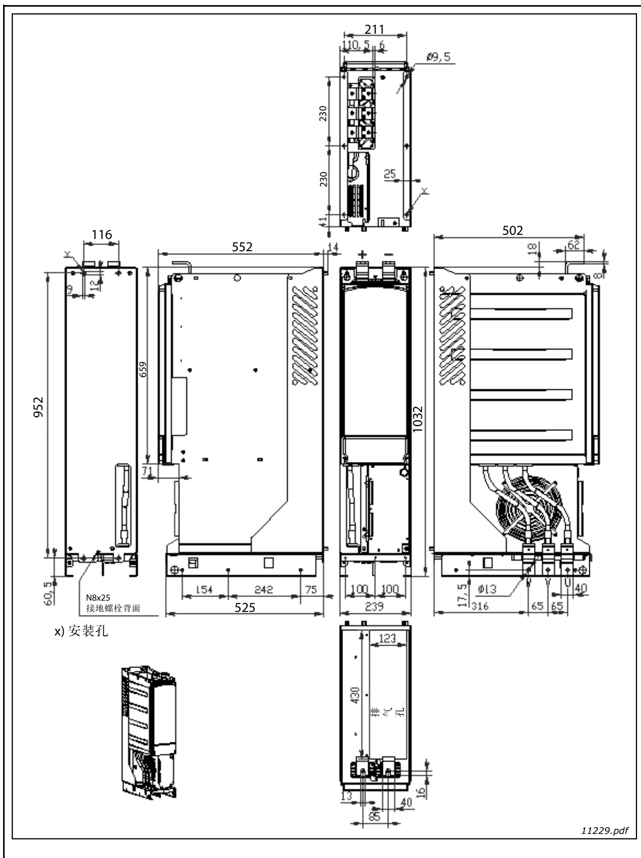
图 78. F110 尺寸
