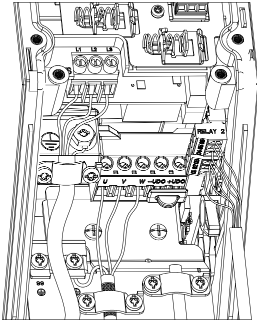
Kuva 17: IP54-kokoluokat I2, I3, I4
