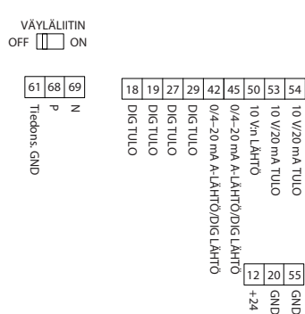
Kuva 24: Ohjausliittimet
