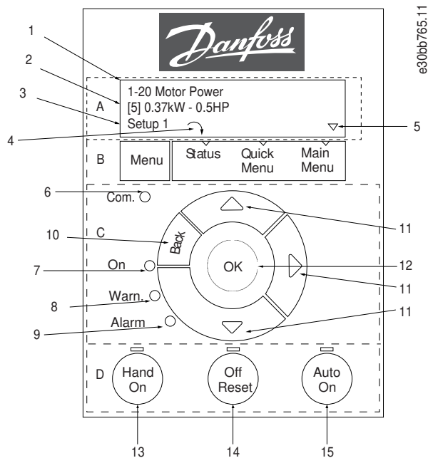
Kuva 26: Paikallishjauspaneeli (LCP)
