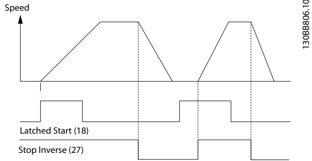
Bild 6.3 Pulsstart/pulsstopp, inverterat
