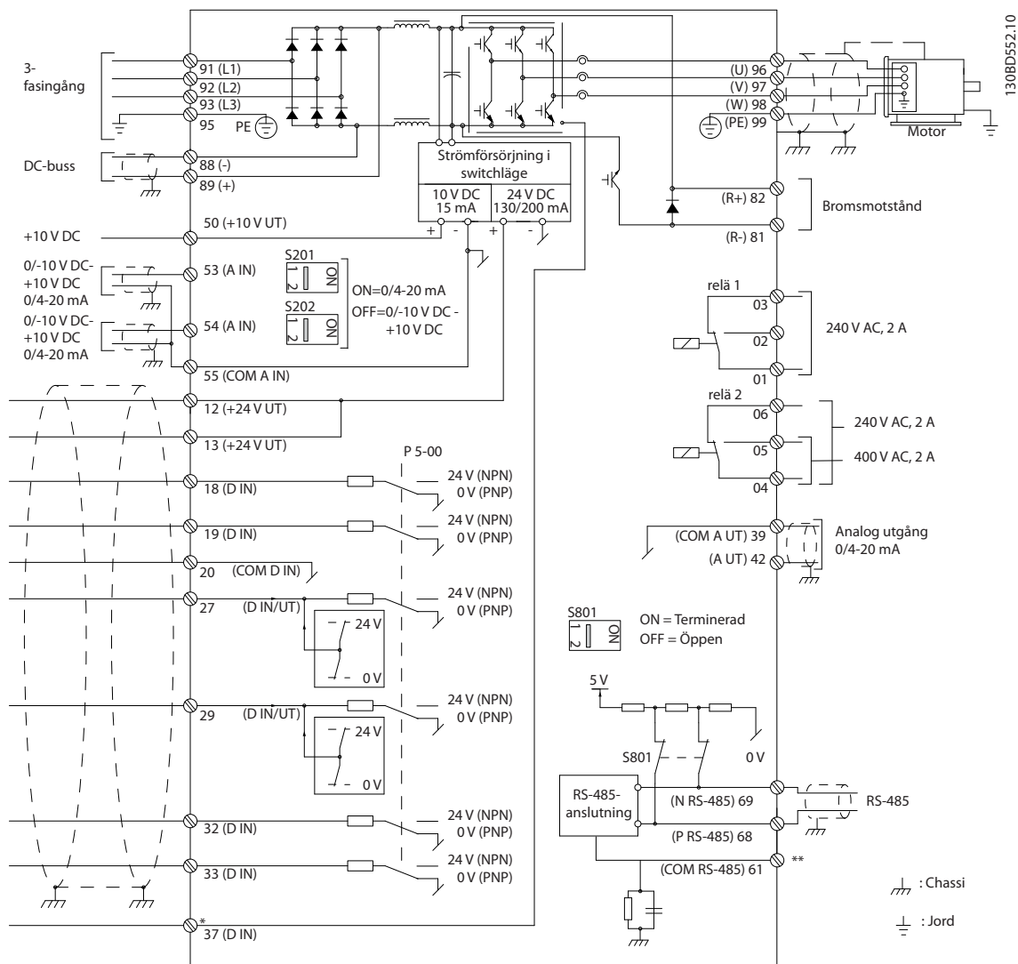
Bild 4.1 Grundläggande kopplingsschema
