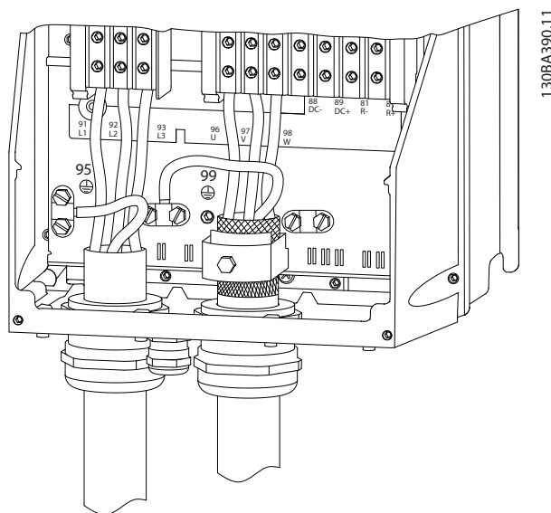
Bild 4.8 Dragning av motor-, nät- och jordningskablar för B- och C-kapslingar, med skärmad kabel
